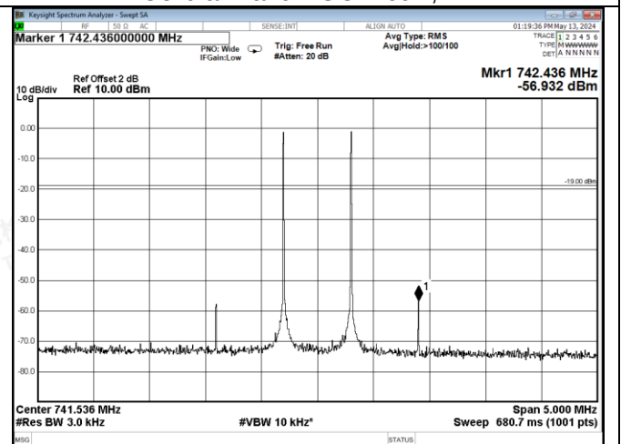
Lower 700MHz band AGC+10dB, DL
