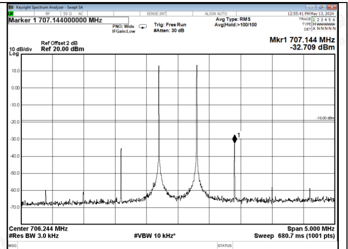
Lower 700MHz band AGC+10dB, UL
