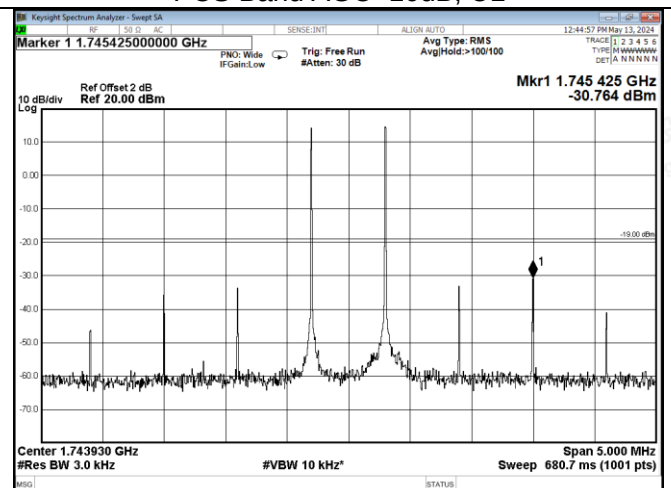
AWS Band AGC+10dB, UL
