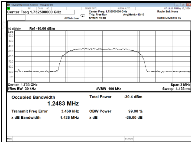
CDMA-AWS band UL input
