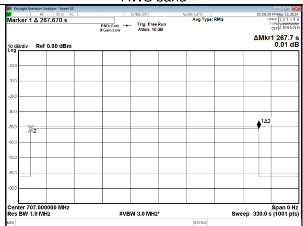
Lower 700MHz band
