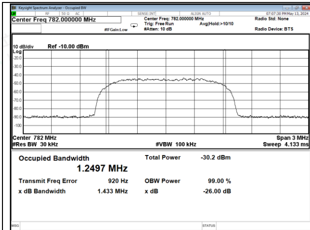
CDMA-Upper 700 band UL input
