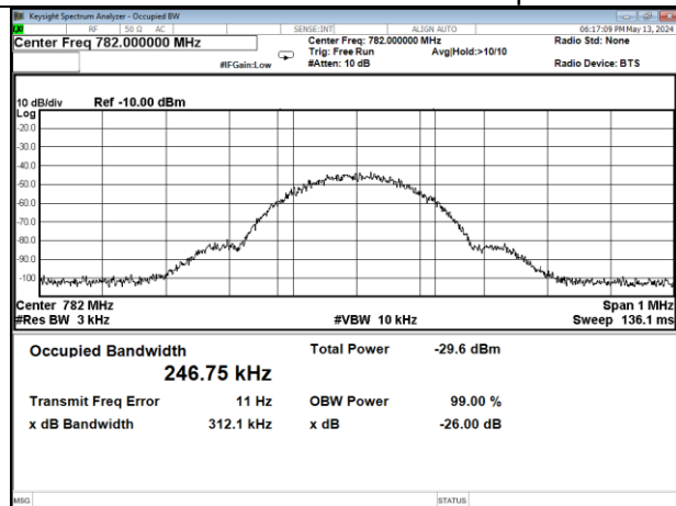
GSM-Upper 700MHz band UL input
