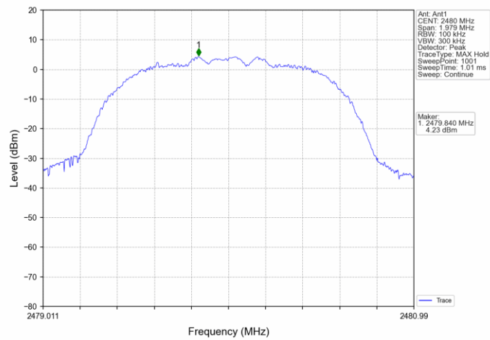
Pi/4DQPSK 2DH5_HOPP Ant1 NTNv
