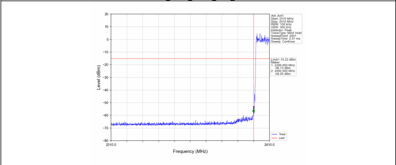
8DPSK_3DH5_HOPP_Ant1_NTNV
