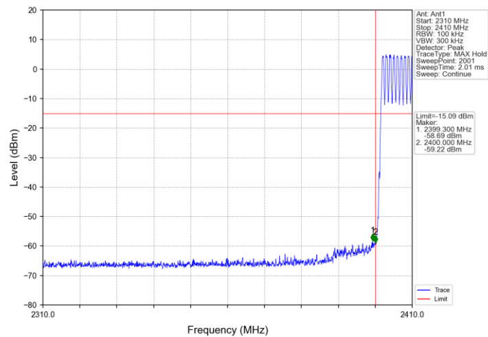
GFSK DH5_HOPP_Ant1_NTNV
