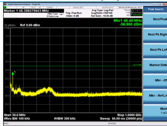
30-1000 MHz (Mid)
