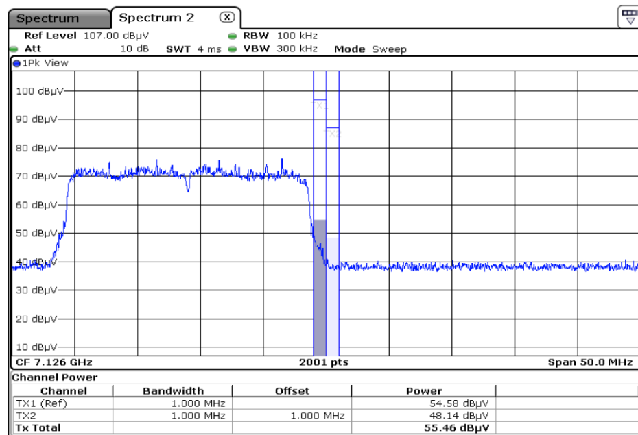
2 Band Edge
