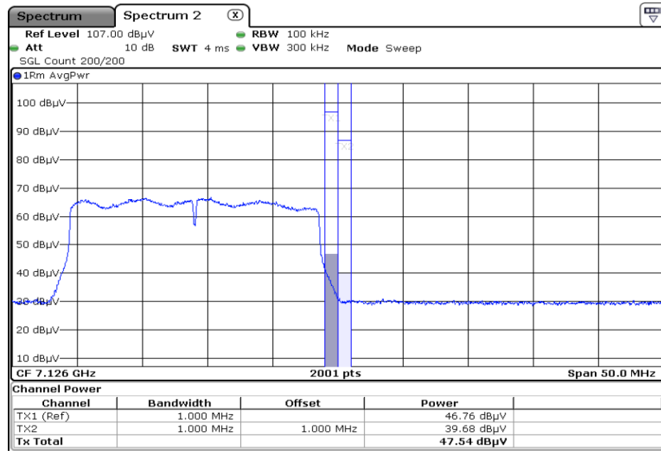
1 Band Edge
