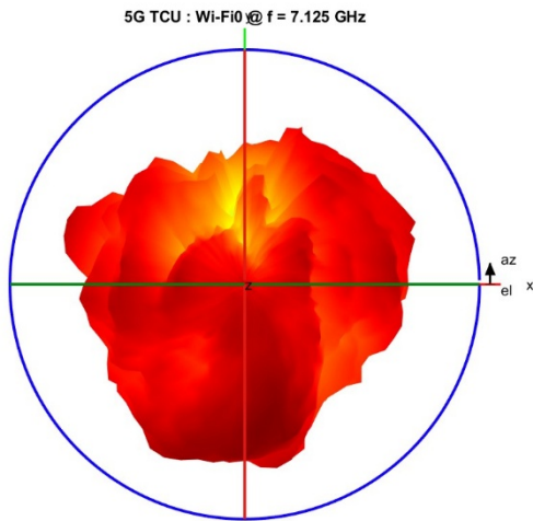
Wi-Fi0
