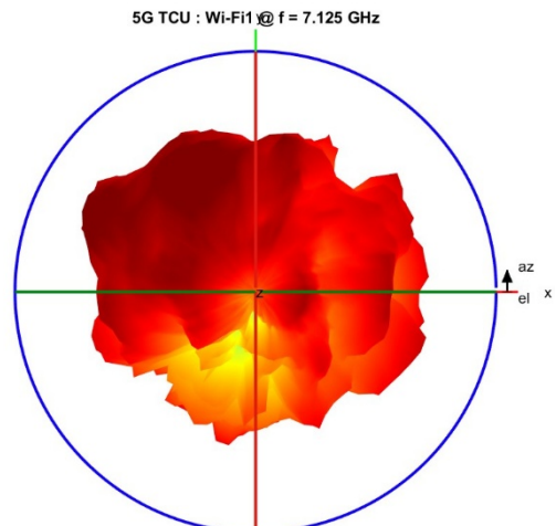
Wi-Fi1
