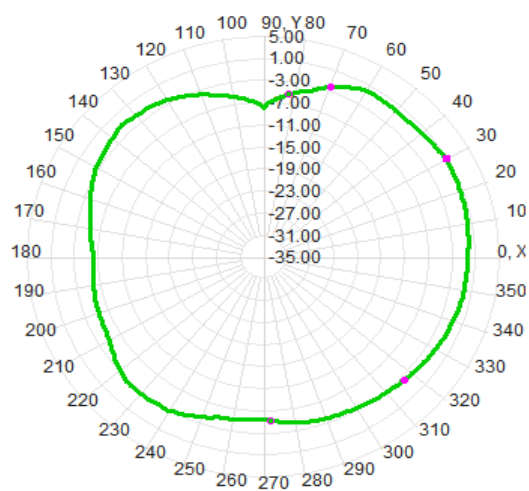
5G theta=90deg
