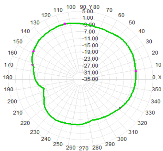
2.4G theta=90deg
