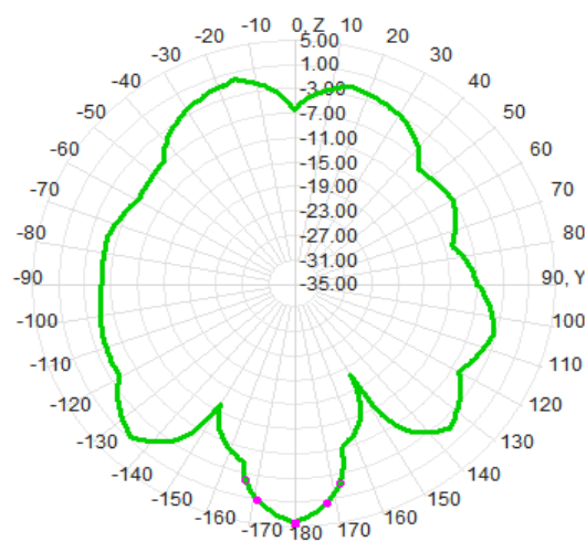
5G phi=90deg
