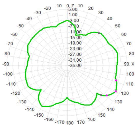
5G phi=0deg
