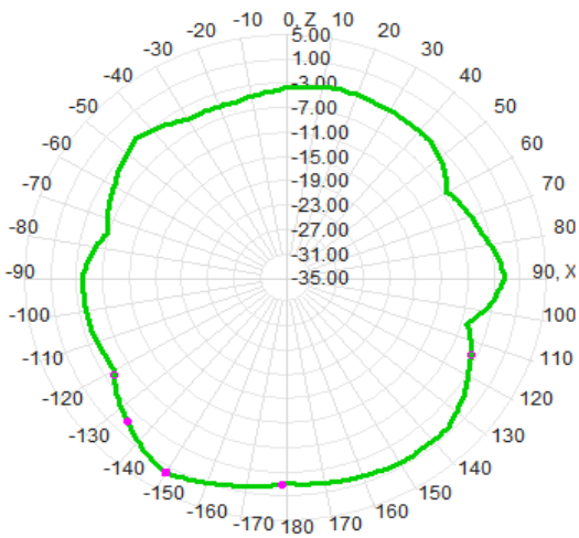
2.4G phi=0deg
