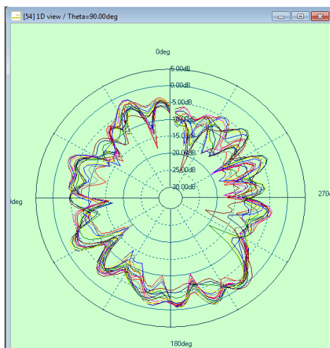
5G phi=0deg
