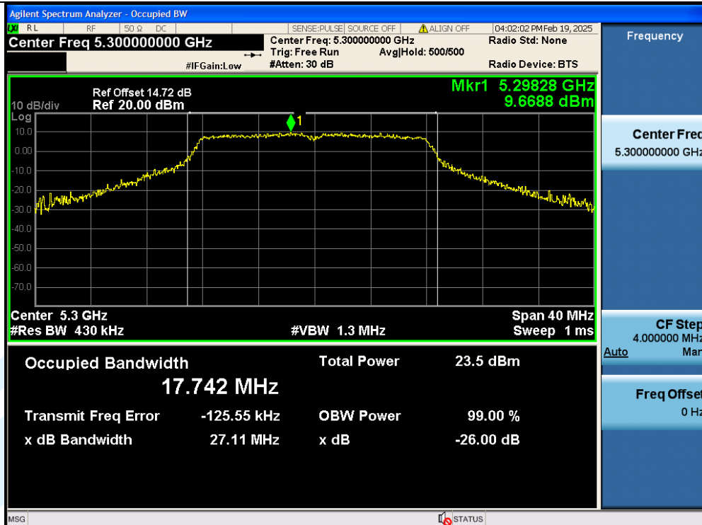
11A-Ant1-5300
