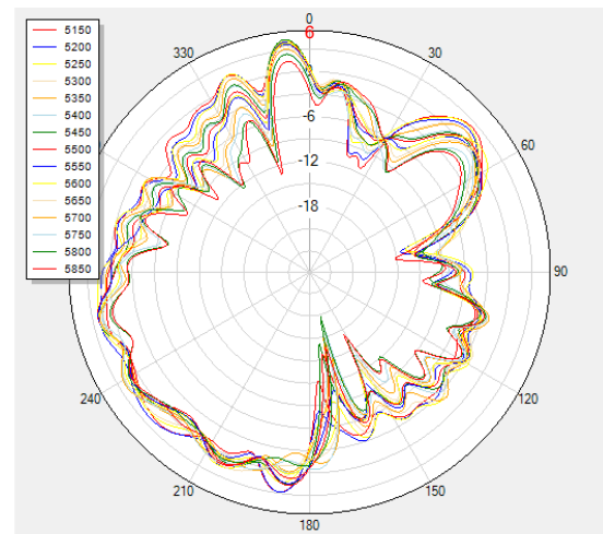
5G phi=90deg
