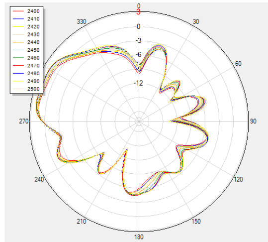
2. 4G theta=90deg
