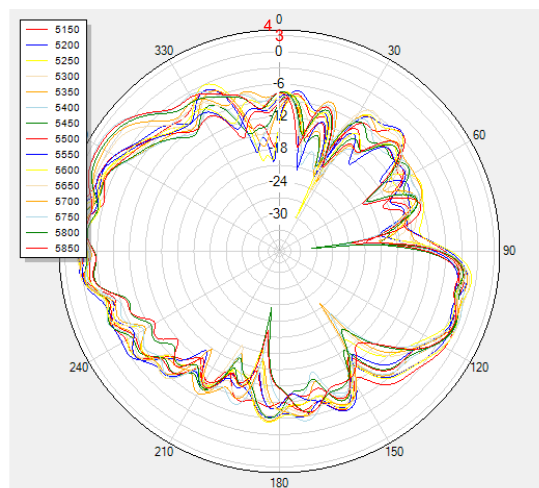
5G theta=90deg
