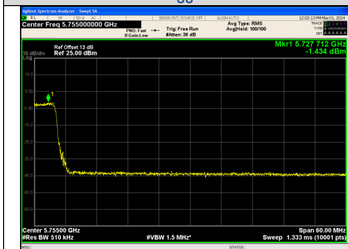
IEEE 802.11ax_Channel 142_40MHz_Antenna 0_RU&amp;Index SU
