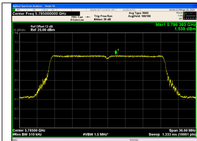
IEEE 802.11ax_Channel 157_20MHz_Antenna 0_RU&amp;Index SU
