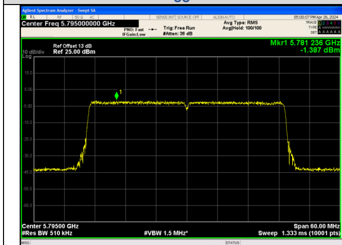
IEEE 802.11ax_Channel 159_40MHz_Antenna 0_RU&amp;Index SU
