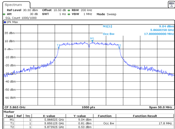
802.11ac20_5865MHz_Chain 0
