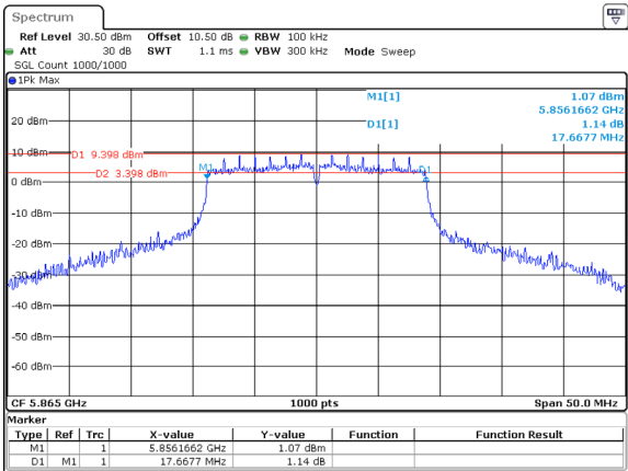
802.11ac20_5865MHz_Chain 0
