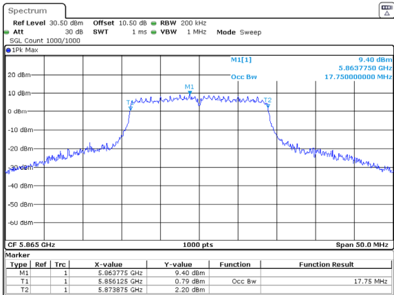
802.11ac20_5865MHz_Chain 1
