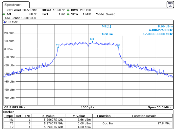
802.11ac20_5885MHz_Chain 0
