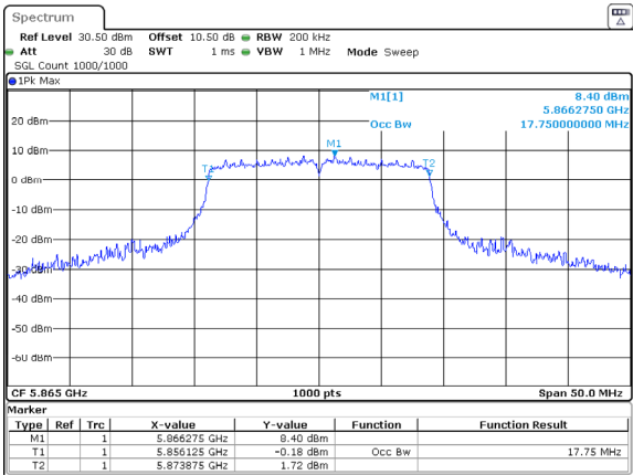
802.11ac20_5865MHz_Chain 2
