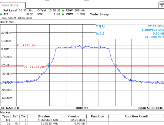
802.11ac20_5580MHz_Chain 0 21.864MHz
