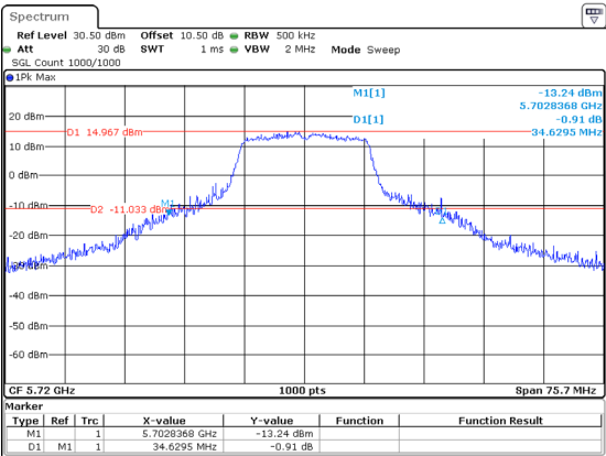
802.11a_5720MHz_Chain 1 34.630MHz
