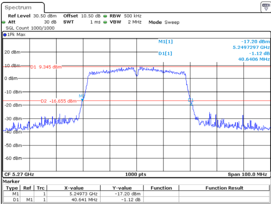
802.11ac40_5270MHz_Chain 2 40.641MHz
