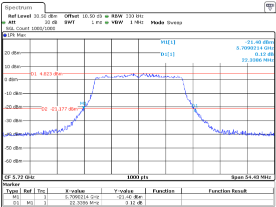
802.11ac20_5720MHz_Chain 0 22.339MHz
