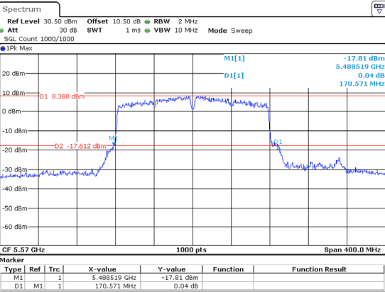
802.11ac160_5570MHz_Chain 1 170.571MHz
