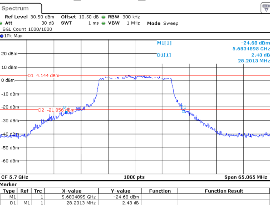
802.11ac20_5700MHz_Chain 0 28.201MHz
