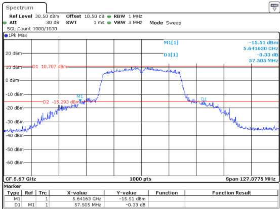
802.11ac40_5670MHz_Chain 2 57.505MHz
