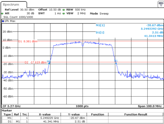
802.11ac40_5270MHz_Chain 0 41.341MHz
