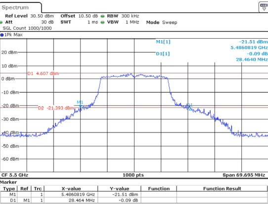
802.11ac20_5500MHz_Chain 0 28.464MHz
