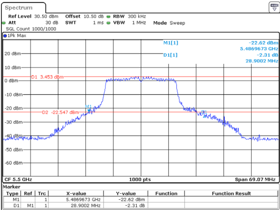
802.11ac20_5500MHz_Chain 2 28.900MHz
