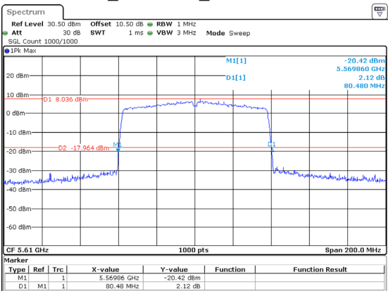
802.11ac80_5610MHz_Chain 0 80.480MHz
