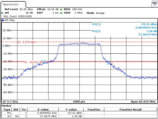
802.11ac20_5700MHz_Chain 1 27.067MHz
