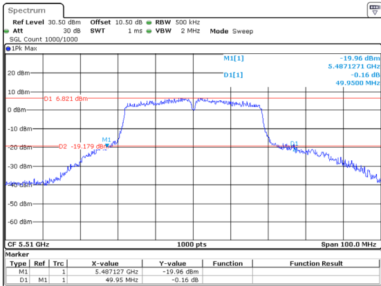
802.11ac40_5510MHz_Chain 2 49.950MHz
