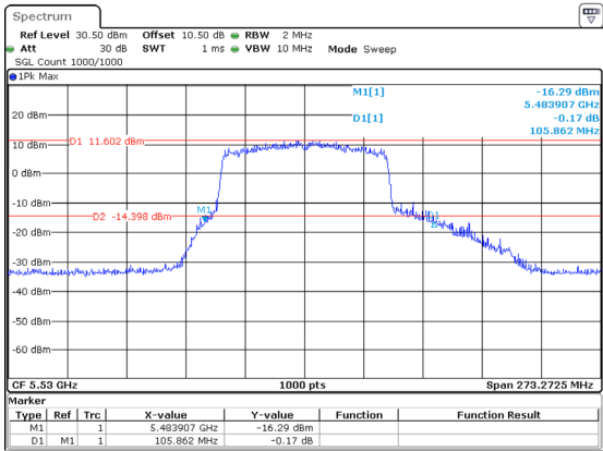
802.11ac80_5530MHz_Chain 0 105.862MHz
