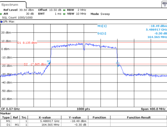
802.11ac160_5570MHz_Chain 2 164.565MHz
