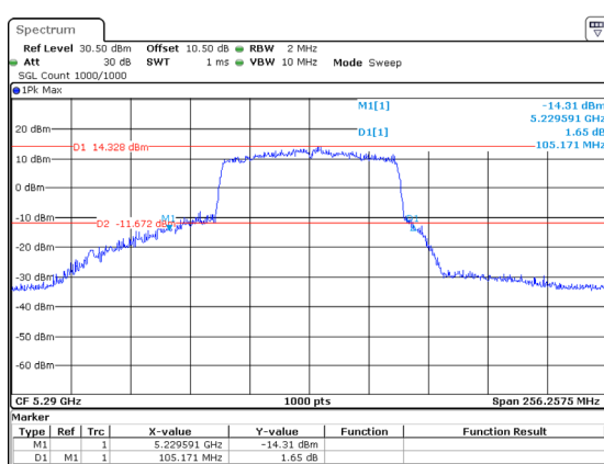
802.11ac80_5290MHz_Chain 2 105.171MHz
