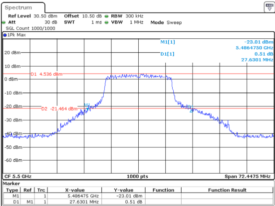
802.11ac20_5500MHz_Chain 1 27.630MHz
