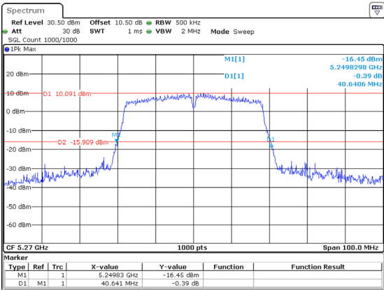
802.11ac40_5270MHz_Chain 1 40.641MHz
