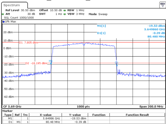
802.11ac80_5690MHz_Chain 0 80.480MHz
