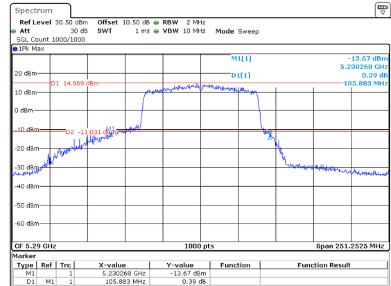
802.11ac80_5290MHz_Chain 1 105.883MHz
