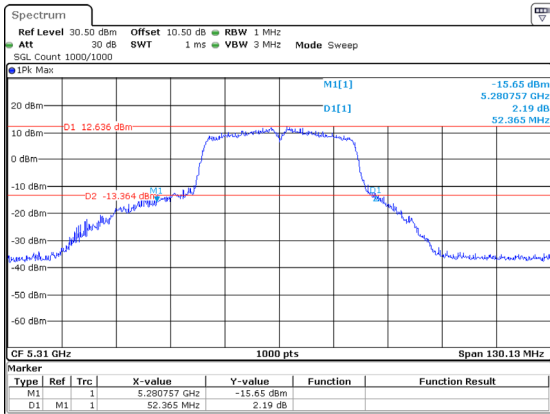
802.11ac40_5310MHz_Chain 2 52.365MHz
