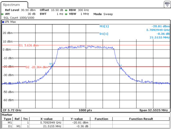
802.11ac20_5720MHz_Chain 1 21.515MHz
