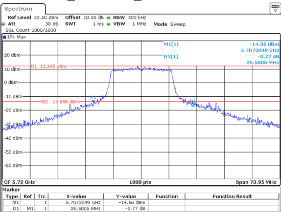
802.11a_5720MHz_Chain 2 26.501MHz
