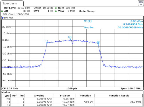
802.11ac40_5270MHz_Chain 0 36.300MHz
