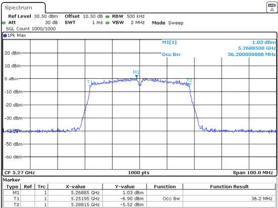
802.11ac40_5270MHz_Chain 2 36.200MHz
