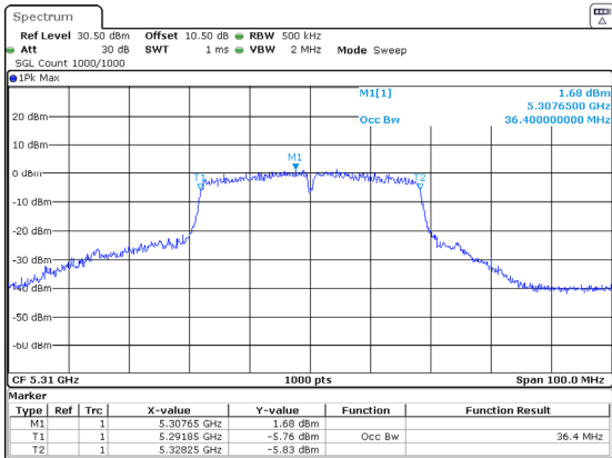
802.11ac40_5310MHz_Chain 1 36.400MHz
