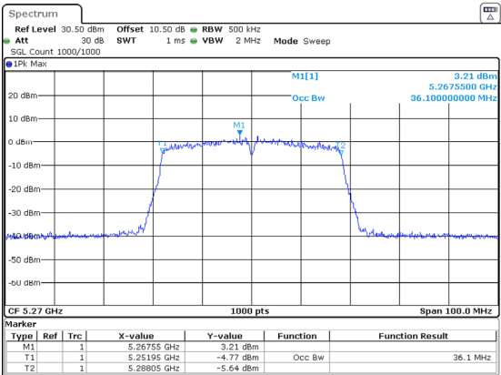
802.11ac40_5270MHz_Chain 1 36.100MHz
