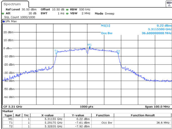
802.11ac40_5310MHz_Chain 0 36.600MHz
