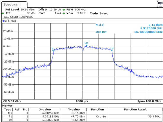
802.11ac40_5310MHz_Chain 2 36.400MHz
