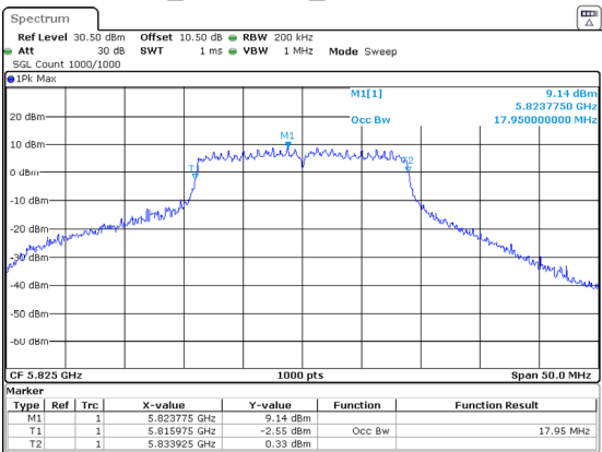
802.11ac20_5825MHz_Chain 1 17.950MHz
