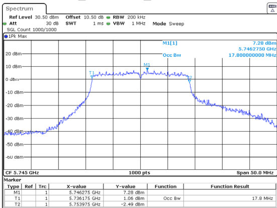
802.11ac20_5745MHz_Chain 2 17.800MHz
