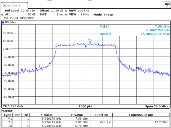
802.11ac20_5785MHz_Chain 2 17.700MHz
