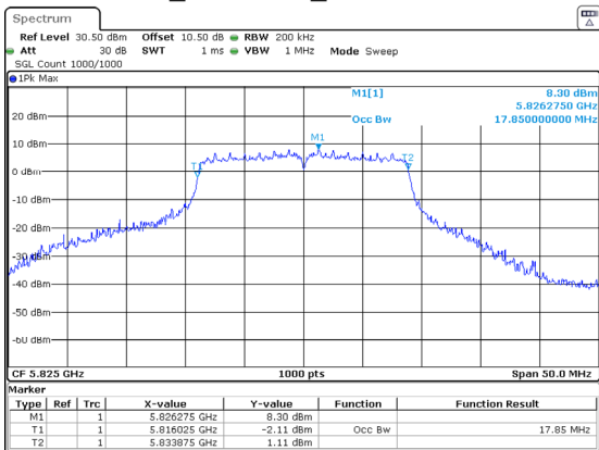
802.11ac20_5825MHz_Chain 2 17.850MHz
