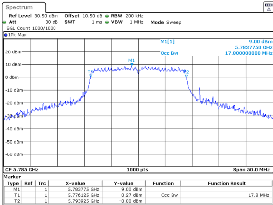
802.11ac20_5785MHz_Chain 1 17.800MHz
