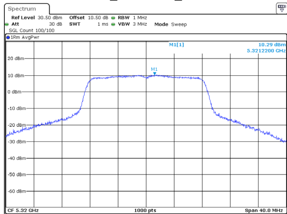
802.11a_5320MHz_Chain 2
