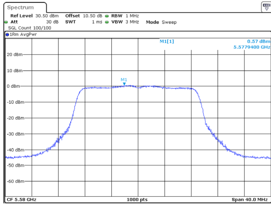
802.11ac20_5580MHz_Chain 2
