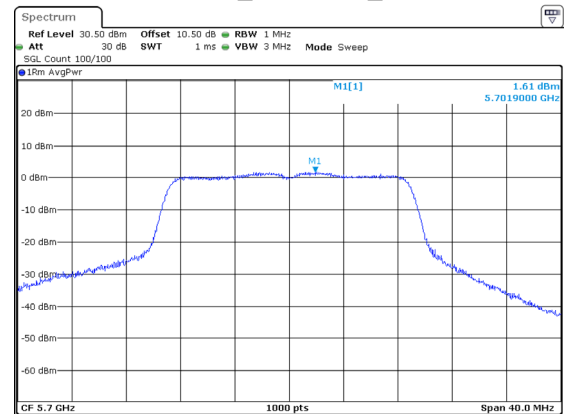
802.11ac20_5700MHz_Chain 1
