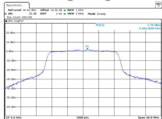
802.11ac20_5500MHz_Chain 1
