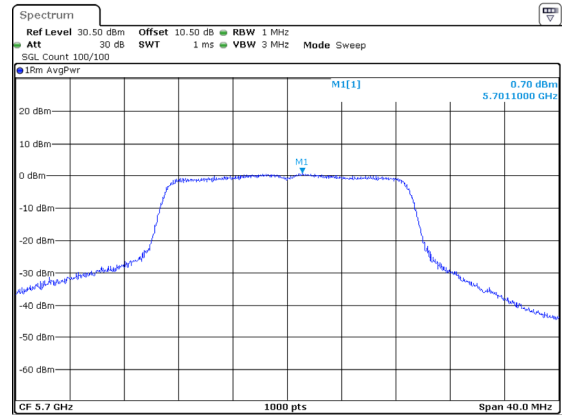
802.11ac20_5700MHz_Chain 2
