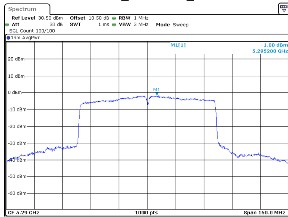
802.11ac80_5290MHz_Chain 2
