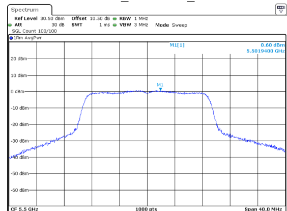
802.11ac20_5500MHz_Chain 2
