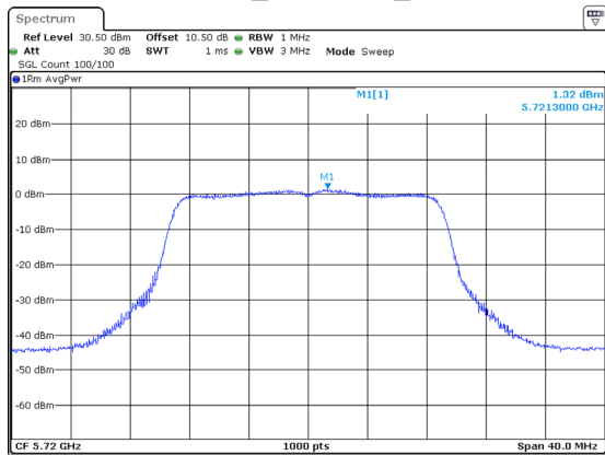
802.11ac20_5720MHz_Chain 2
