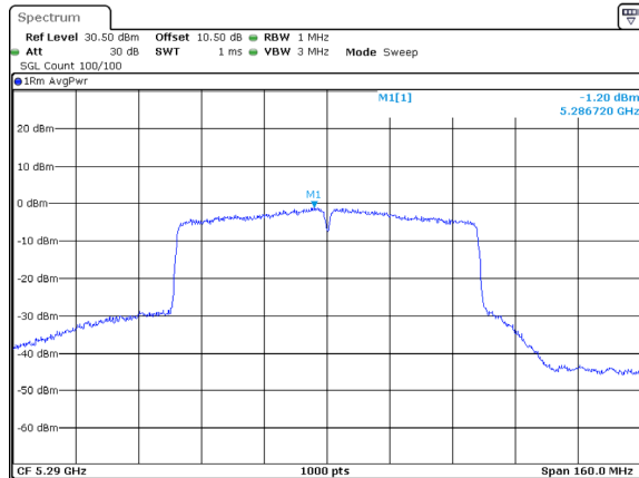
802.11ac80_5290MHz_Chain 0
