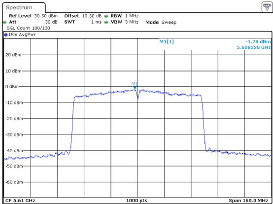
802.11ac80_5610MHz_Chain 1
