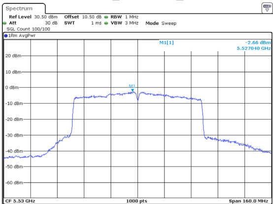
802.11ac80_5530MHz_Chain 2
