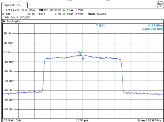
802.11ac80_5610MHz_Chain 2
