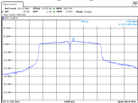
802.11ac40_5755MHz_Chain 2
