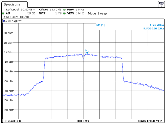
802.11ac80_5530MHz_Chain 1
