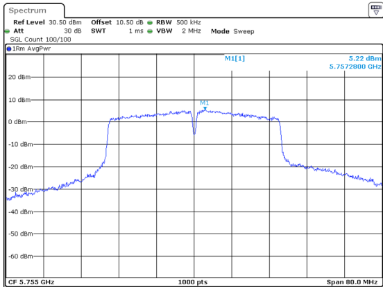
802.11ac40_5755MHz_Chain 0
