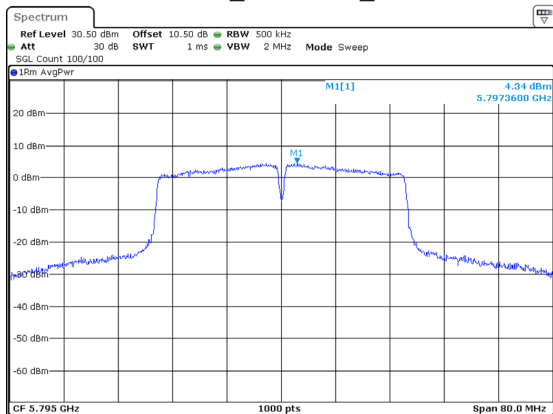
802.11ac40_5795MHz_Chain 2
