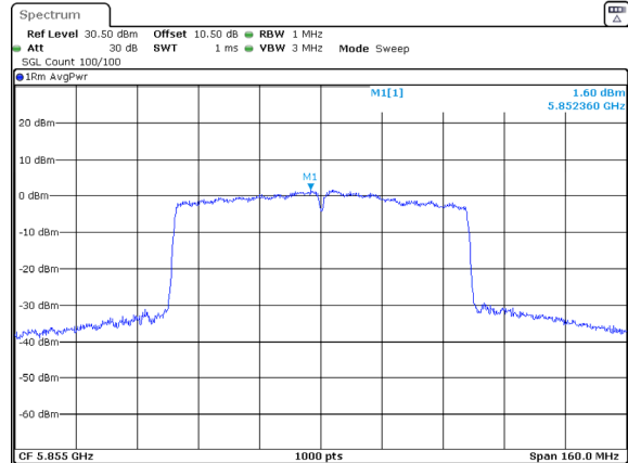
802.11ac80_5855MHz_Chain 1
