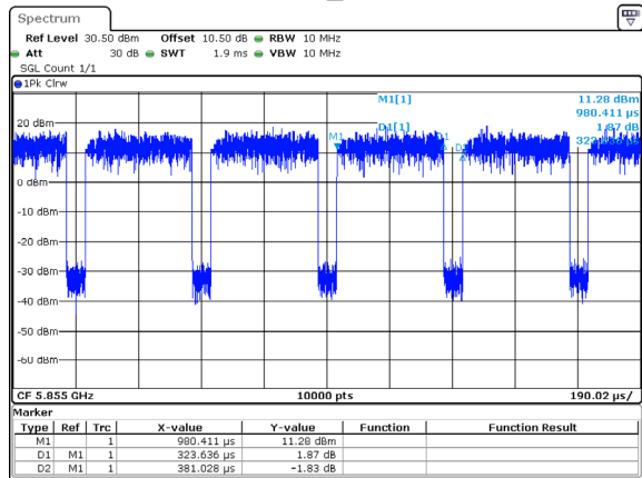
802.11ac80_5855MHz
