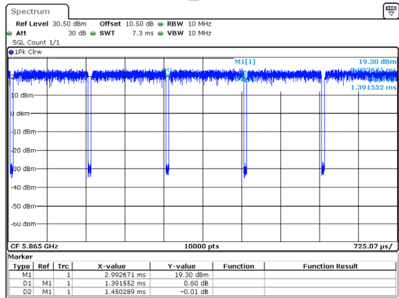
802.11a_5865MHz
