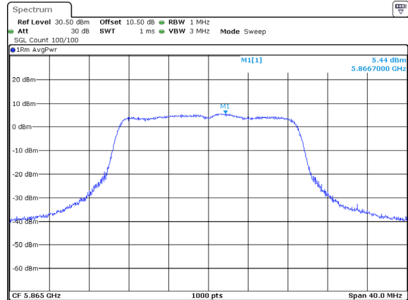
802.11ac20_5865MHz_Chain 1
