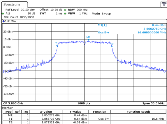
802.11a_5865MHz_Chain 2
