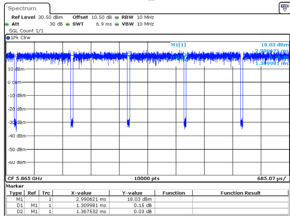
802.11ac20_5865MHz
