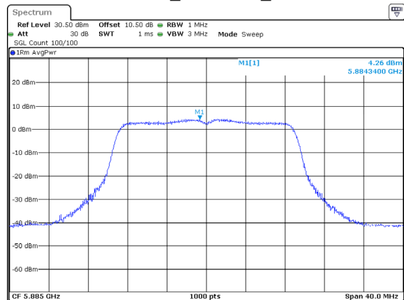
802.11ac20_5885MHz_Chain 2
