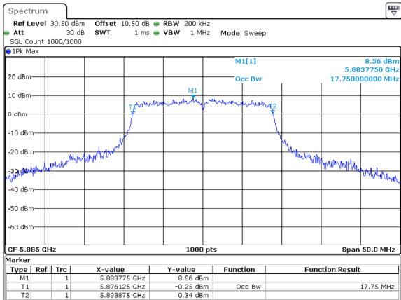
802.11ac20_5885MHz_Chain 0
