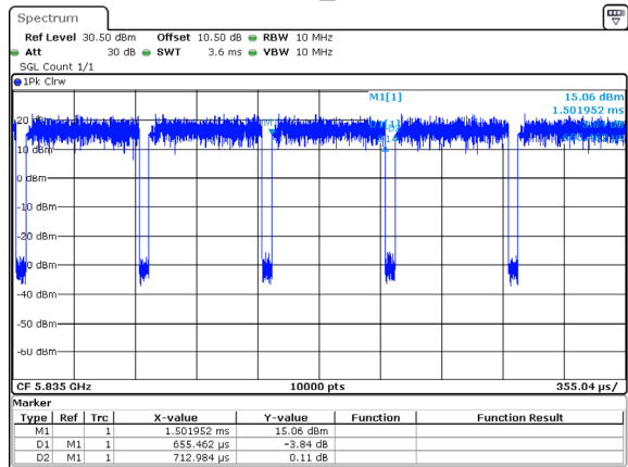
802.11ac40_5835MHz
