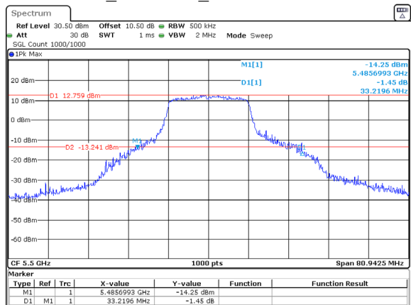
802.11a_5500MHz_Chain 1 33.220MHz
