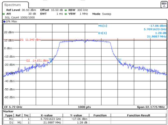
802.11a_5720MHz_Chain 0 21.989MHz
