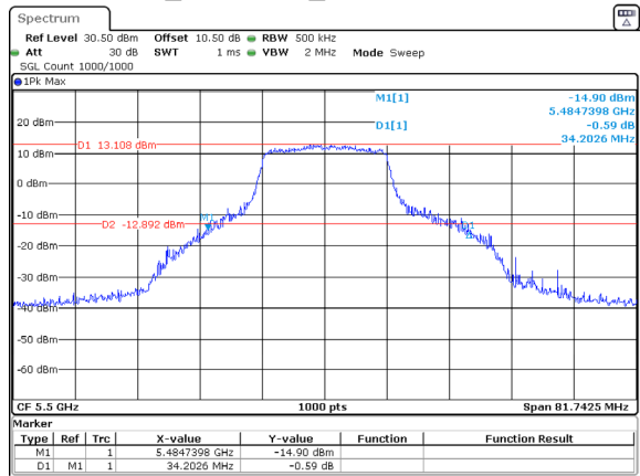
802.11a_5500MHz_Chain 0 34.203MHz
