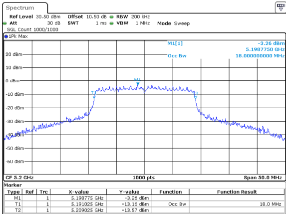
802.11ac20_5200MHz_Chain 1
