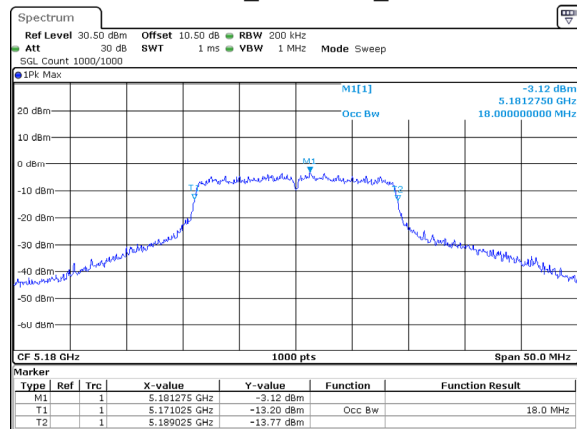
802.11ac20_5180MHz_Chain 0
