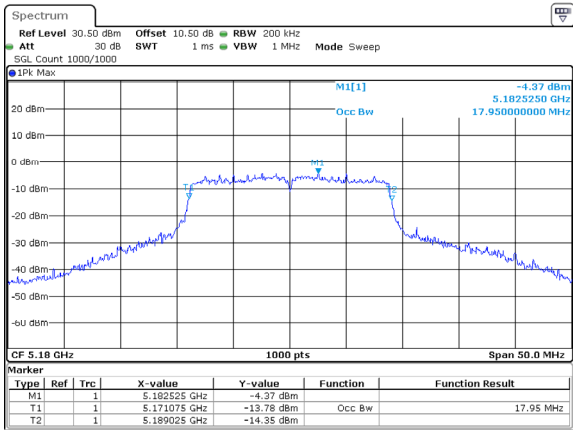
802.11ac20_5180MHz_Chain 2
