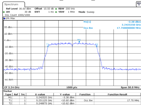
802.11ac20_5240MHz_Chain 0
