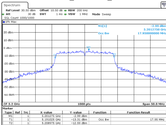
802.11ac20_5200MHz_Chain 0
