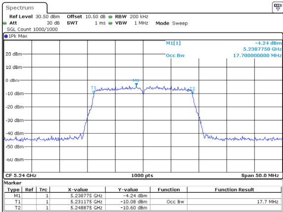
802.11ac20_5240MHz_Chain 2
