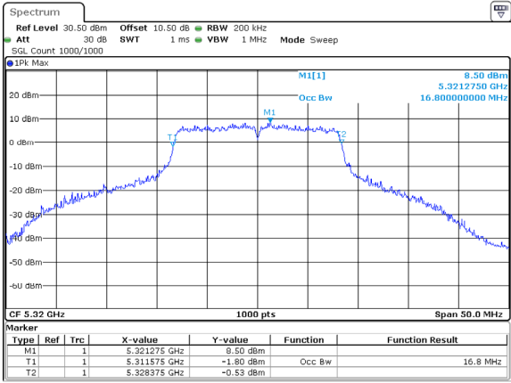
802.11a_5320MHz_Chain 1
