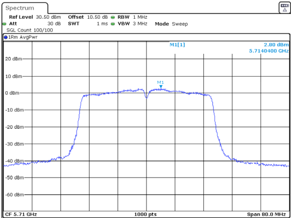
802.11ac40_5710MHz_Chain 1
