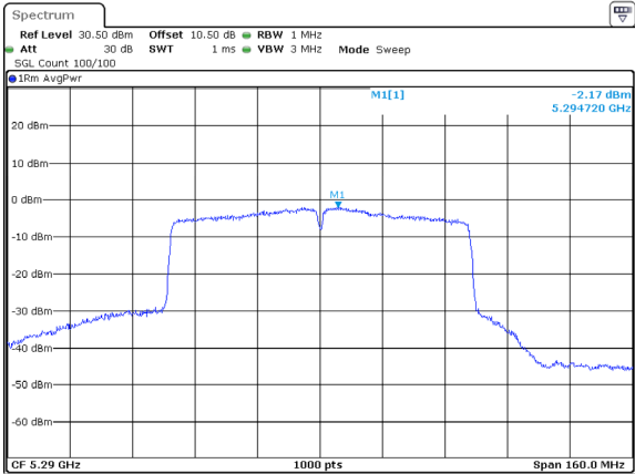
802.11ac80_5290MHz_Chain 2
