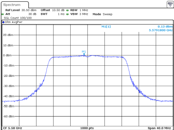
802.11ac20_5580MHz_Chain 2
