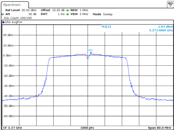
802.11ac40_5270MHz_Chain 2
