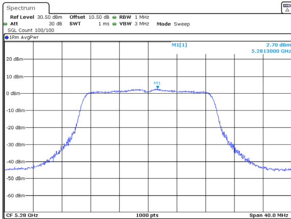
802.11ac20_5280MHz_Chain 0
