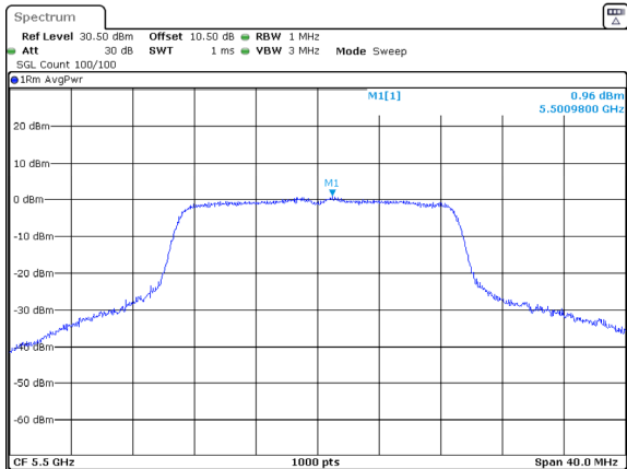
802.11ac20_5500MHz_Chain 1
