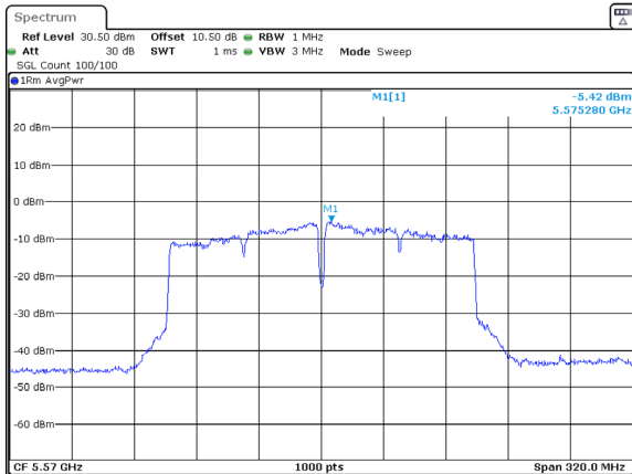
802.11ac160_5570MHz_Chain 1
