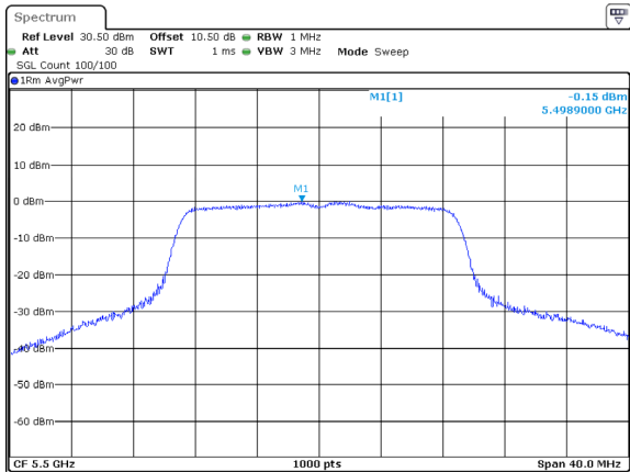
802.11ac20_5500MHz_Chain 2
