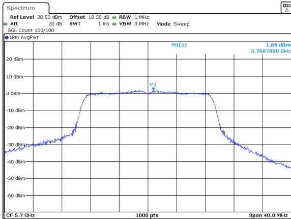
802.11ac20_5700MHz_Chain 0
