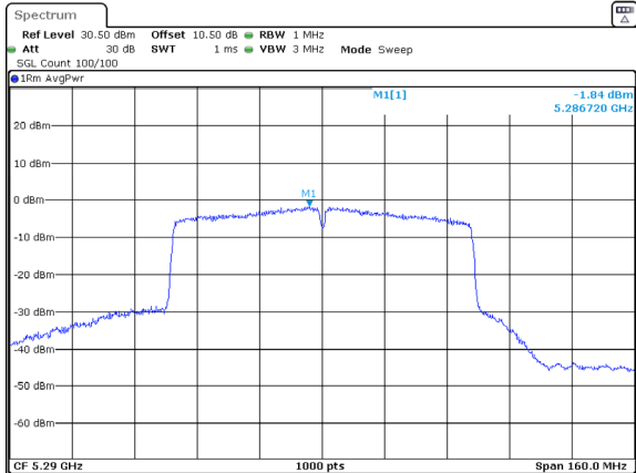
802.11ac80_5290MHz_Chain 1
