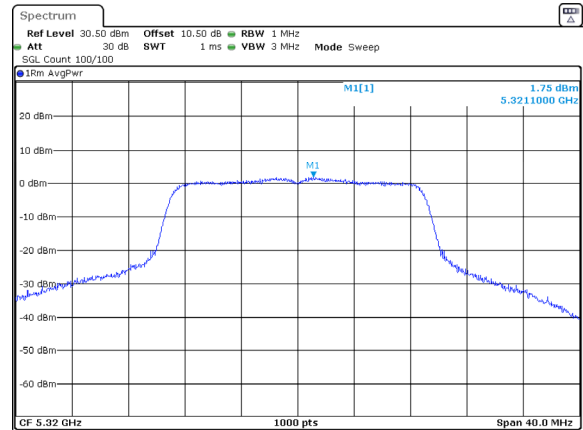
802.11ac20_5320MHz_Chain 0
