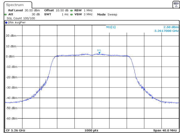
802.11ac20_5260MHz_Chain 0
