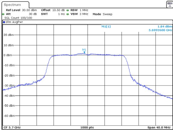
802.11ac20_5700MHz_Chain 1
