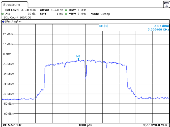
802.11ac160_5570MHz_Chain 0
