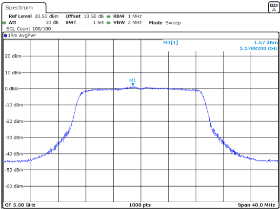
802.11ac20_5580MHz_Chain 1
