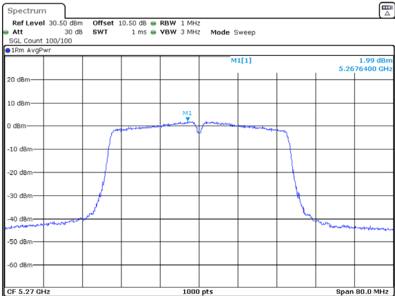
802.11ac40_5270MHz_Chain 0
