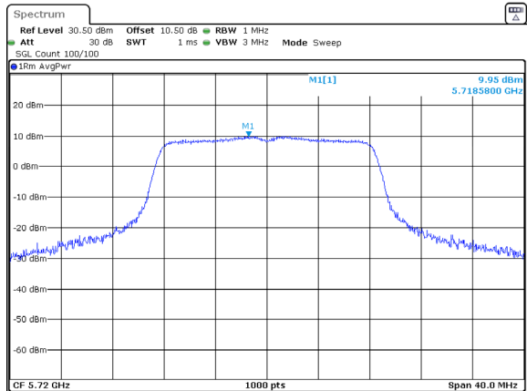
802.11a_5720MHz_Chain 1
