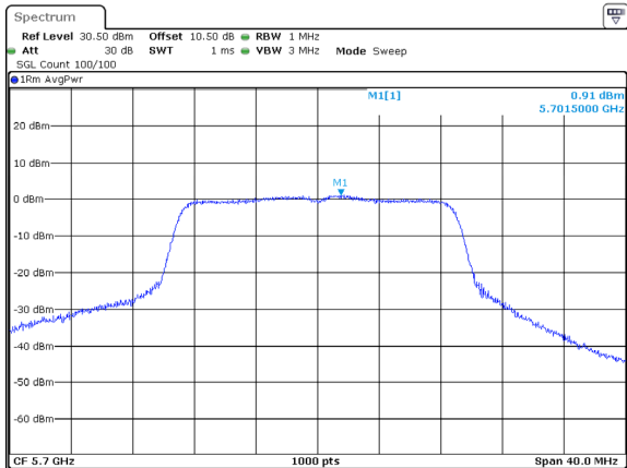
802.11ac20_5700MHz_Chain 2
