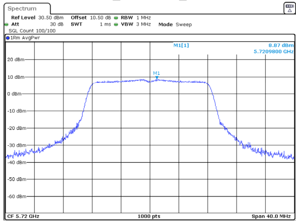
802.11a_5720MHz_Chain 0
