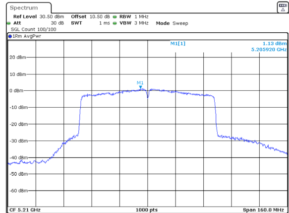
802.11ac80_5210MHz_Chain 1
