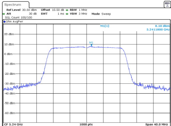
802.11ac20_5240MHz_Chain 0
