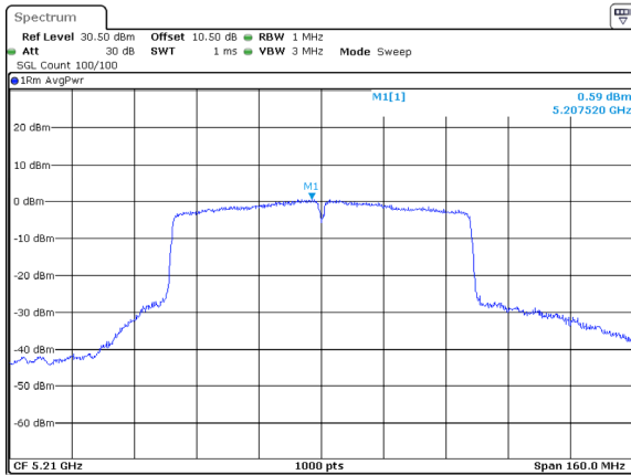
802.11ac80_5210MHz_Chain 2
