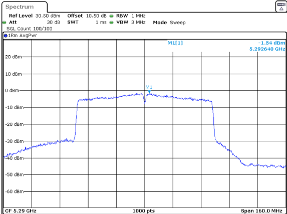
802.11ac80_5290MHz_Chain 0
