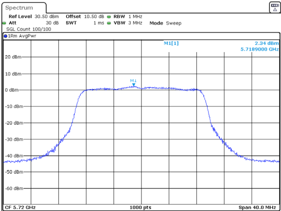
802.11ac20_5720MHz_Chain 1
