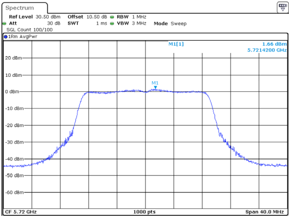
802.11ac20_5720MHz_Chain 2
