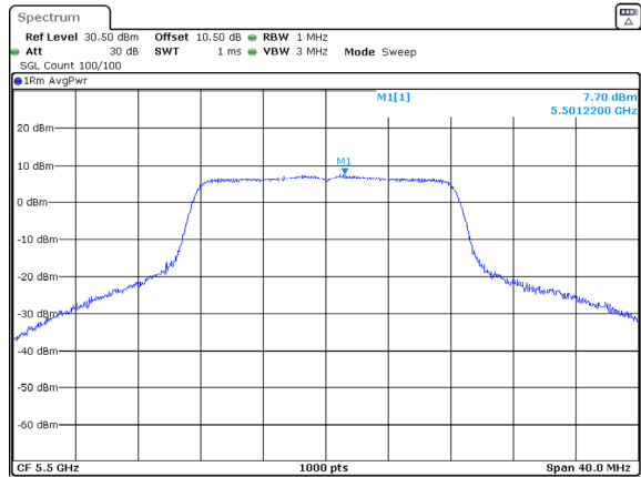
802.11a_5500MHz_Chain 2
