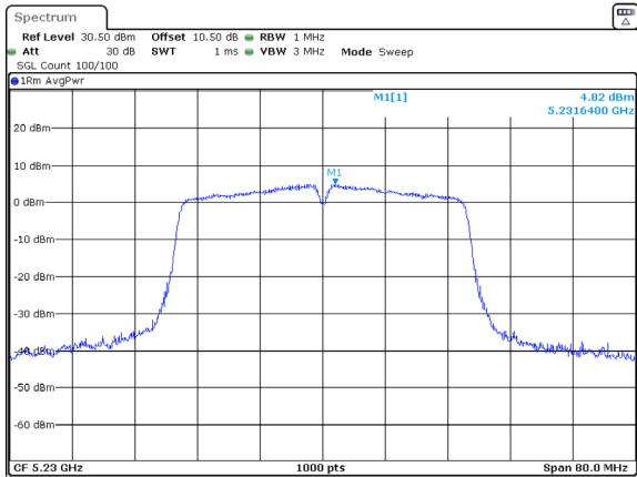
802.11ac40_5230MHz_Chain 1
