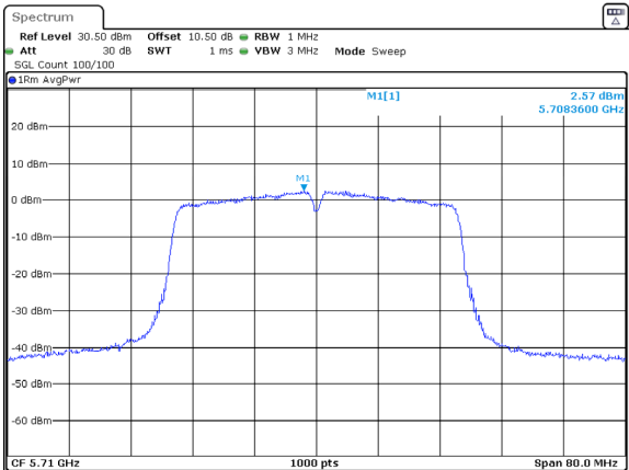
802.11ac40_5710MHz_Chain 0
