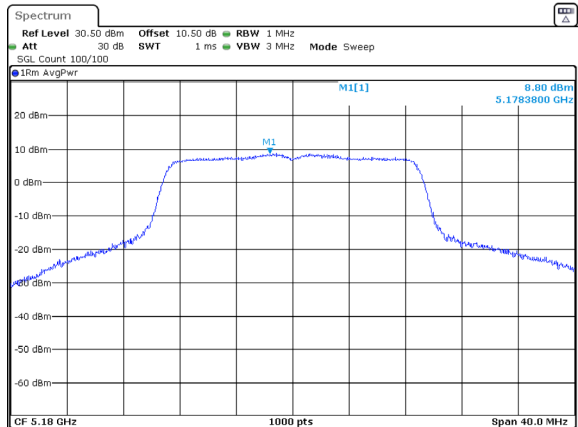
802.11ac20_5180MHz_Chain 0
