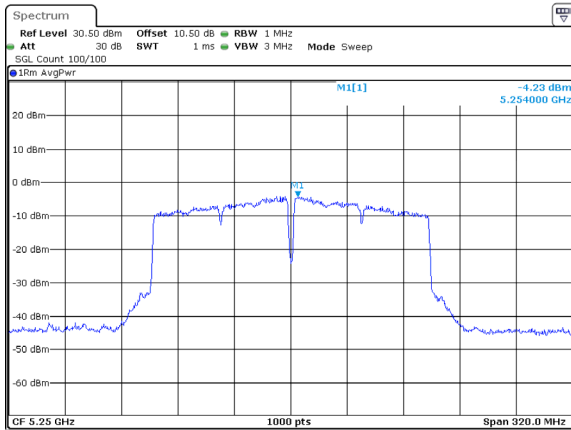
802.11ac160_5250MHz_Chain 2
