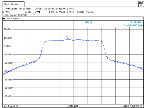
802.11a_5500MHz_Chain 1
