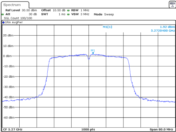
802.11ac40_5270MHz_Chain 1
