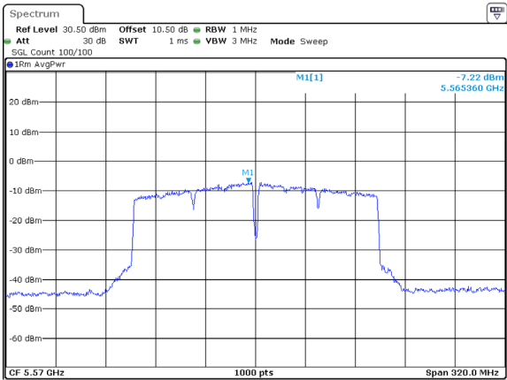
802.11ac160_5570MHz_Chain 2
