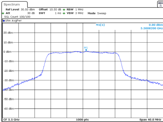
802.11ac20_5500MHz_Chain 0
