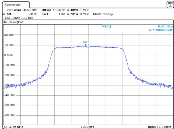
802.11a_5720MHz_Chain 2
