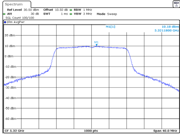
802.11a_5320MHz_Chain 1
