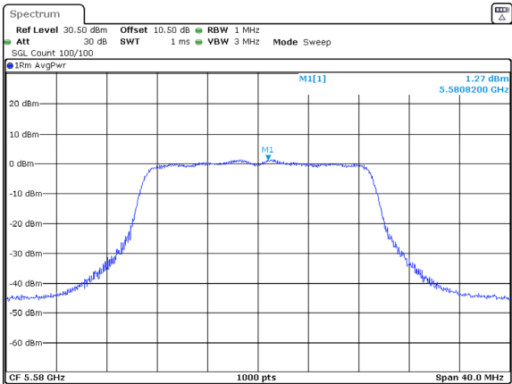
802.11ac20_5580MHz_Chain 0
