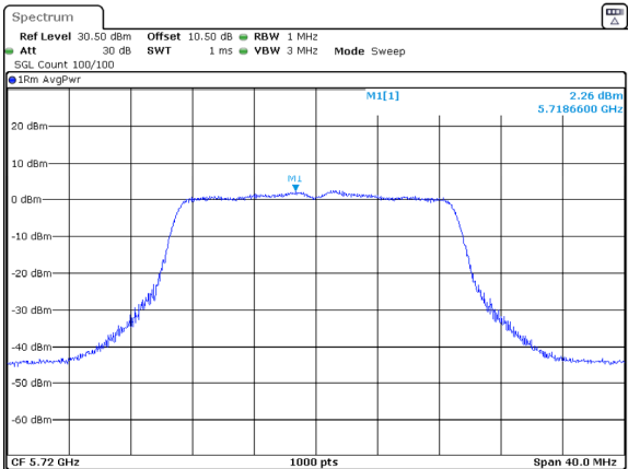
802.11ac20_5720MHz_Chain 0
