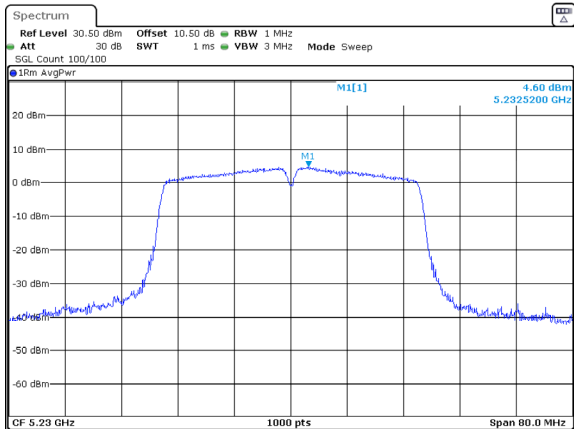
802.11ac40_5230MHz_Chain 0
