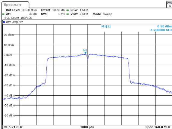
802.11ac80_5210MHz_Chain 0
