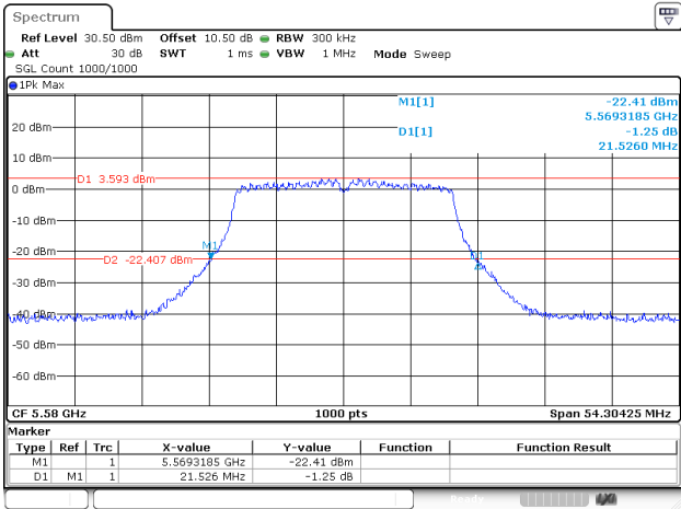
802.11ac20_5580MHz_Chain 2
