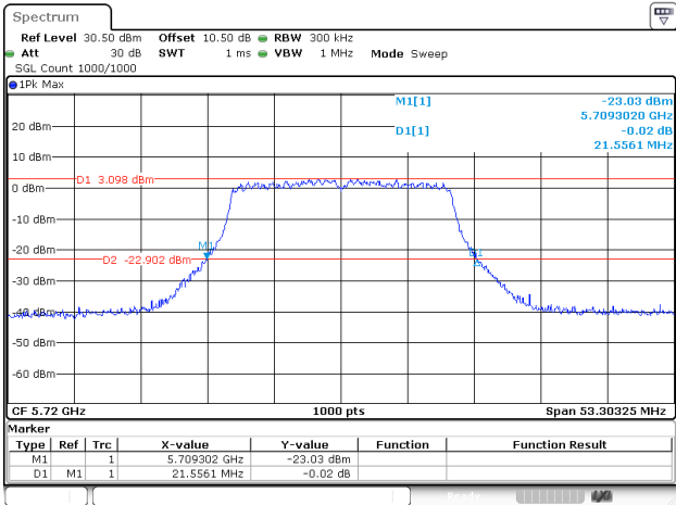
802.11ac20_5720MHz_Chain 2
