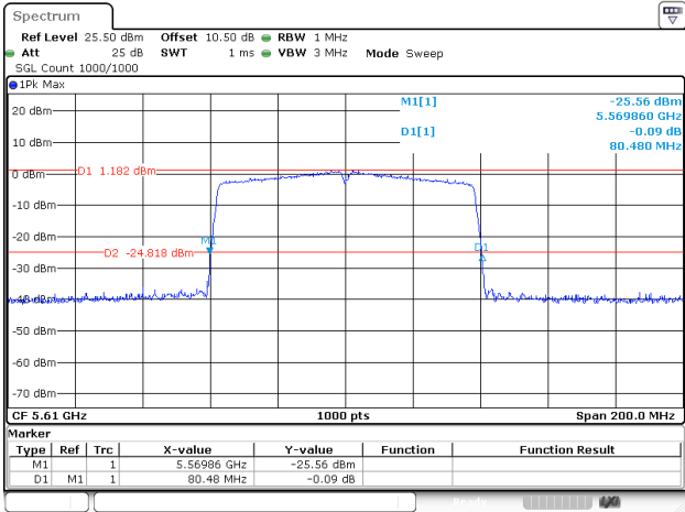
802.11ac80_5610MHz_Chain 0
