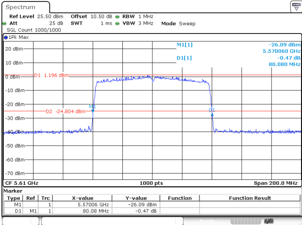
802.11ac80_5610MHz_Chain 2
