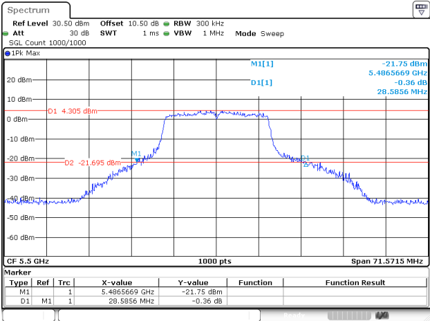
802.11ac20_5500MHz_Chain 0
