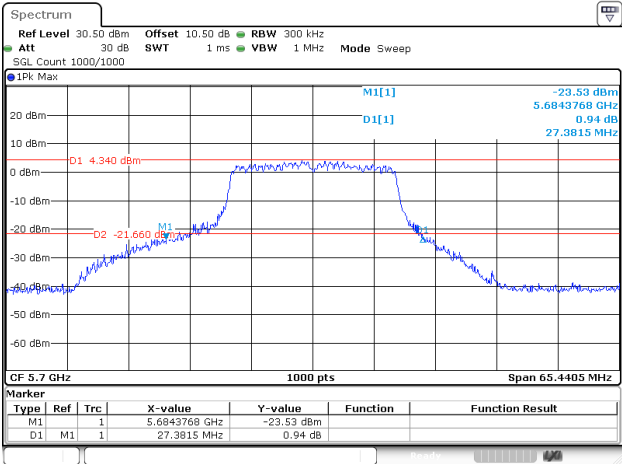
802.11ac20_5700MHz_Chain 1
