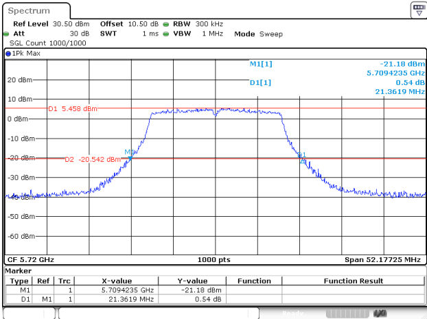
802.11a_5720MHz_Chain 2
