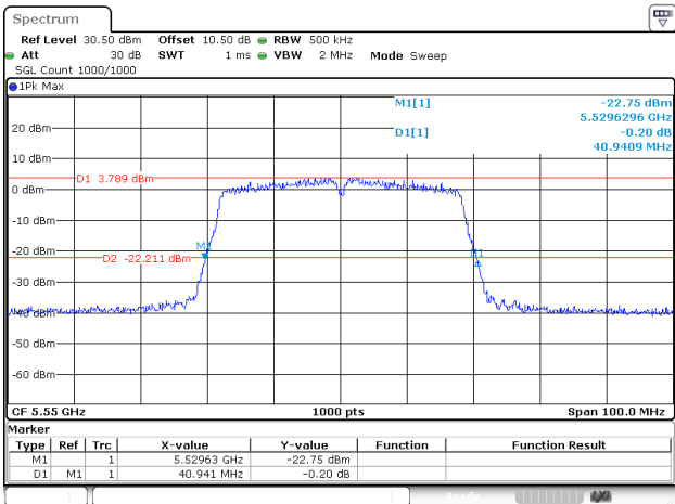
802.11ac40_5550MHz_Chain 2
