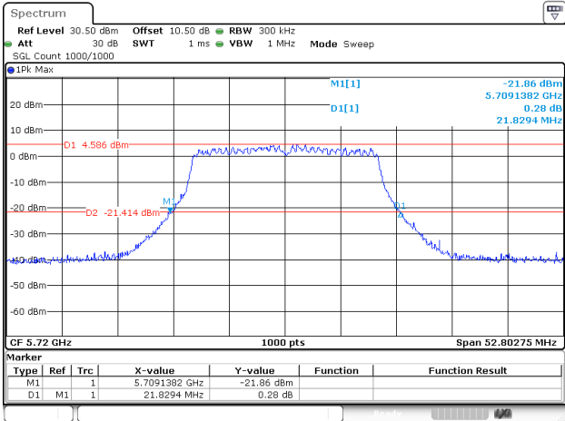
802.11ac20_5720MHz_Chain 1
