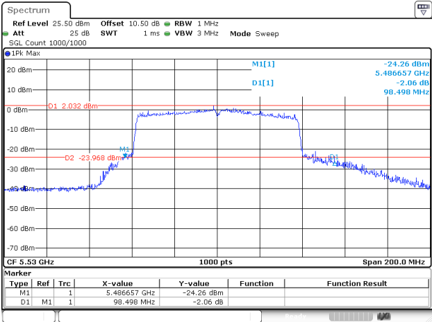
802.11ac80_5530MHz_Chain 2
