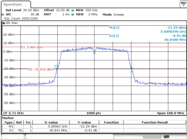
802.11ac40_5710MHz_Chain 1
