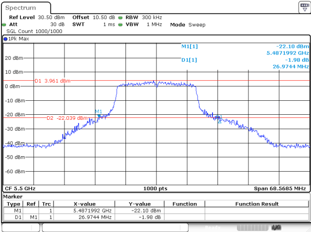
802.11ac20_5500MHz_Chain 2
