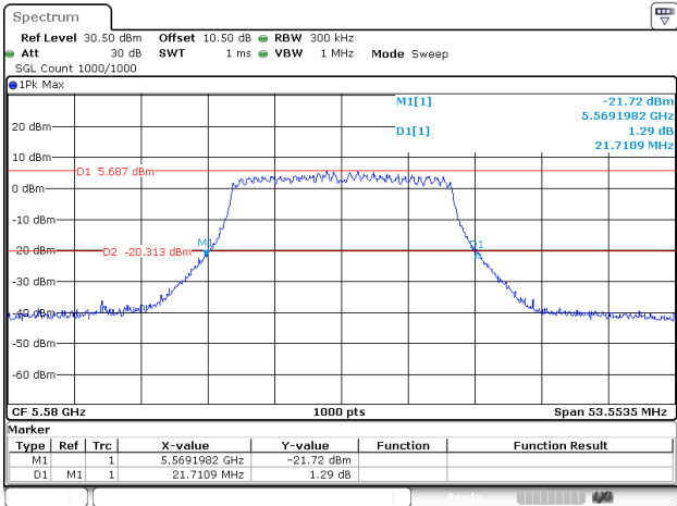
802.11ac20_5580MHz_Chain 1
