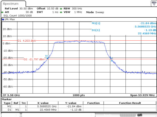
802.11ac20_5580MHz_Chain 0
