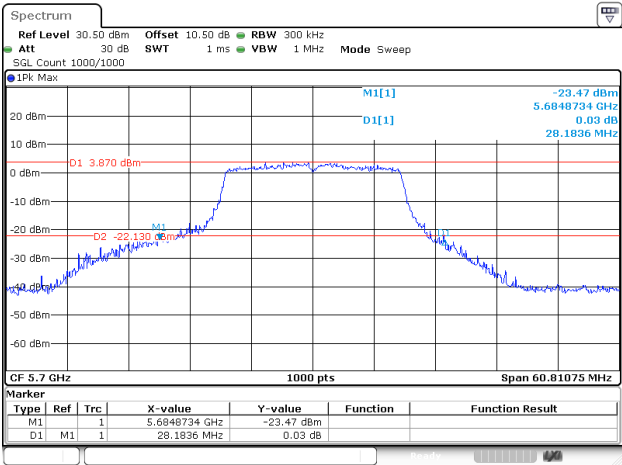
802.11ac20_5700MHz_Chain 0
