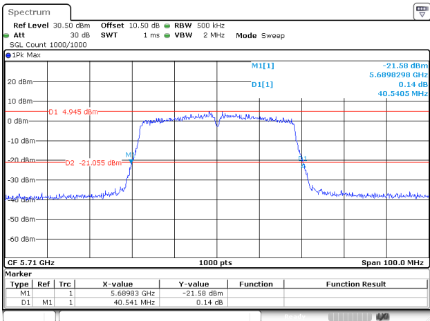
802.11ac40_5710MHz_Chain 2
