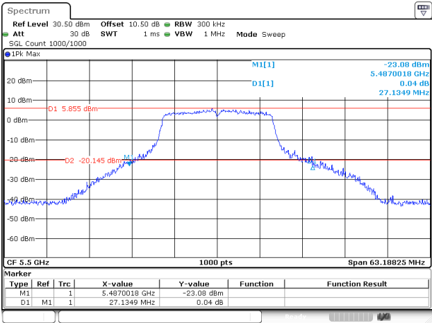
802.11a_5500MHz_Chain 2
