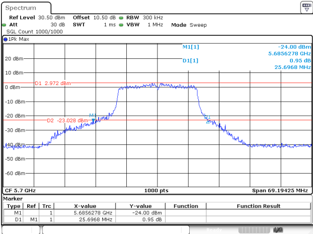
802.11ac20_5700MHz_Chain 2
