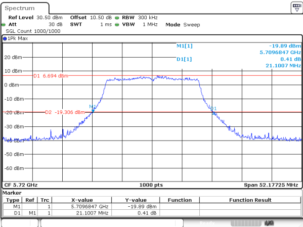
802.11a_5720MHz_Chain 0
