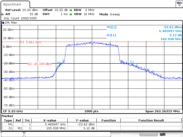
802.11ac80_5530MHz_Chain 0
