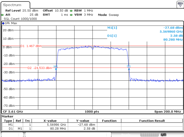
802.11ac80_5610MHz_Chain 1
