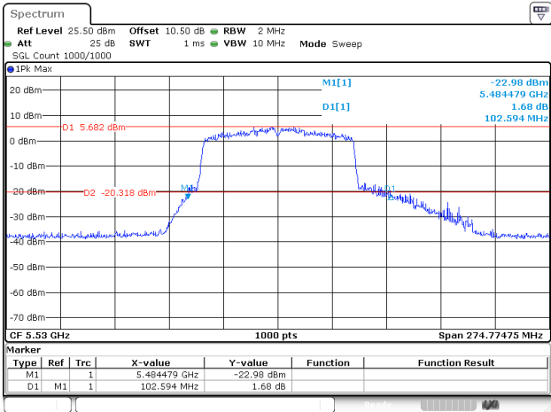
802.11ac80_5530MHz_Chain 1
