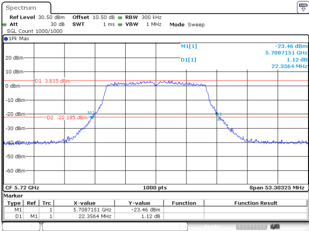
802.11ac20_5720MHz_Chain 0
