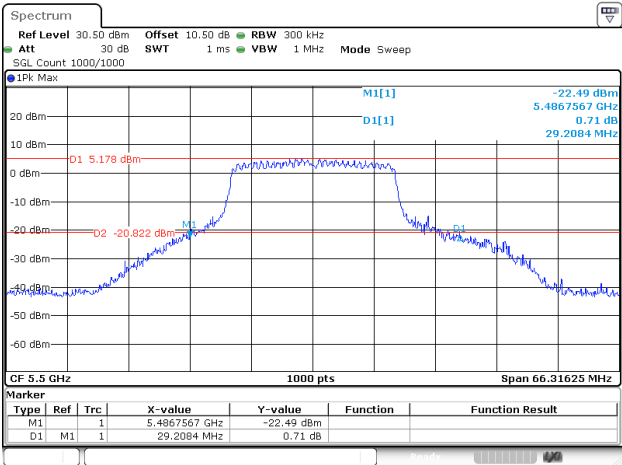
802.11ac20_5500MHz_Chain 1
