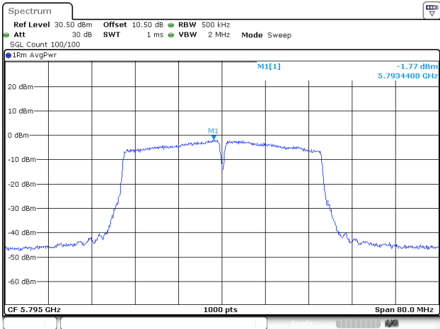
802.11ac40_5795MHz_Chain 2
