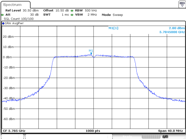
802.11ac20_5785MHz_Chain 2
