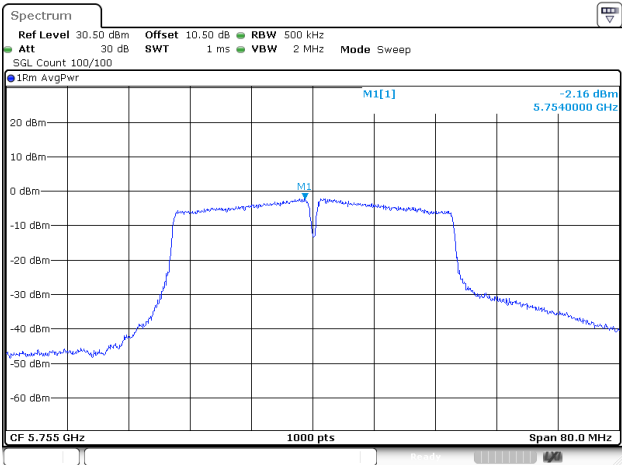
802.11ac40_5755MHz_Chain 2
