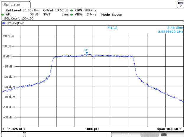
802.11ac20_5825MHz_Chain 2
