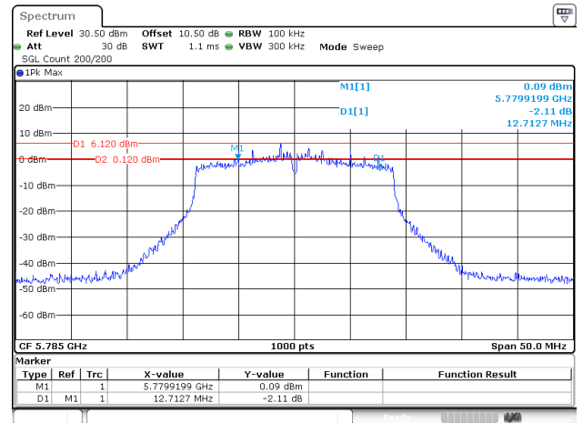
802.11ac20_5785MHz_ANT1
