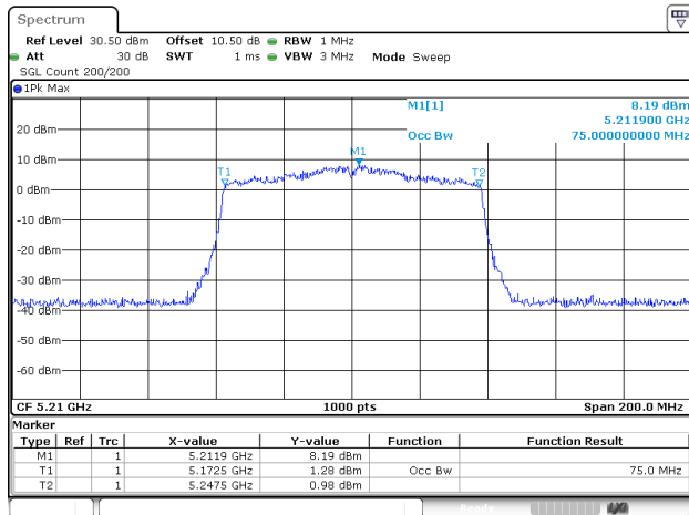
802.11ac80_5210MHz_ANT1
