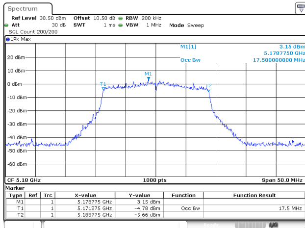
802.11ac20_5180MHz_ANT1
