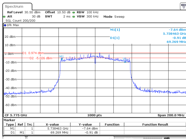
802.11ac80_5775MHz_ANT1
