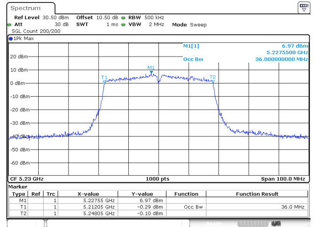
802.11ac40_5230MHz_ANT2
