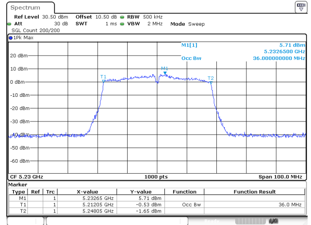
802.11ac40_5230MHz_ANT1
