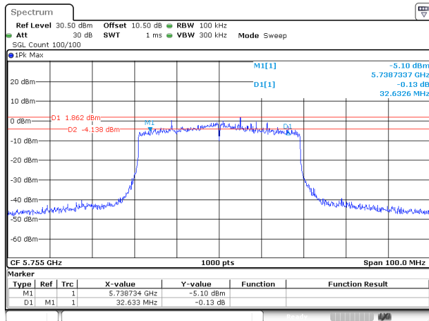
802.11ax40_5755MHz_RU_Full_ANT1
