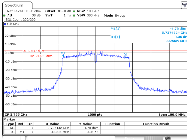
802.11ac40_5755MHz_ANT1
