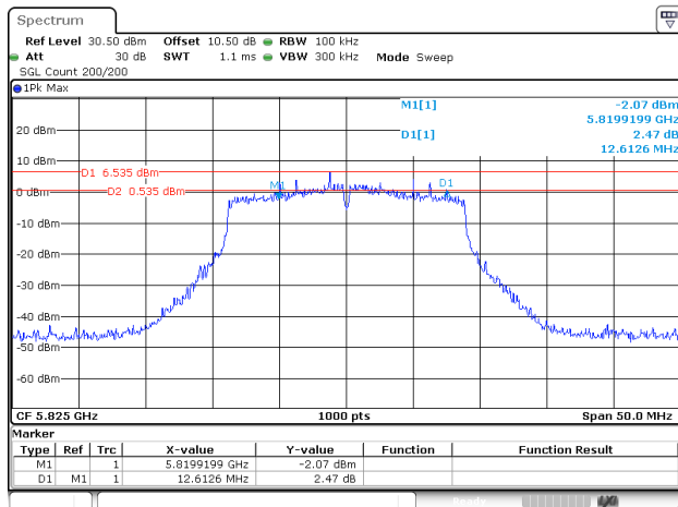
802.11ac20_5825MHz_ANT1
