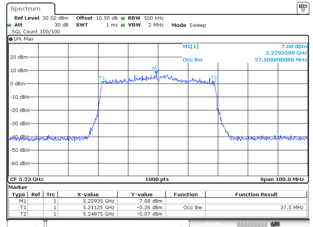
802.11ax40_5230MHz_RU_Full_ANT1
