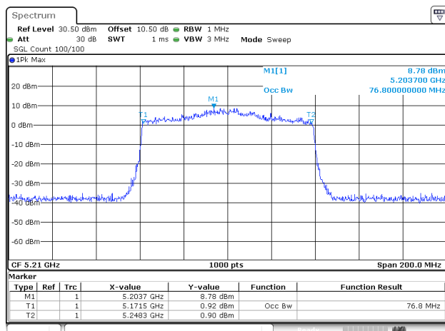
802.11ax80_5210MHz_RU_Full_ANT1
