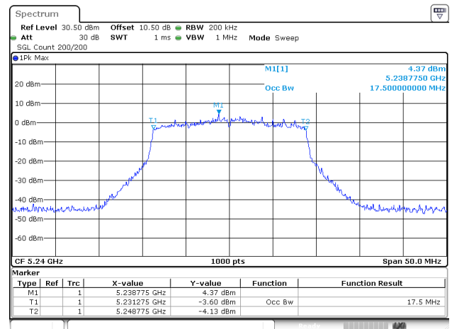
802.11ac20_5240MHz_ANT2
