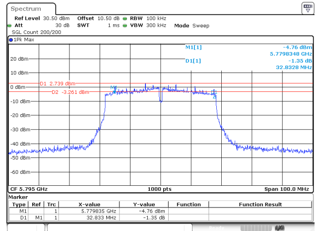
802.11ac40_5795MHz_ANT1
