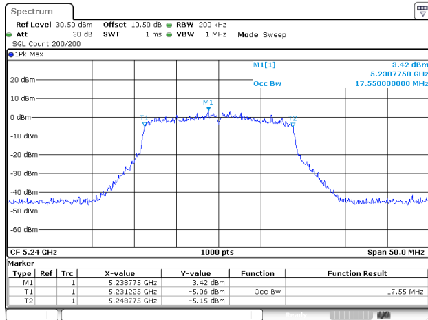
802.11ac20_5240MHz_ANT1
