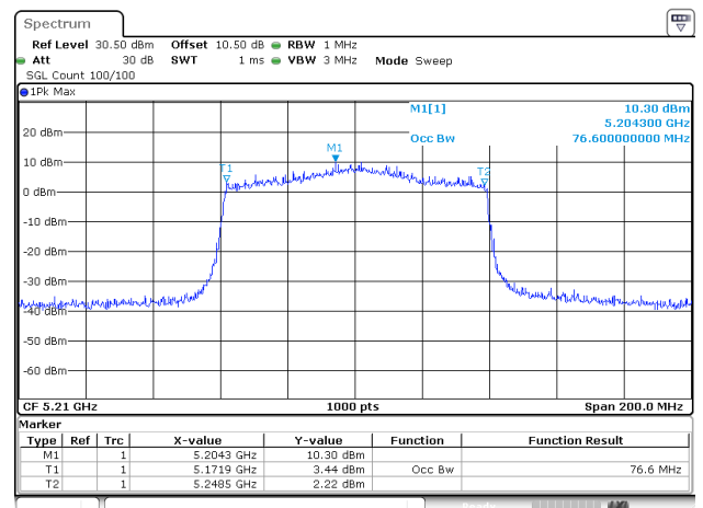
802.11ax80_5210MHz_RU_Full_ANT2
