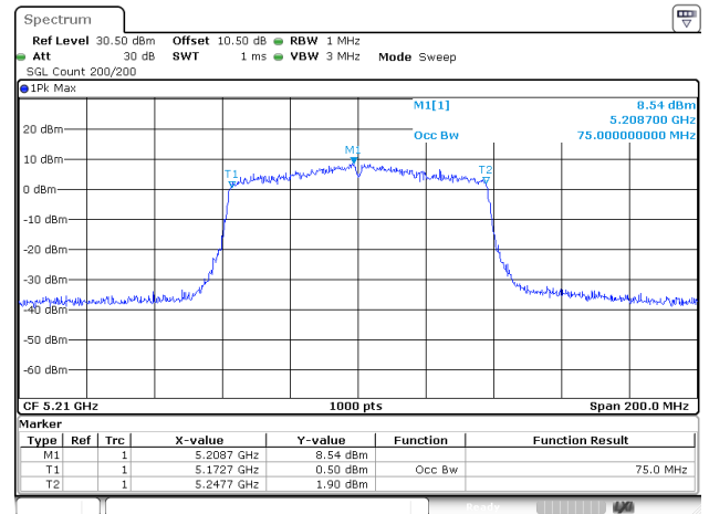
802.11ac80_5210MHz_ANT2
