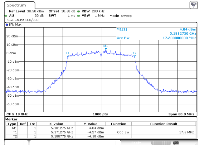
802.11ac20_5180MHz_ANT2
