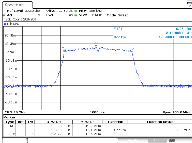
802.11ac40_5190MHz_ANT1
