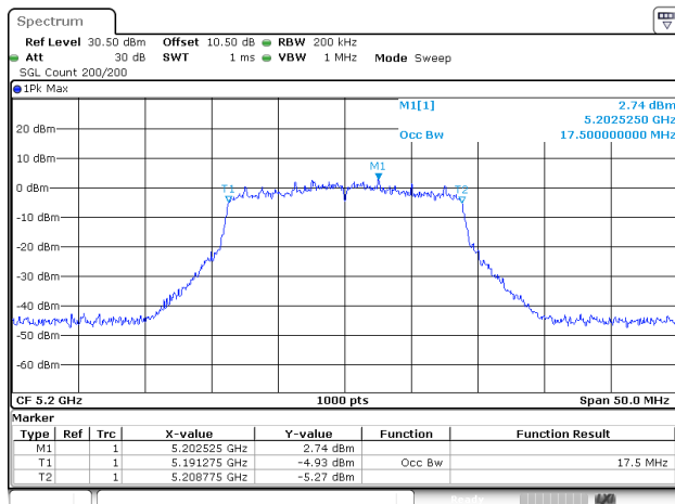
802.11ac20_5200MHz_ANT2
