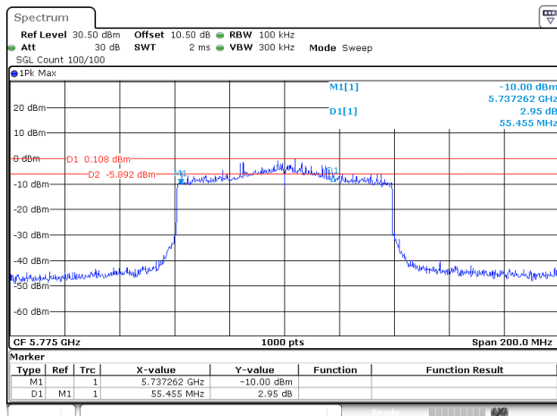
802.11ax80_5775MHz_RU_Full_ANT1
