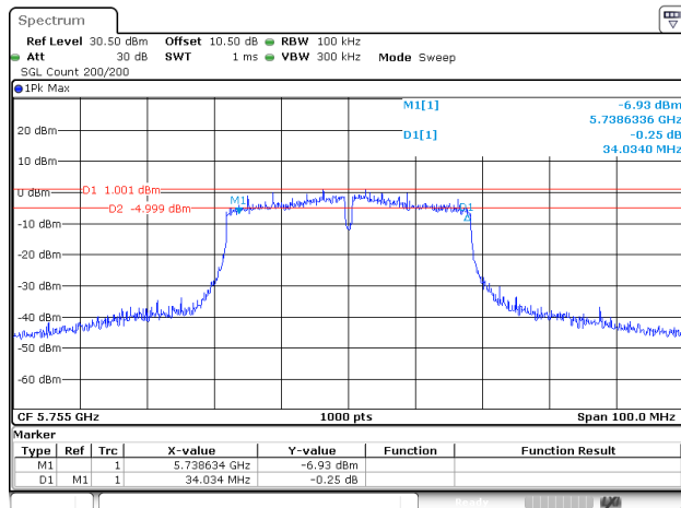
802.11ac40_5755MHz_ANT2
