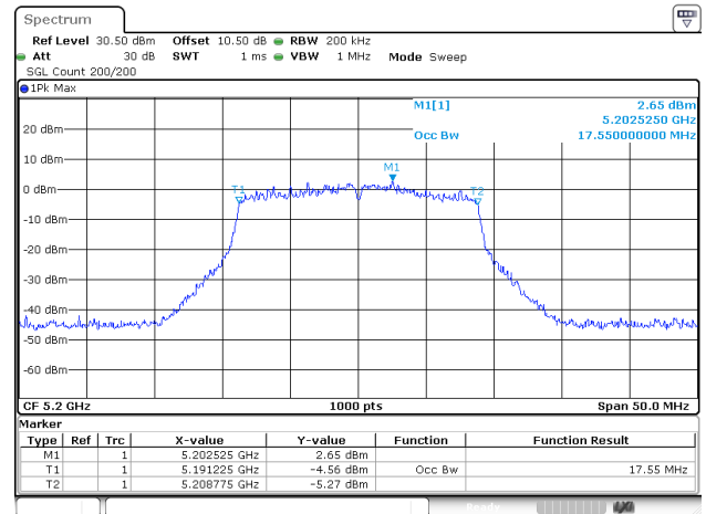
802.11ac20_5200MHz_ANT1
