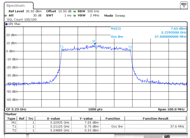
802.11ax40_5230MHz_RU_Full_ANT2
