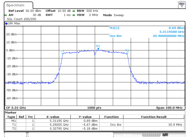
802.11ac40_5310MHz_ANT1
