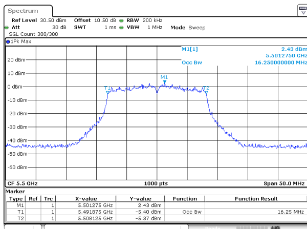
802.11a_5500MHz_ANT1
