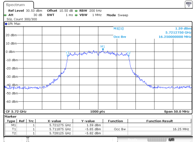
802.11a_5720MHz_ANT1
