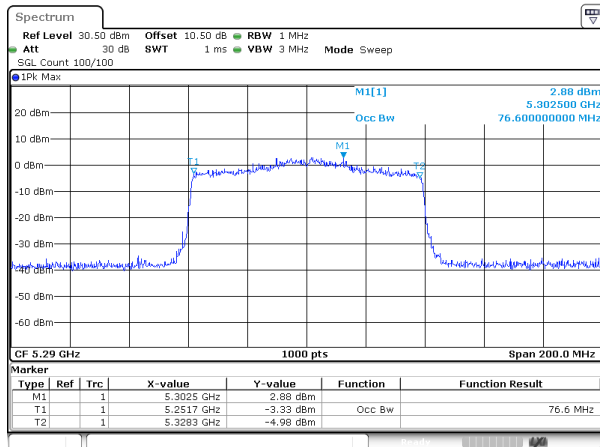
802.11ax80_5290MHz_RU_Full_ANT1
