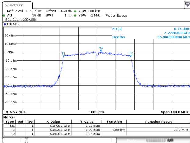
802.11ac40_5270MHz_ANT2
