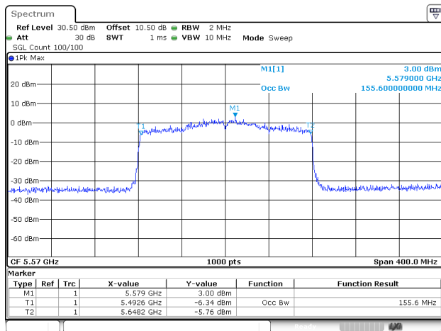
802.11ax160_5570MHz_RU_Full_ANT1
