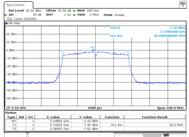
802.11ac40_5550MHz_ANT1
