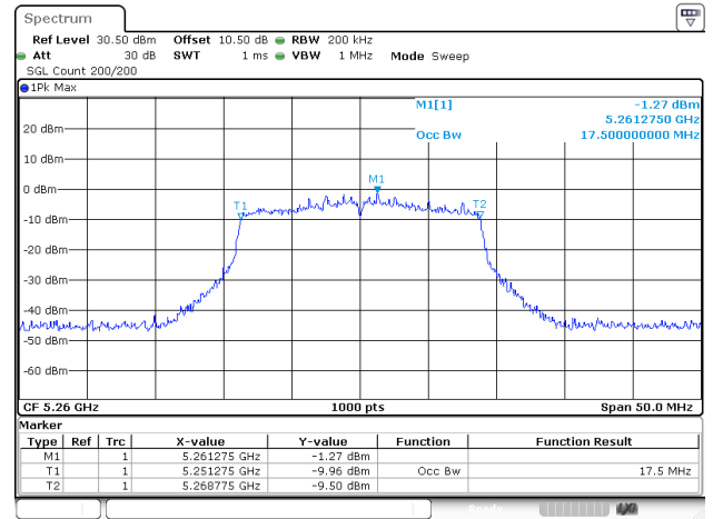
802.11ac20_5260MHz_ANT2
