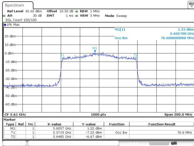
802.11ax80_5610MHz_RU_Full_ANT2
