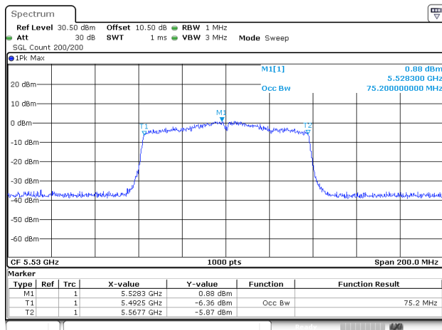
802.11ac80_5530MHz_ANT1
