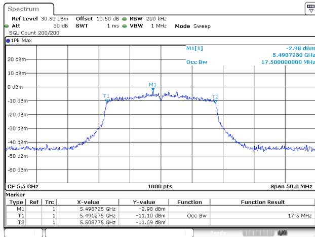
802.11ac20_5500MHz_ANT1
