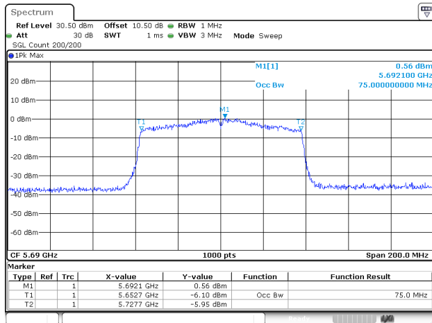
802.11ac80_5690MHz_ANT1
