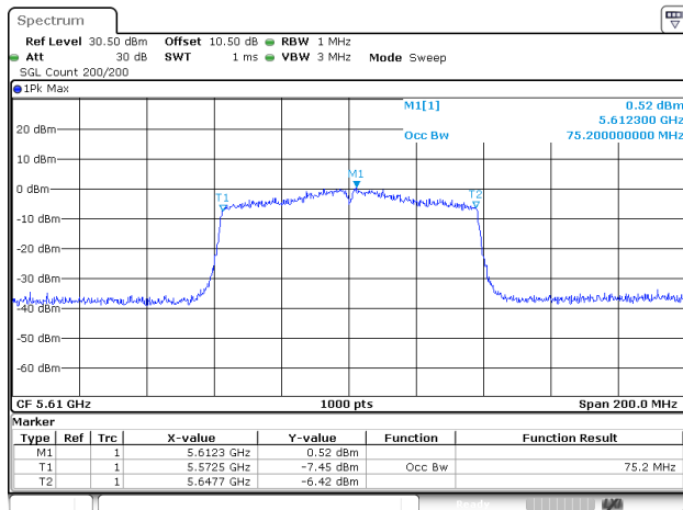
802.11ac80_5610MHz_ANT2
