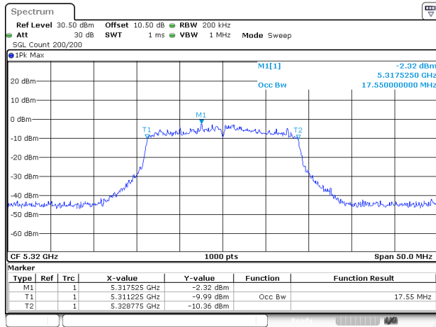
802.11ac20_5320MHz_ANT1
