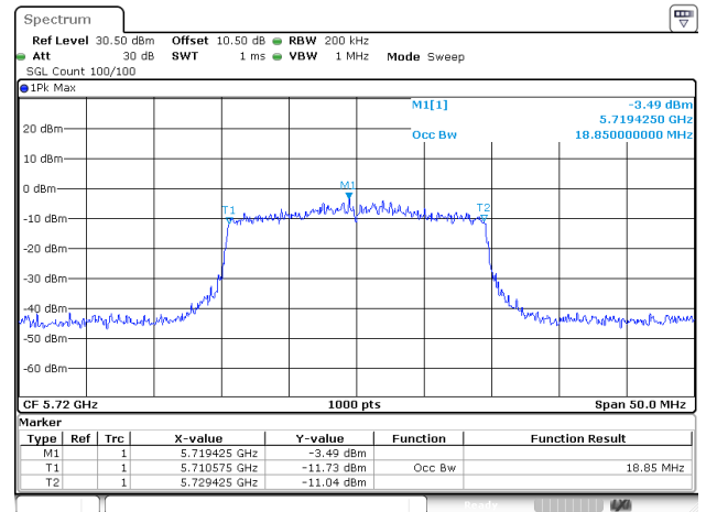
802.11ax20_5720MHz_RU_Full_ANT2
