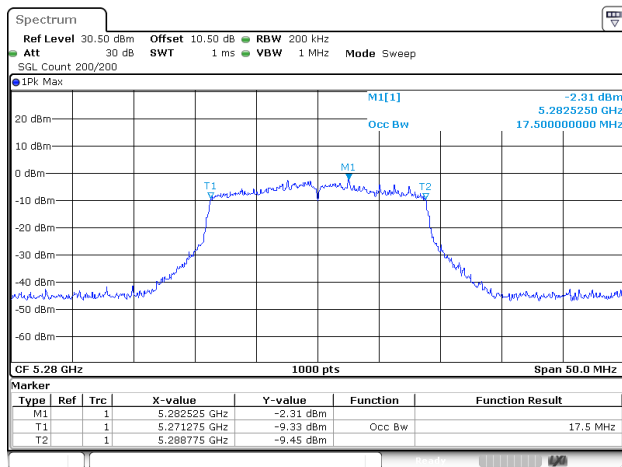
802.11ac20_5280MHz_ANT2
