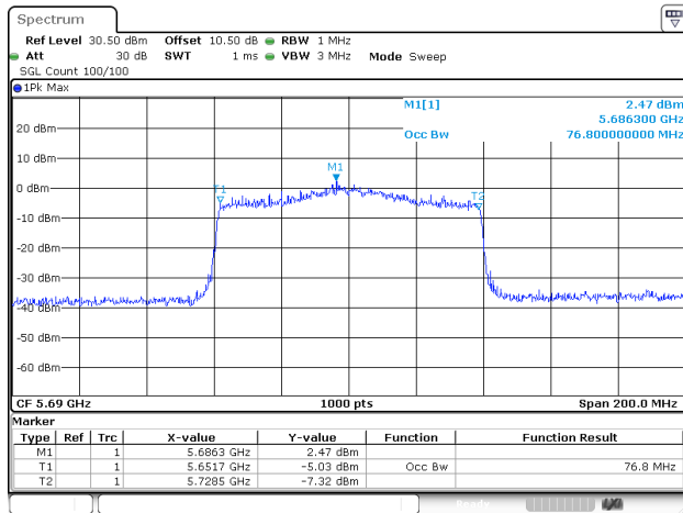
802.11ax80_5690MHz_RU_Full_ANT1
