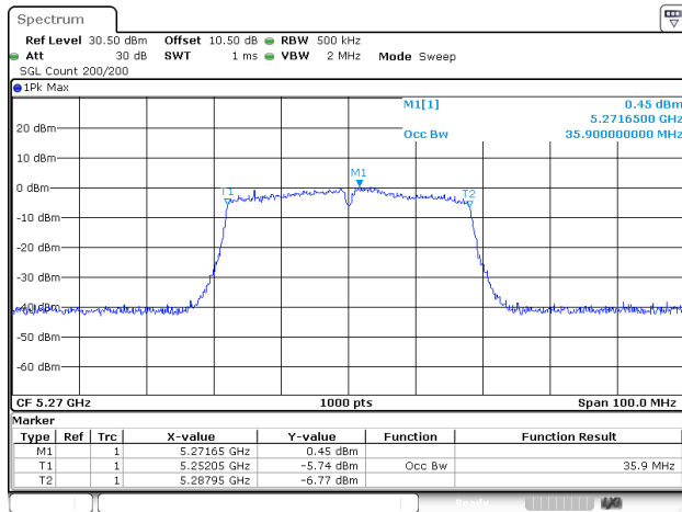
802.11ac40_5270MHz_ANT1
