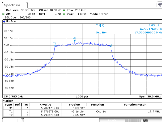
802.11ac20_5785MHz_ANT2
