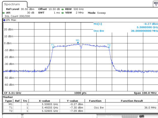
802.11ac40_5510MHz_ANT1
