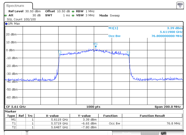
802.11ax80_5610MHz_RU_Full_ANT1
