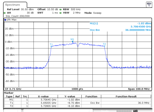
802.11ac40_5710MHz_ANT1
