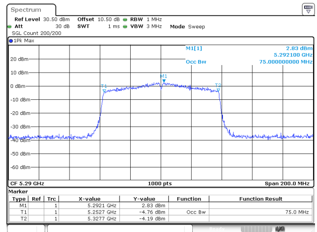
802.11ac80_5290MHz_ANT2
