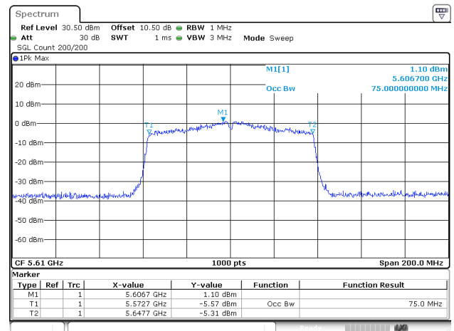
802.11ac80_5610MHz_ANT1
