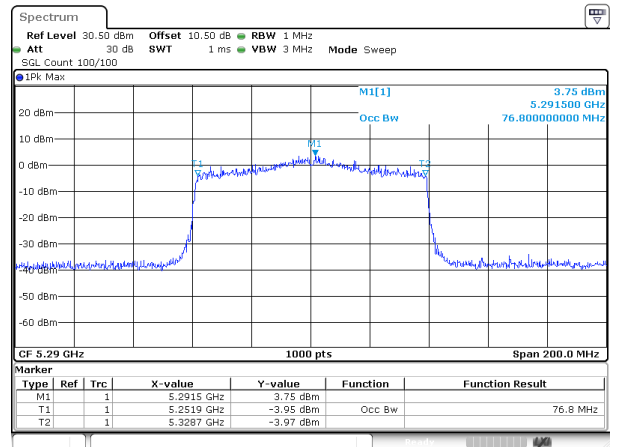
802.11ax80_5290MHz_RU_Full_ANT2
