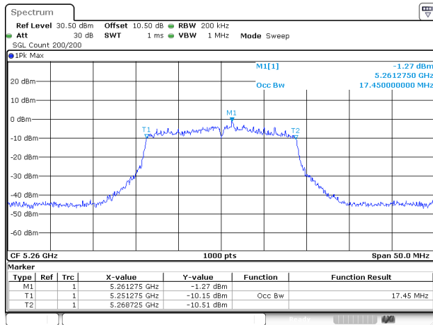
802.11ac20_5260MHz_ANT1
