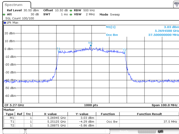
802.11ax40_5270MHz_RU_Full_ANT1
