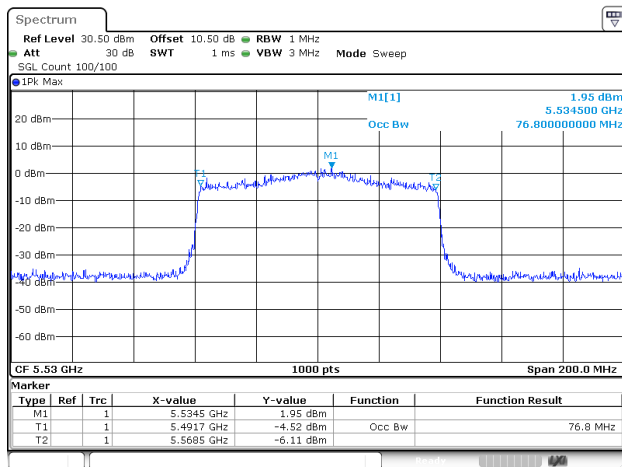
802.11ax80_5530MHz_RU_Full_ANT1
