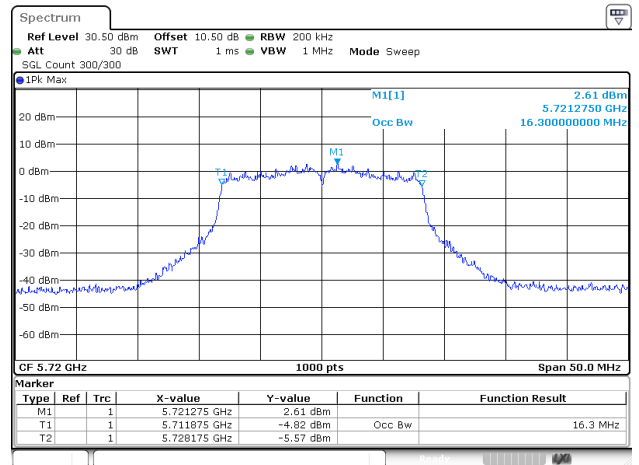
802.11a_5720MHz_ANT2
