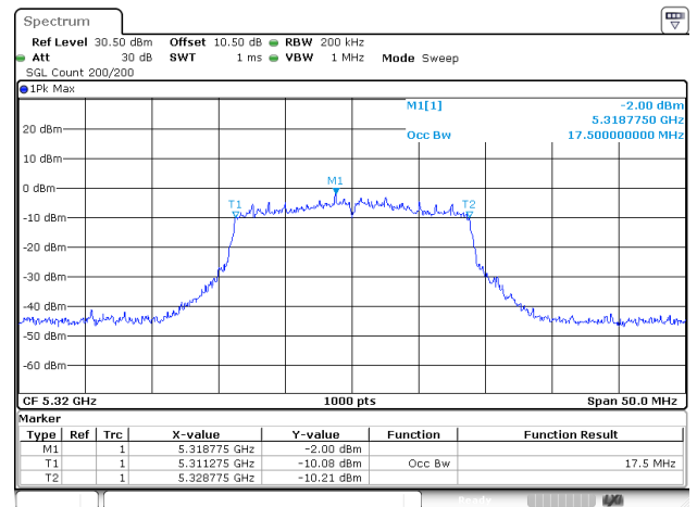
802.11ac20_5320MHz_ANT2
