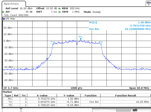
802.11a_5700MHz_ANT1
