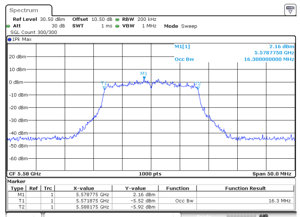
802.11a_5580MHz_ANT1
