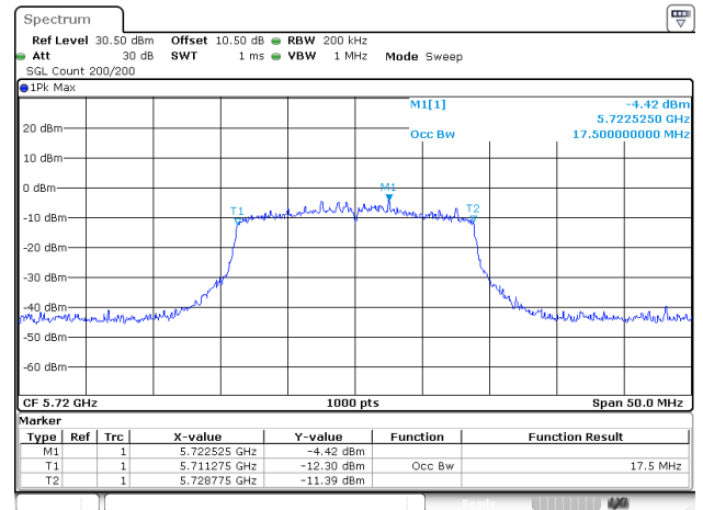
802.11ac20_5720MHz_ANT2
