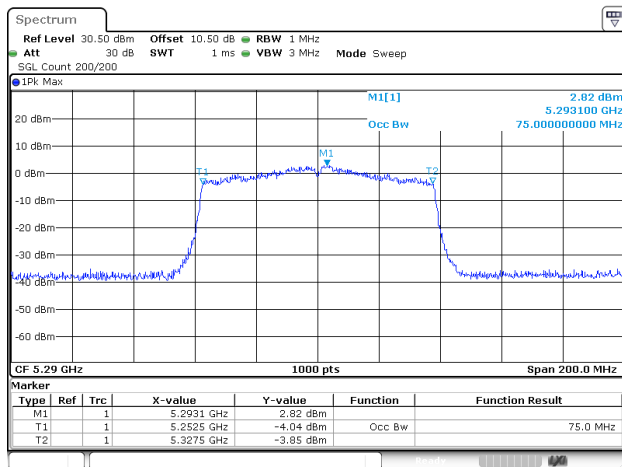
802.11ac80_5290MHz_ANT1
