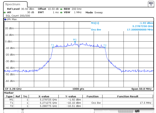
802.11ac20_5280MHz_ANT1
