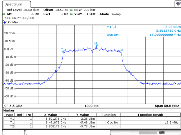
802.11a_5500MHz_ANT2
