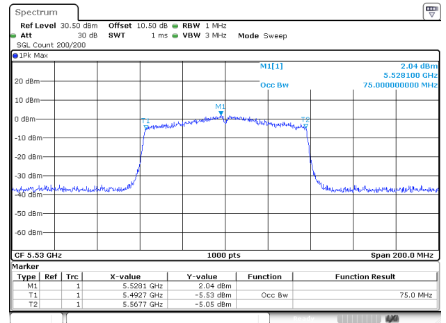
802.11ac80_5530MHz_ANT2
