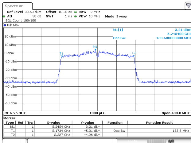
802.11ac160_5250MHz_ANT1
