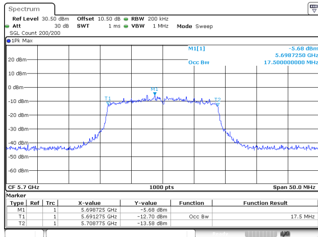
802.11ac20_5700MHz_ANT2
