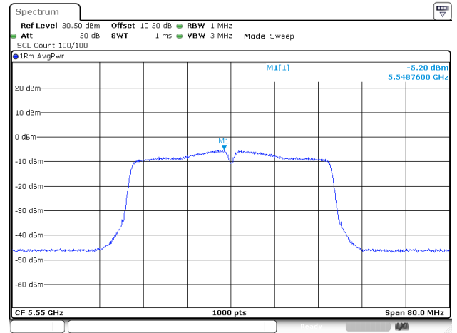
802.11ac40_5550MHz_ANT1
