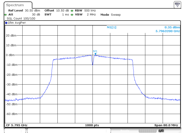
802.11ac40_5795MHz_ANT1
