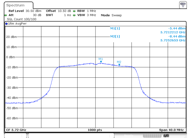
802.11ac20_5720MHz_ANT2
