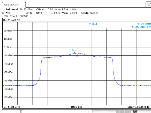
802.11ac80_5530MHz_ANT1
