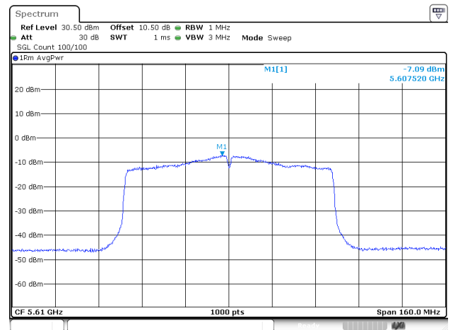
802.11ac80_5610MHz_ANT1
