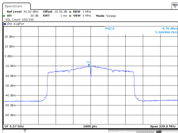
802.11ax160_5570MHz_RU_Full_ANT1
