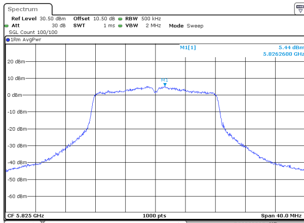
802.11a_5825MHz_ANT1
