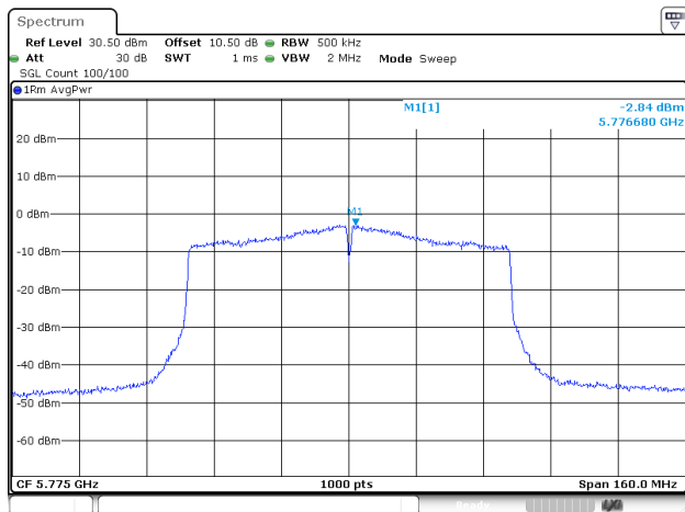
802.11ac80_5775MHz_ANT1
