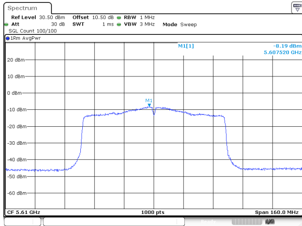
802.11ac80_5610MHz_ANT2
