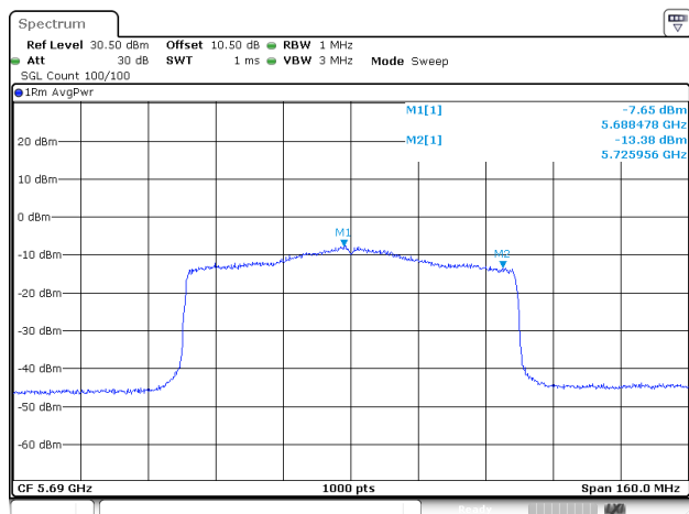
802.11ax80_5690MHz_RU_Full_ANT1
