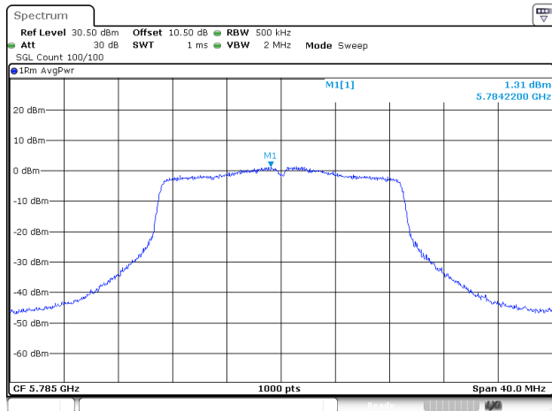
802.11ac20_5785MHz_ANT2
