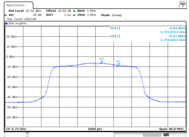
802.11ax20_5720MHz_RU_Full_ANT2
