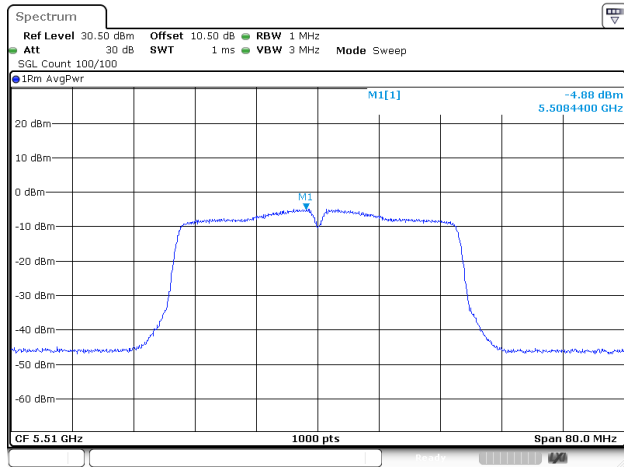
802.11ac40_5510MHz_ANT1
