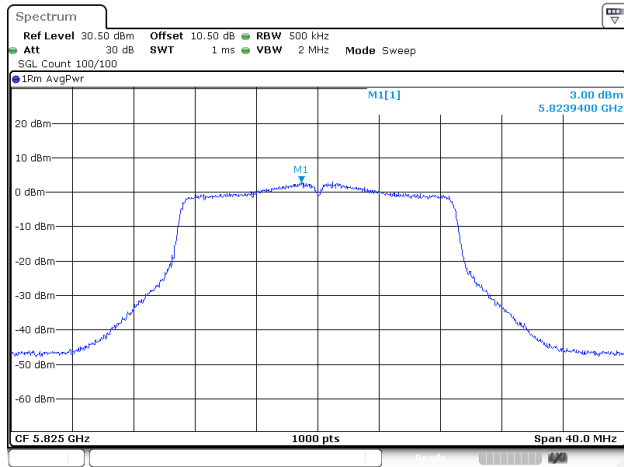
802.11ac20_5825MHz_ANT1
