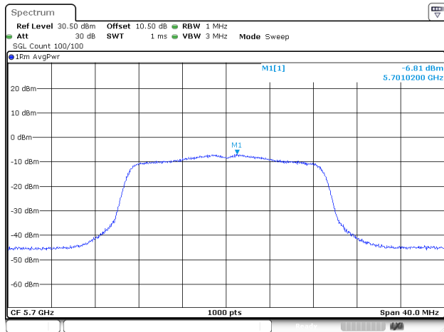
802.11ac20_5700MHz_ANT2
