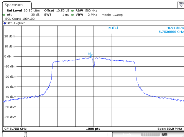
802.11ac40_5755MHz_ANT2
