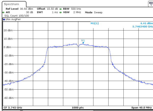
802.11a_5745MHz_ANT1
