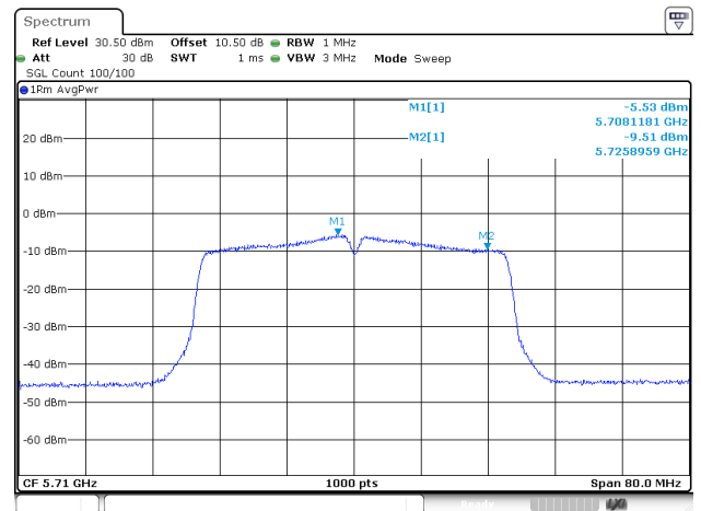
802.11ac40_5710MHz_ANT1
