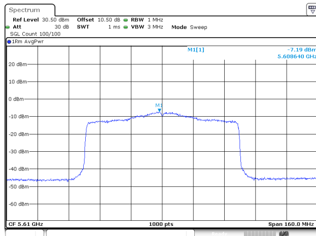
802.11ax80_5610MHz_RU_Full_ANT1
