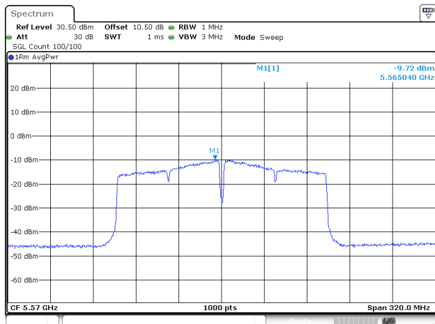
802.11ac160_5570MHz_ANT1
