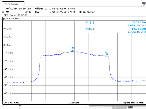
802.11ac80_5690MHz_ANT1
