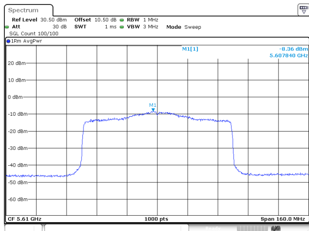
802.11ax80_5610MHz_RU_Full_ANT2
