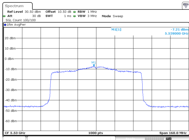
802.11ax80_5530MHz_RU_Full_ANT1
