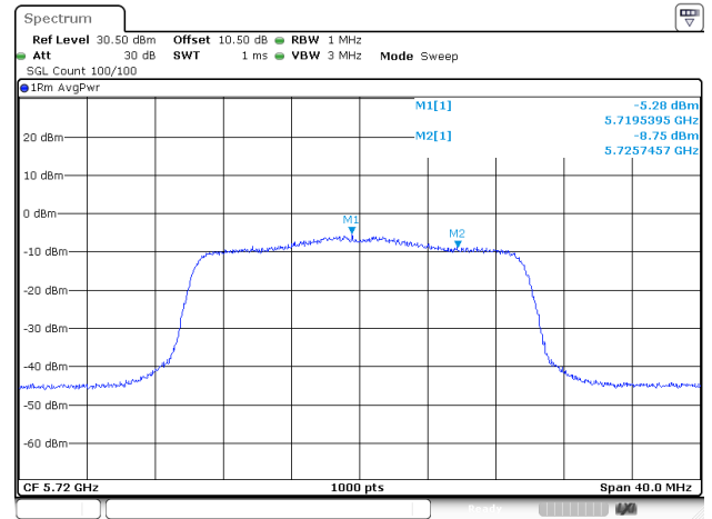
802.11ax20_5720MHz_RU_Full_ANT1
