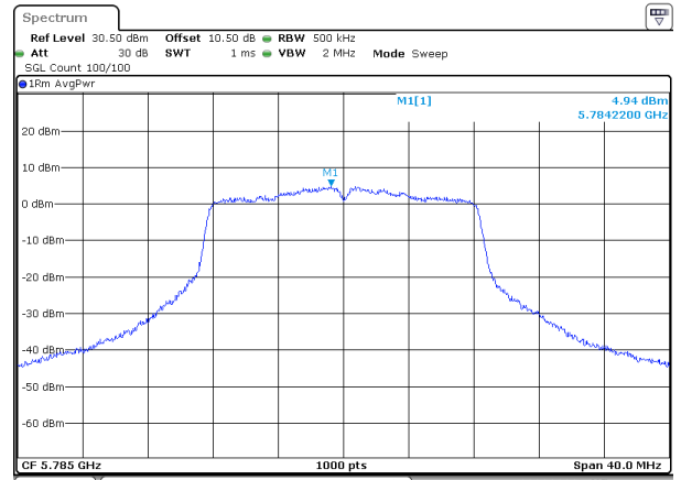
802.11a_5785MHz_ANT1
