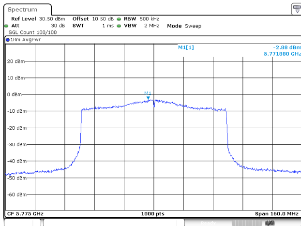
802.11ax80_5775MHz_RU_Full_ANT1
