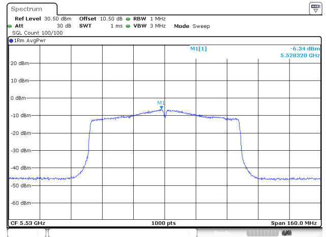
802.11ac80_5530MHz_ANT2
