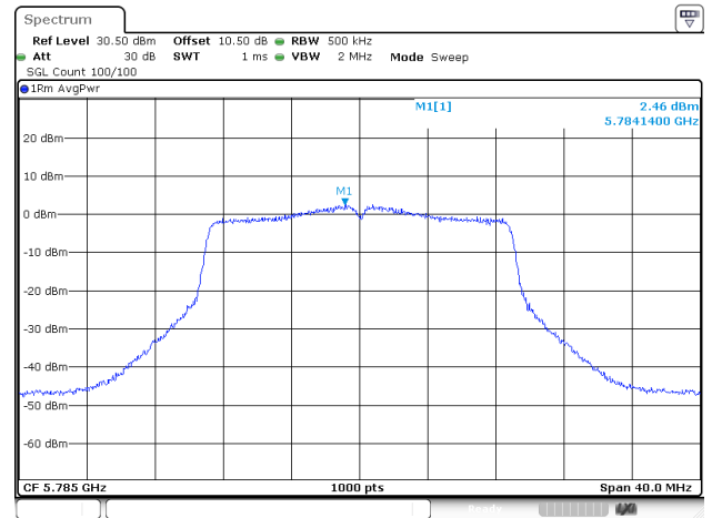
802.11ac20_5785MHz_ANT1
