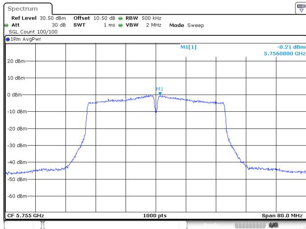
802.11ac40_5755MHz_ANT1
