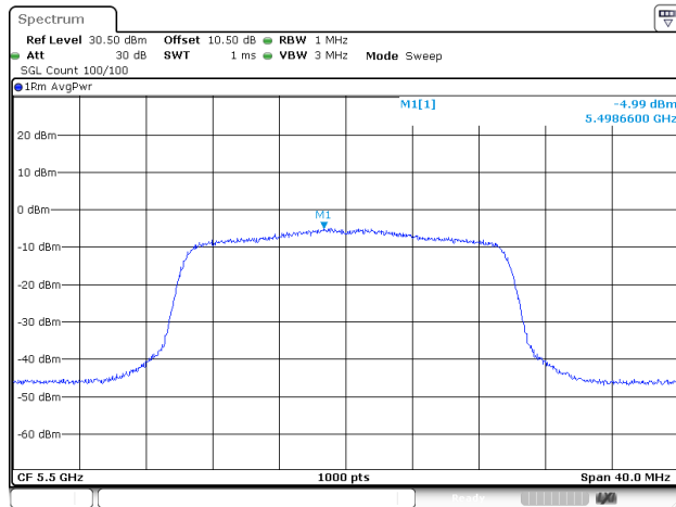
802.11ax20_5500MHz_RU_Full_ANT1
