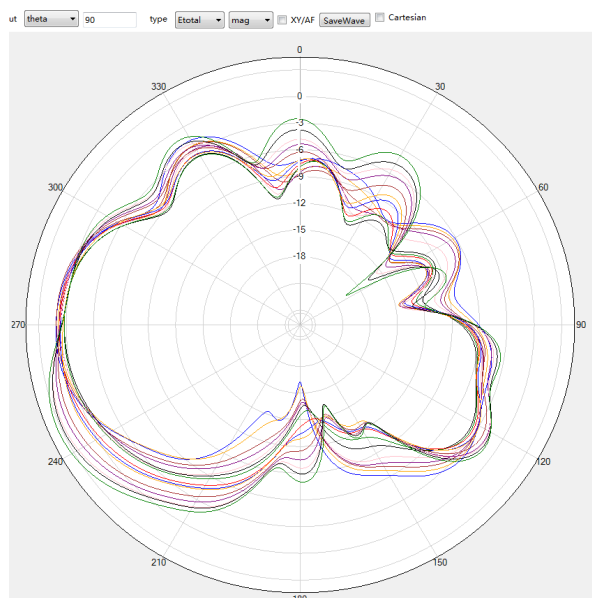
5G theta=90deg
