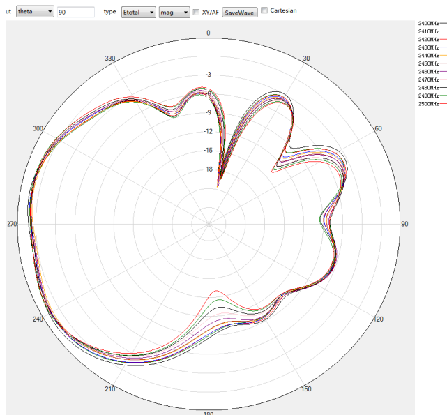
2.4G theta=90deg
