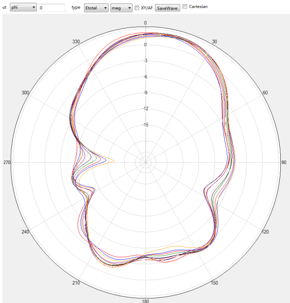
2.4G phi=0deg
