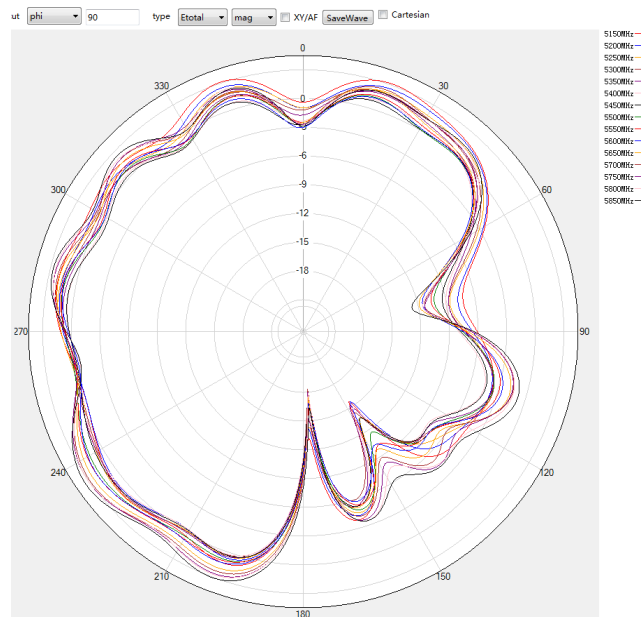
5G phi=90deg
