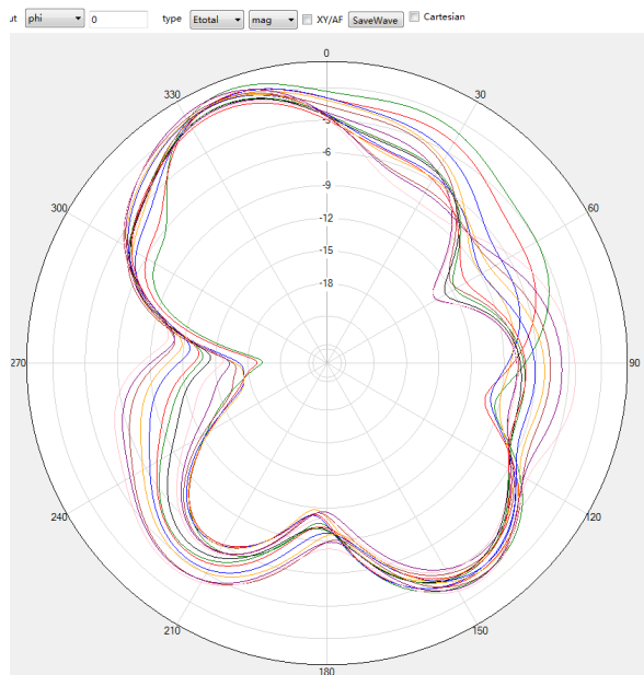
5G phi=0deg
