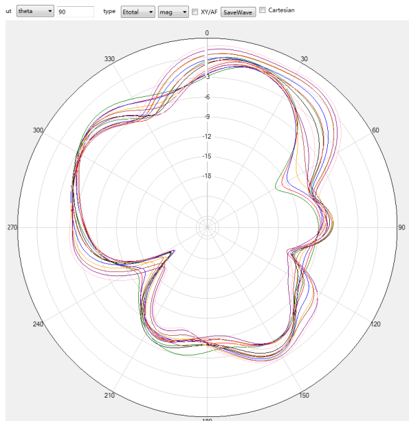
5G theta=90deg
