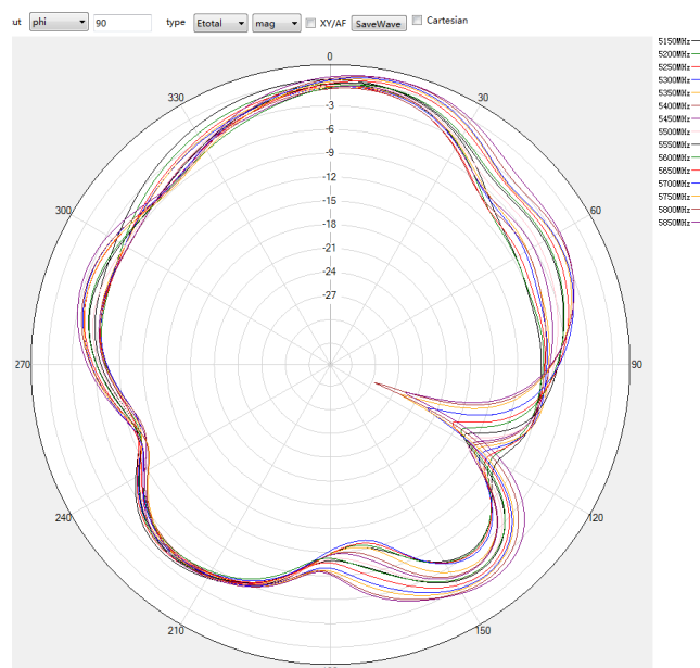
5G phi=90deg
