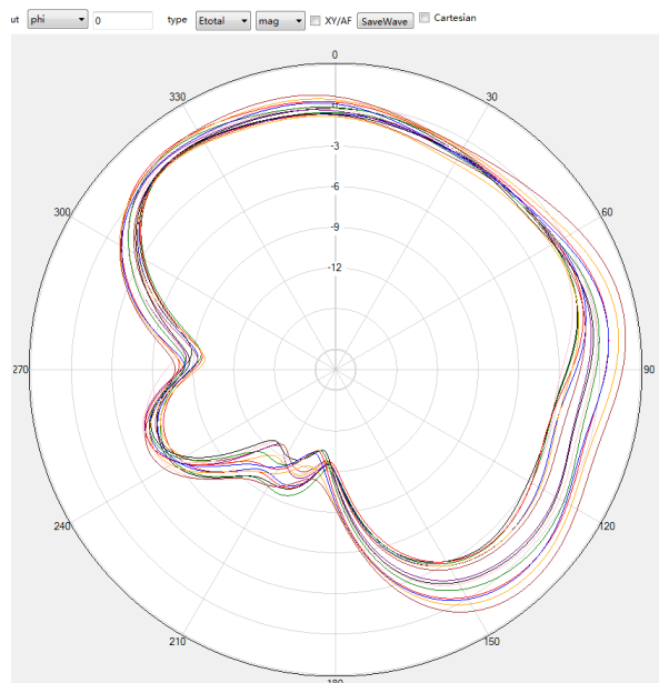
5G phi=0deg
