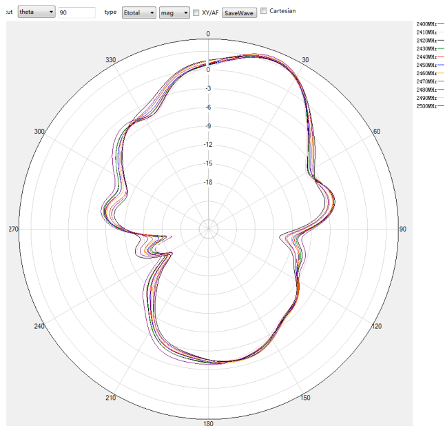
2.4G theta=90deg
