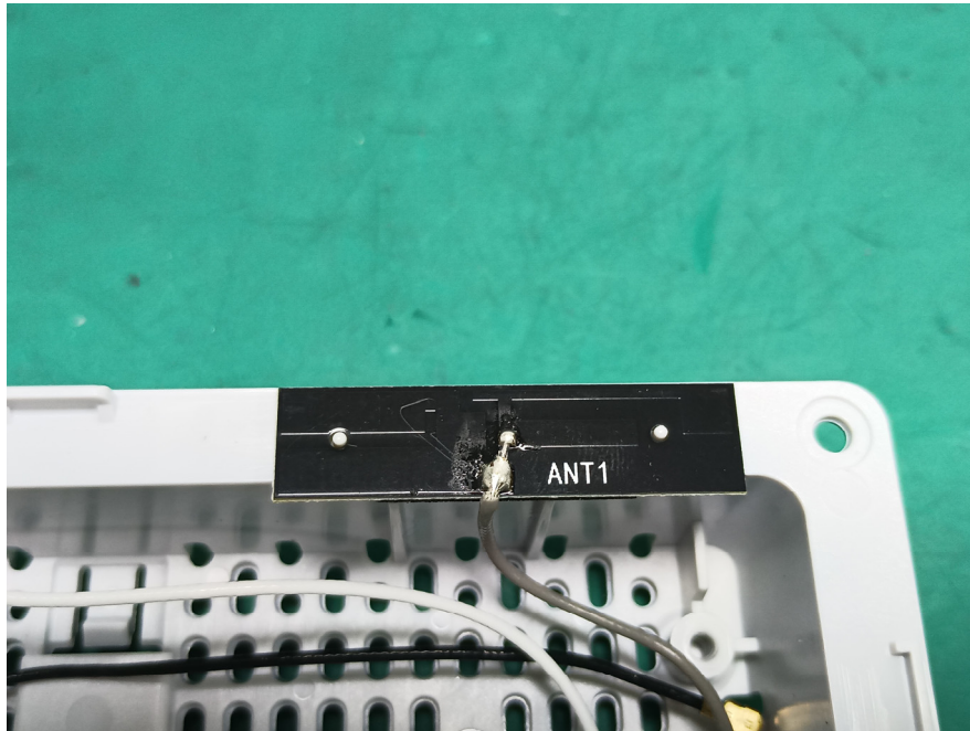
2.4G/5G ANT1
