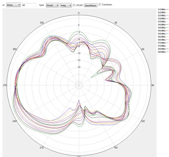
5G theta=90deg
