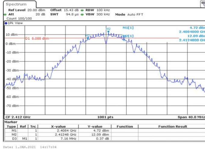
11BMIMO_Ant2_2412
