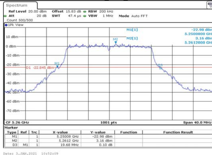
11A CDD_Ant2_5260
