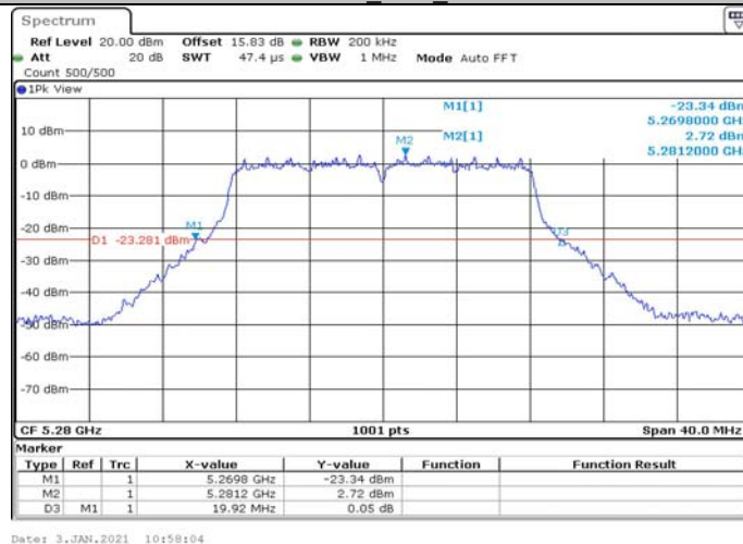
11A CDD_Ant1_5280
