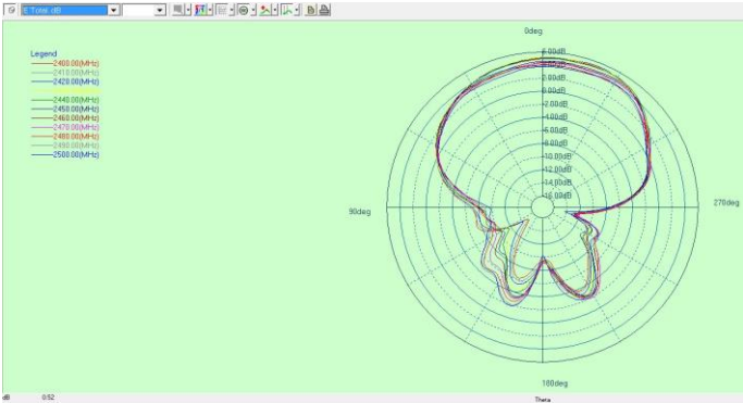
Phi=0
