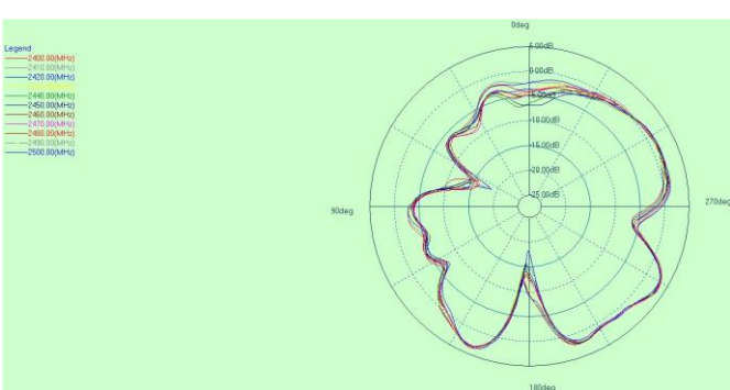
Phi=0
