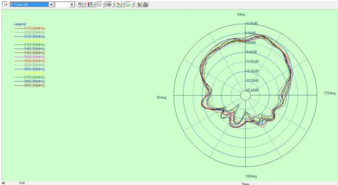
Phi=90
