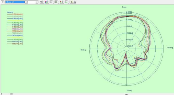
Phi=0
