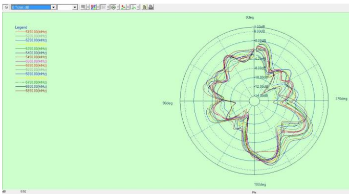
Theta=90
