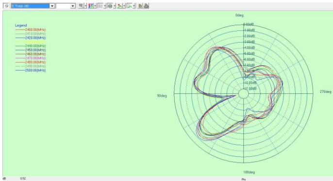
Theta=90
