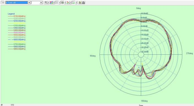
Phi=0
