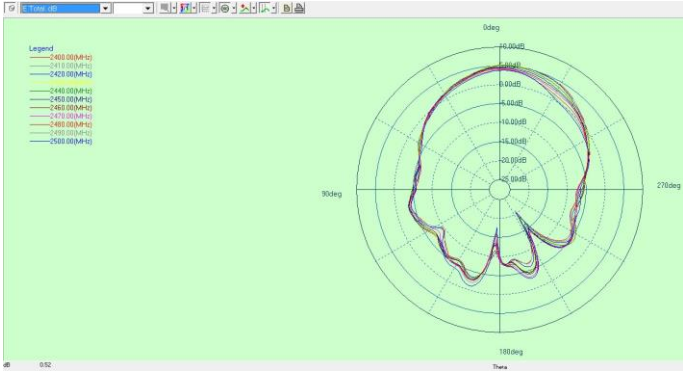
Phi=90
