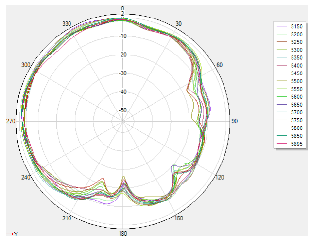
5G phi=90deg
