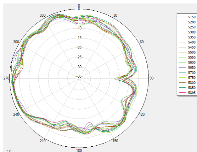
5G theta=90deg
