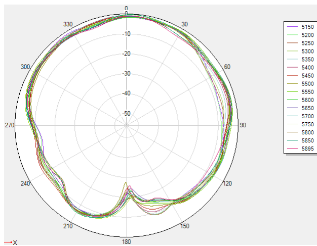
5G phi=0deg
