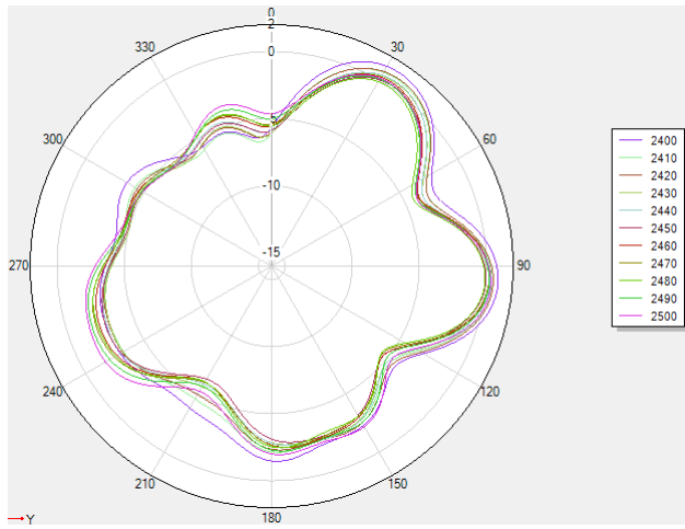
2.4G theta=90deg
