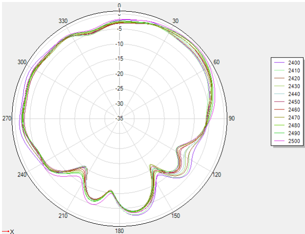
2.4G phi=0deg
