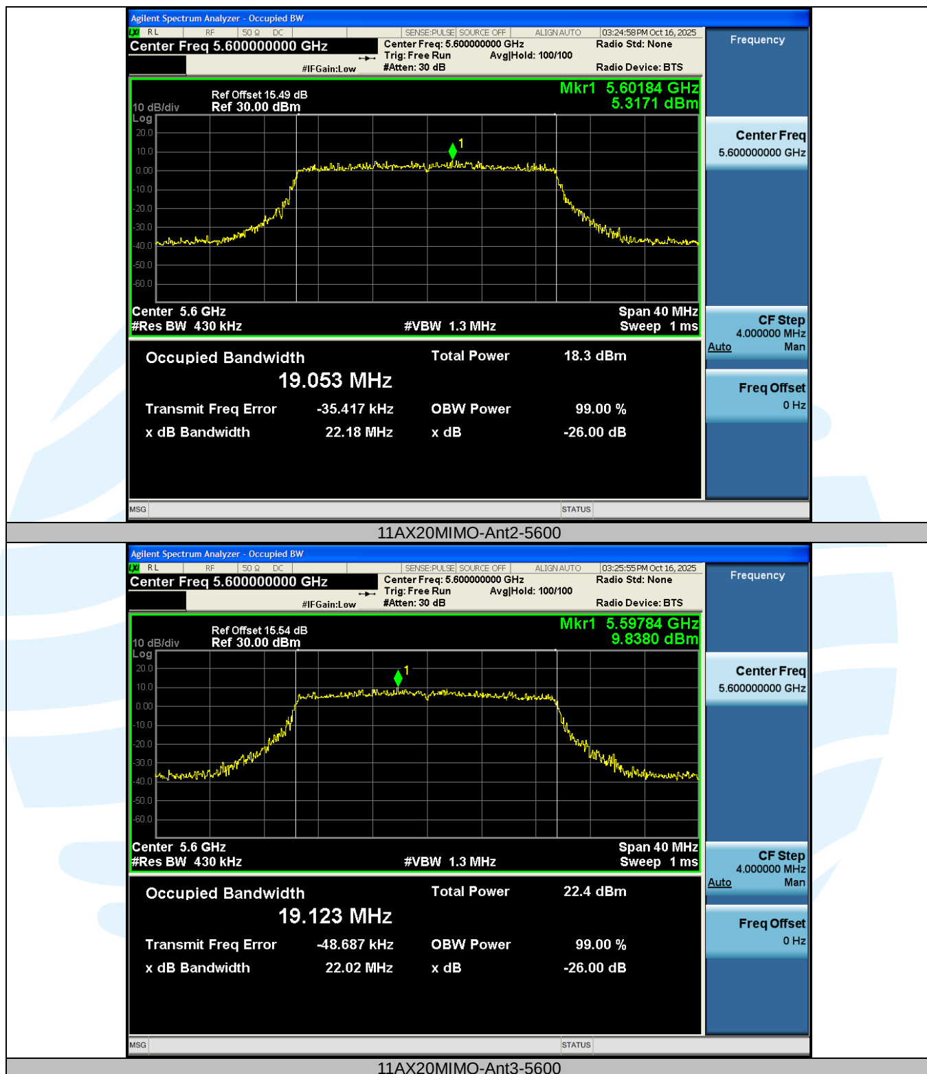
11AX20MIMO-Ant3-5600
