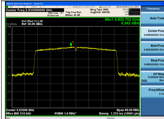
IEEE 802.11ax_Channel 167_40MHz_Antenna 3_RU&amp;Index SU
