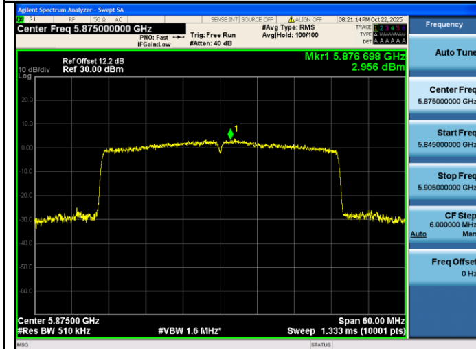
IEEE 802.11ax_Channel 175_40MHz_Antenna 1_RU&amp;Index SU
