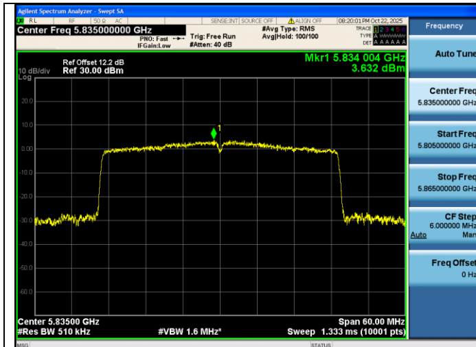
IEEE 802.11ax_Channel 167_40MHz_Antenna 1_RU&amp;Index SU
