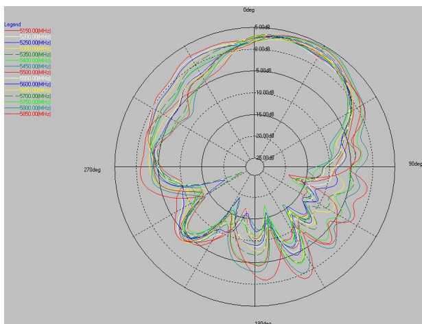
5G \phi=0^\circ
