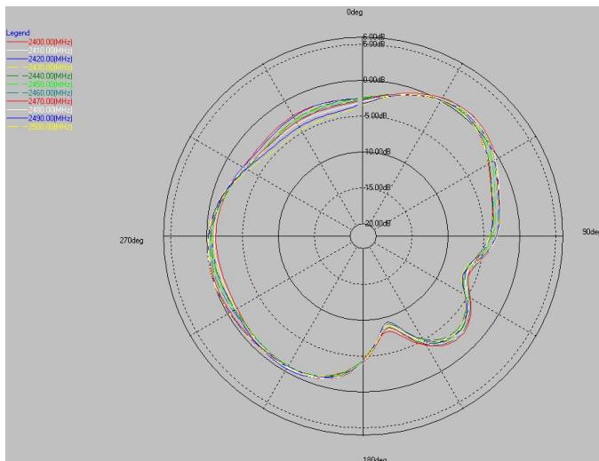
2.4G \theta=90^\circ
