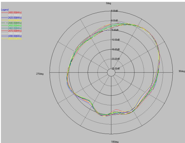
2.4G phi=0deg
