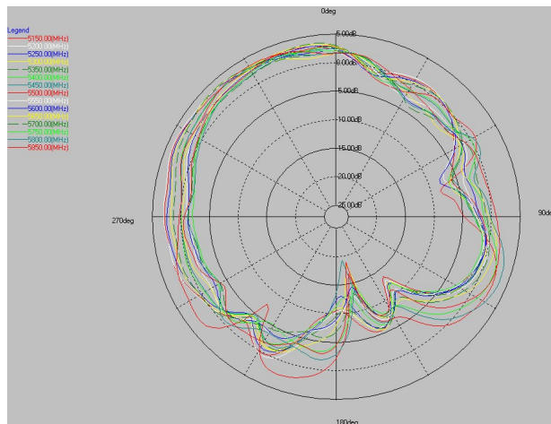
5G \phi=90^\circ
