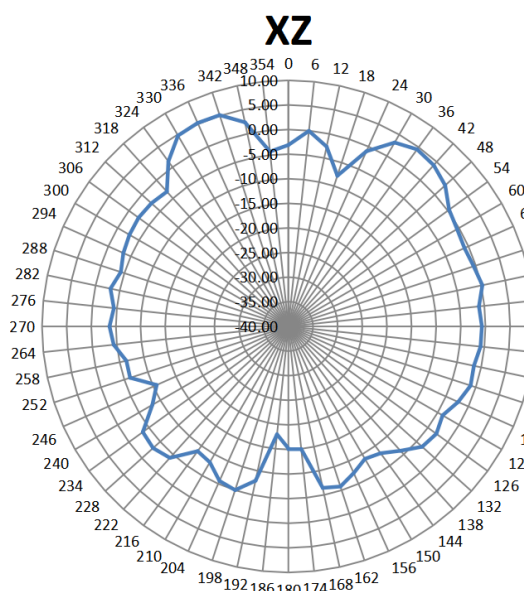
5G 辐射方向图 Radiation Patterns(unit:dB) 5G 5650MHz
