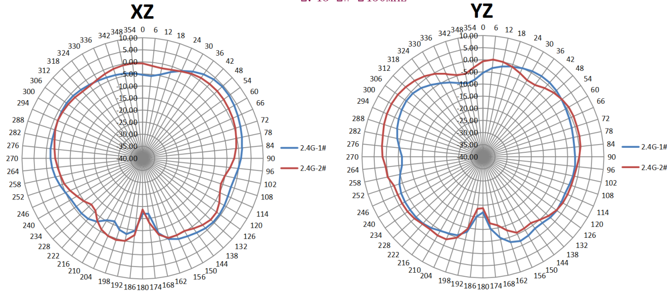
2.4G 辐射方向图 Radiation Patterns(unit:dB) 2.4G-1# 2480MHz 2.4G-2# 2450MHz
