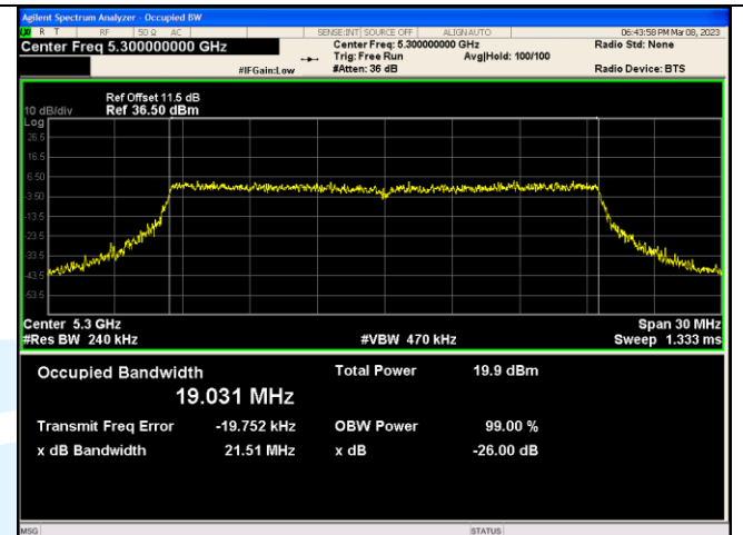
IEEE 802.11ax_Channel 60_20MHz_Antenna 3_RU&amp;Index SU
