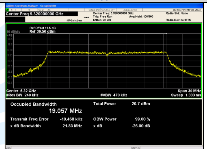
IEEE 802.11ax_Channel 64_20MHz_Antenna 3_RU&amp;Index SU
