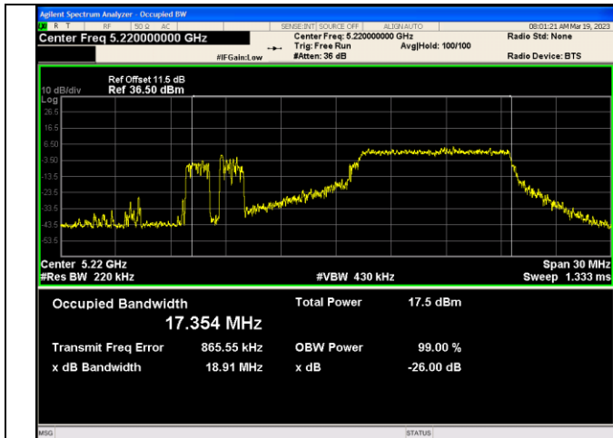
IEEE 802.11ax_Channel 44_20MHz_Antenna 0_RU&amp;Index 52RU39
