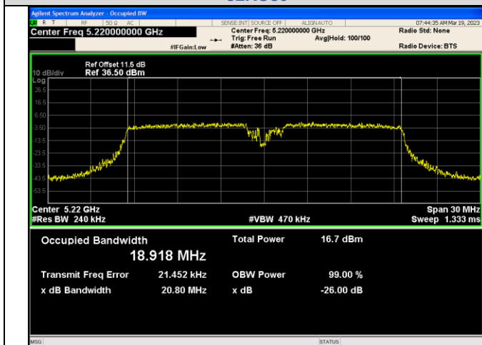
IEEE 802.11ax_Channel 44_20MHz_Antenna 0_RU&amp;Index 106RU53
