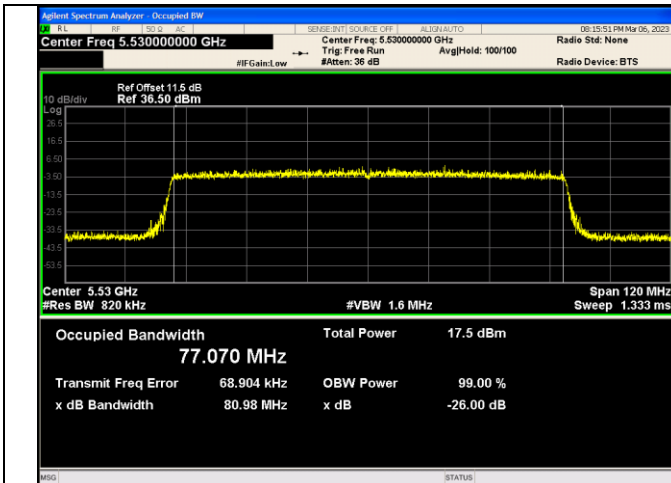
IEEE 802.11ax_Channel 106_80MHz_Antenna 0_RU&amp;Index SU
