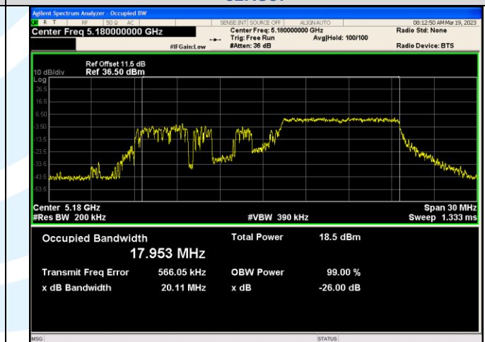
IEEE 802.11ax_Channel 36_20MHz_Antenna 1_RU&amp;Index 106RU53
