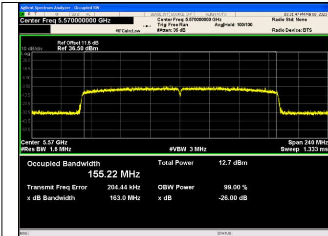
IEEE 802.11ax_Channel 114_160MHz_Antenna 2_RU&amp;Index SU
