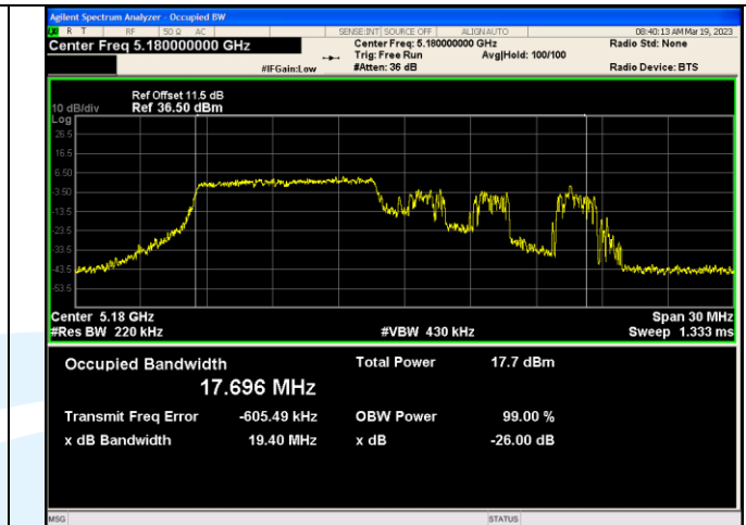
IEEE 802.11ax_Channel 36_20MHz_Antenna 1_RU&amp;Index 52RU37
