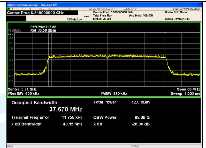
IEEE 802.11ax_Channel 102_40MHz_Antenna 3_RU&amp;Index SU
