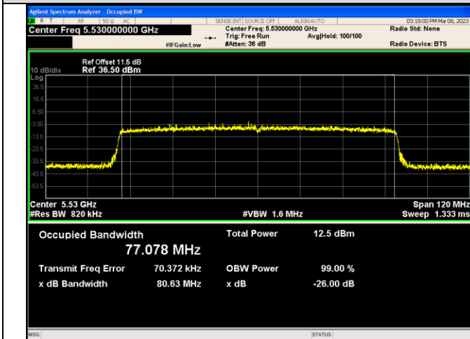
IEEE 802.11ax_Channel 106_80MHz_Antenna 2_RU&amp;Index SU
