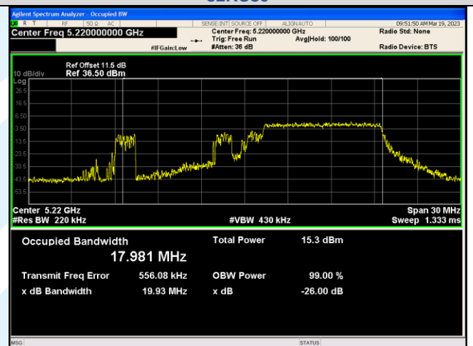
IEEE 802.11ax_Channel 44_20MHz_Antenna 3_RU&amp;Index 52RU39
