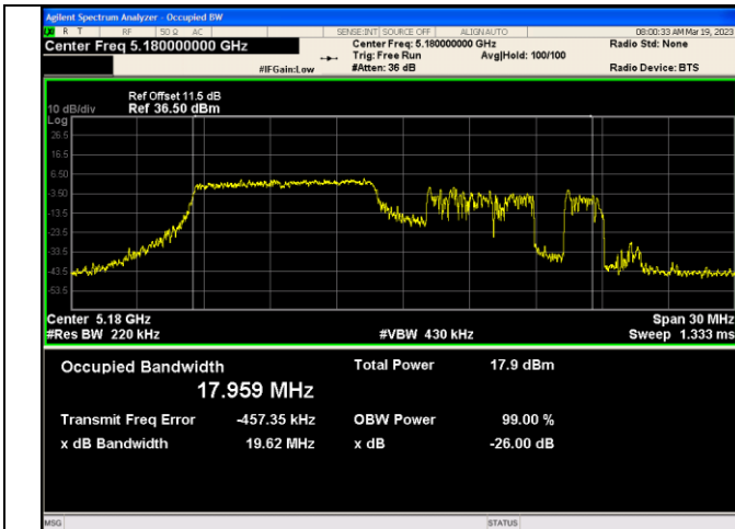
IEEE 802.11ax_Channel 36_20MHz_Antenna 0_RU&amp;Index 52RU37
