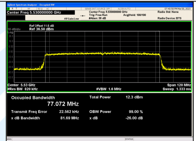
IEEE 802.11ax_Channel 106_80MHz_Antenna 3_RU&amp;Index SU
