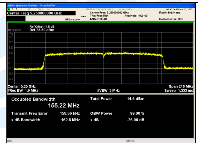
IEEE 802.11ax_Channel 50_80+80MHz_Antenna 1_RU&amp;Index SU
