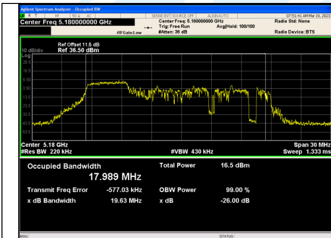
IEEE 802.11ax_Channel 36_20MHz_Antenna 0_RU&amp;Index 26RU0
