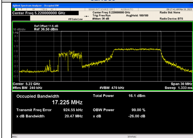
IEEE 802.11ax_Channel 44_20MHz_Antenna 2_RU&amp;Index 52RU39
