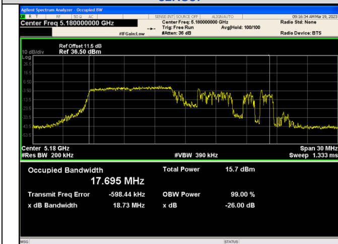
IEEE 802.11ax_Channel 36_20MHz_Antenna 2_RU&amp;Index 52RU37
