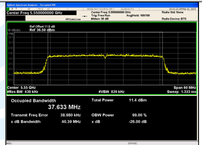
IEEE 802.11ax_Channel 110_40MHz_Antenna 3_RU&amp;Index SU
