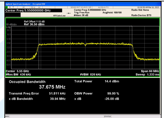
IEEE 802.11ax_Channel 110_40MHz_Antenna 1_RU&amp;Index SU
