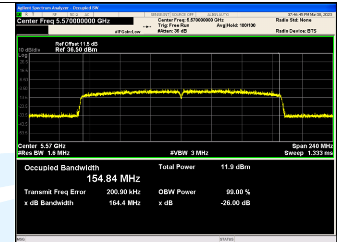
IEEE 802.11ax_Channel 114_160MHz_Antenna 3_RU&amp;Index SU
