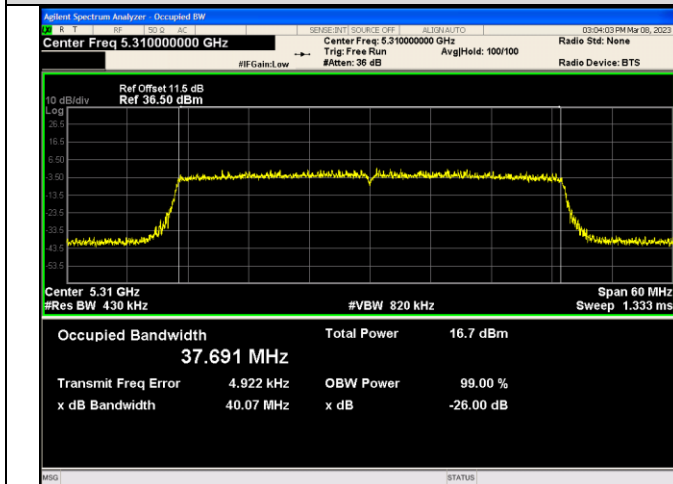
IEEE 802.11ax_Channel 62_40MHz_Antenna 2_RU&amp;Index SU
