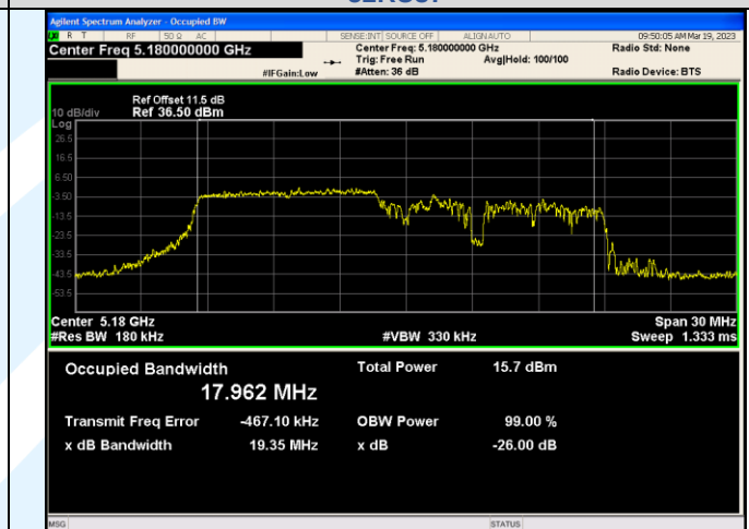
IEEE 802.11ax_Channel 36_20MHz_Antenna 3_RU&amp;Index 52RU37
