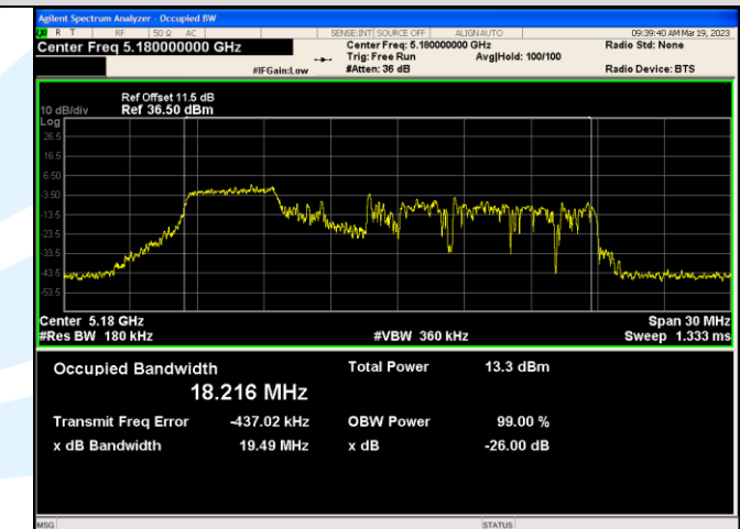
IEEE 802.11ax_Channel 36_20MHz_Antenna 3_RU&amp;Index 26RU0
