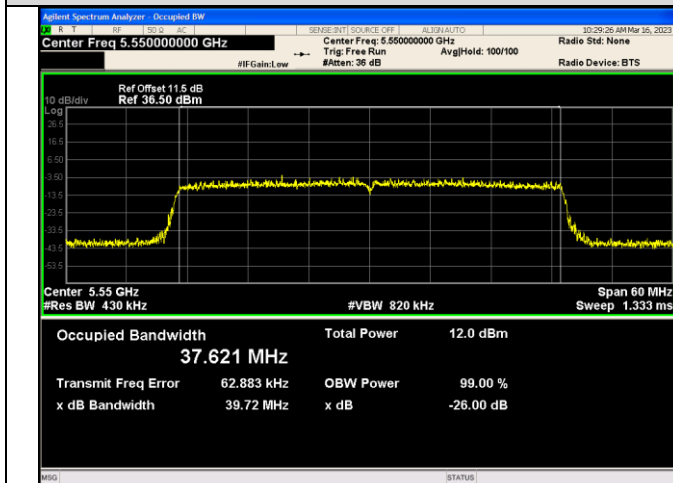
IEEE 802.11ax_Channel 110_40MHz_Antenna 2_RU&amp;Index SU
