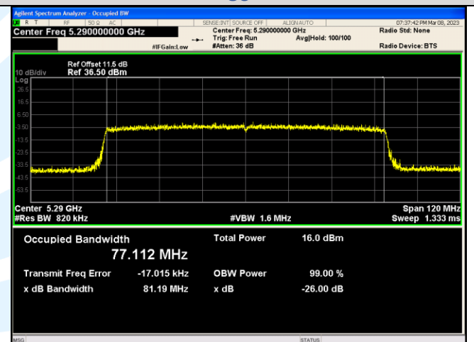
IEEE 802.11ax_Channel 58_80MHz_Antenna 3_RU&Index SU
