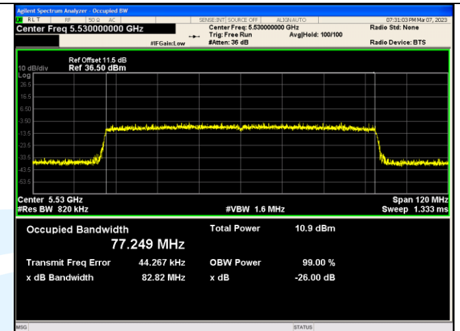
IEEE 802.11ax_Channel 106_80MHz_Antenna 1_RU&amp;Index SU
