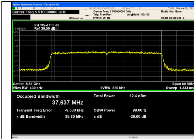
IEEE 802.11ax_Channel 102_40MHz_Antenna 2_RU&amp;Index SU
