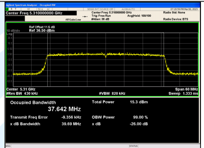
IEEE 802.11ax_Channel 62_40MHz_Antenna 3_RU&amp;Index SU
