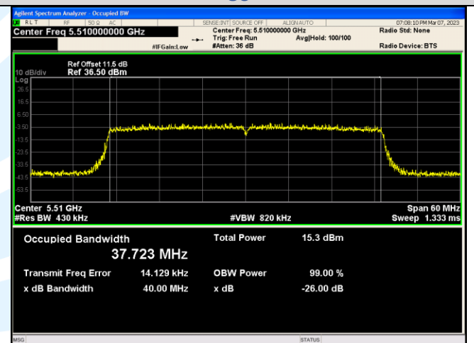
IEEE 802.11ax_Channel 102_40MHz_Antenna 1_RU&amp;Index SU
