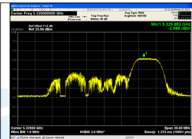
IEEE 802.11ax_Channel 64_20MHz_Antenna 3_RU&Index 26RU8
