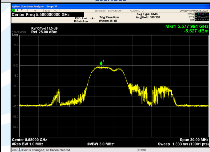
IEEE 802.11ax_Channel 116_20MHz_Antenna 1_RU&amp;Index 26RU4
