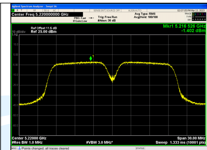
IEEE 802.11ax_Channel 44_20MHz_Antenna 1_RU&Index 106RU53
