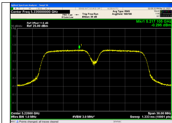
IEEE 802.11ax_Channel 44_20MHz_Antenna 0_RU&Index 106RU53
