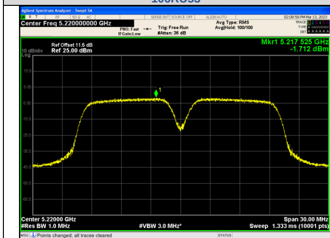
IEEE 802.11ax_Channel 44_20MHz_Antenna 2_RU&Index 106RU53
