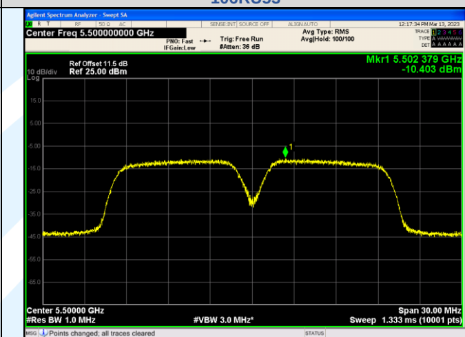
IEEE 802.11ax_Channel 100_20MHz_Antenna 3_RU&amp;Index 106RU53
