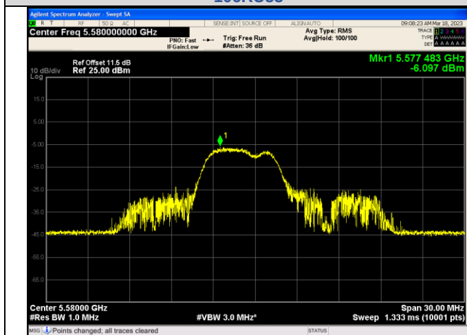
IEEE 802.11ax_Channel 116_20MHz_Antenna 0_RU&amp;Index 26RU4
