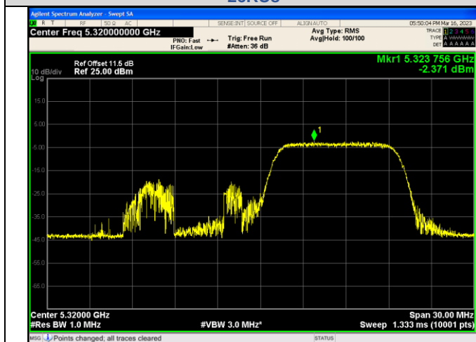
IEEE 802.11ax_Channel 64_20MHz_Antenna 0_RU&Index 52RU40
