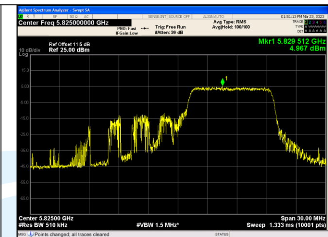
IEEE 802.11ax_Channel 165_20MHz_Antenna 3_RU&Index 52RU40
