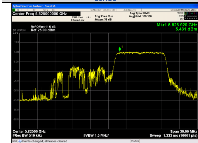
IEEE 802.11ax_Channel 165_20MHz_Antenna 0_RU&amp;Index 52RU40
