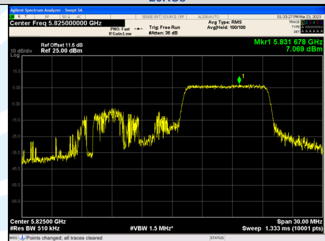
IEEE 802.11ax_Channel 165_20MHz_Antenna 1_RU&amp;Index 52RU40
