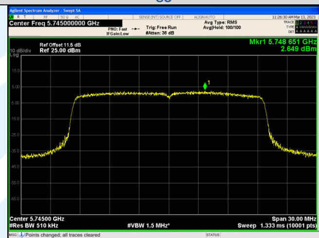
IEEE 802.11ax_Channel 149_20MHz_Antenna 3_RU&Index SU
