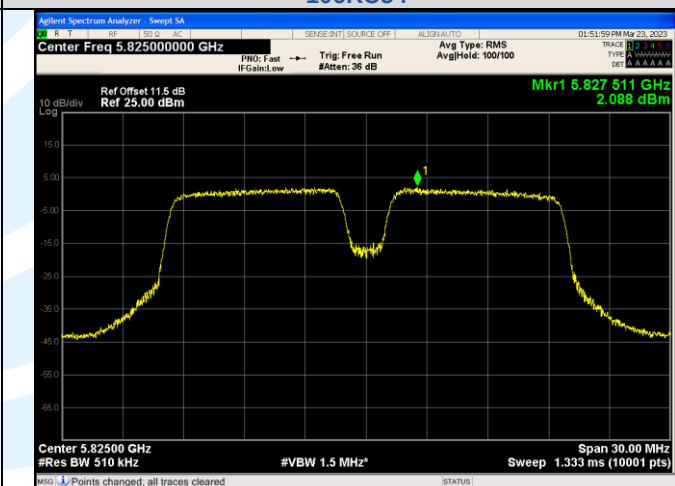
IEEE 802.11ax_Channel 165_20MHz_Antenna 3_RU&Index 106RU54
