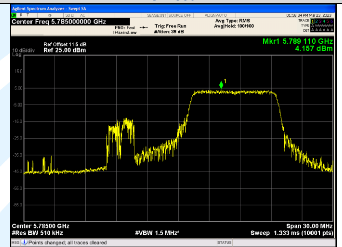
IEEE 802.11ax_Channel 157_20MHz_Antenna 3_RU&amp;Index 52RU39
