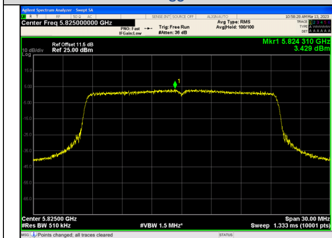
IEEE 802.11ax_Channel 165_20MHz_Antenna 2_RU&Index SU
