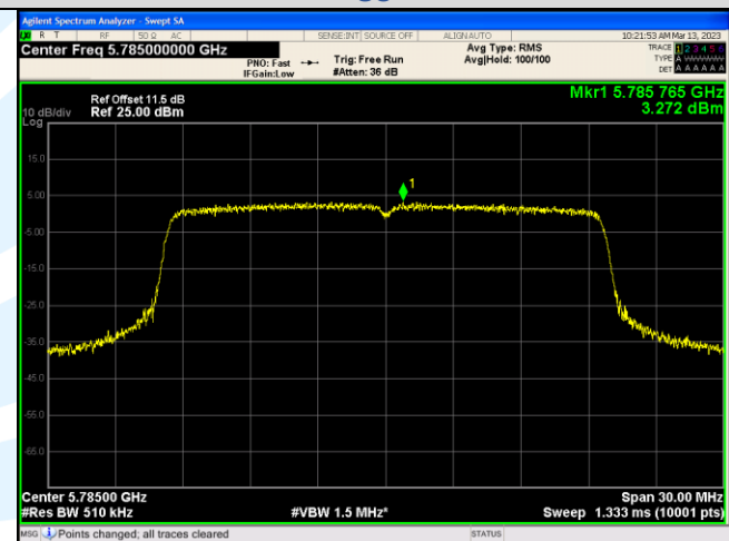
IEEE 802.11ax_Channel 157_20MHz_Antenna 1_RU&Index SU
