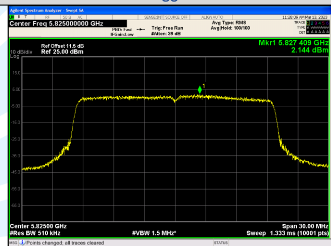
IEEE 802.11ax_Channel 165_20MHz_Antenna 3_RU&Index SU
