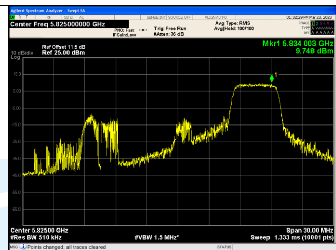
IEEE 802.11ax_Channel 165_20MHz_Antenna 1_RU&amp;Index 26RU8
