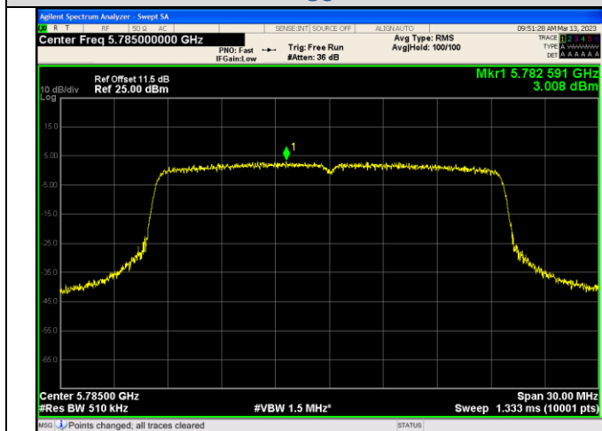
IEEE 802.11ax_Channel 157_20MHz_Antenna 0_RU&Index SU
