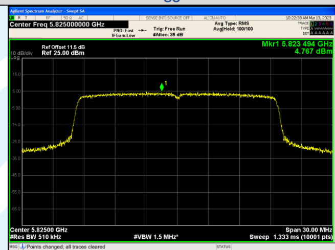
IEEE 802.11ax_Channel 165_20MHz_Antenna 1_RU&Index SU
