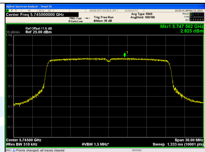
IEEE 802.11ax_Channel 149_20MHz_Antenna 1_RU&Index SU
