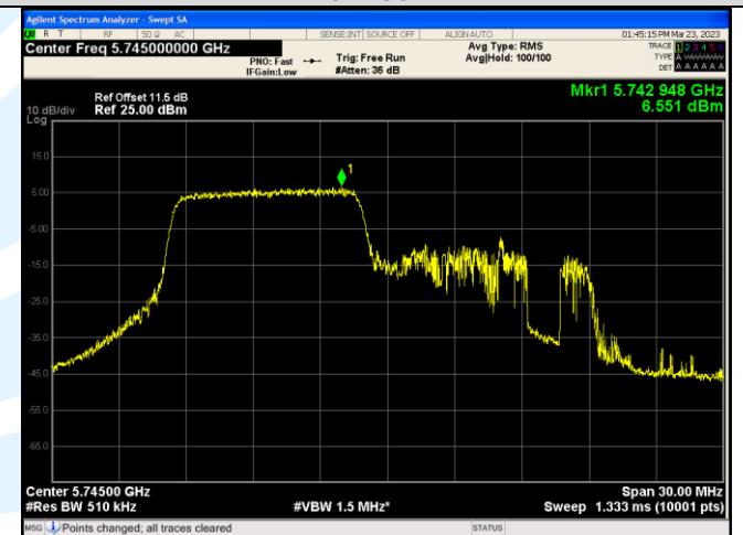
IEEE 802.11ax_Channel 149_20MHz_Antenna 3_RU&amp;Index 52RU37
