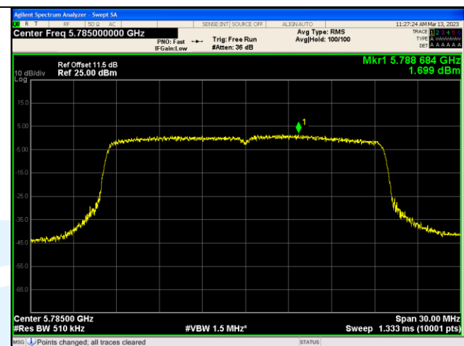
IEEE 802.11ax_Channel 157_20MHz_Antenna 3_RU&Index SU
