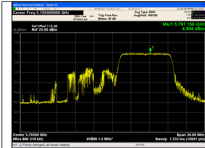
IEEE 802.11ax_Channel 157_20MHz_Antenna 0_RU&amp;Index 52RU39
