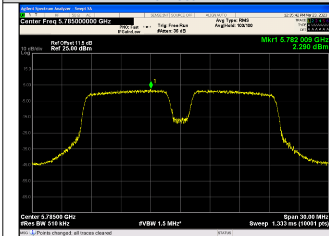
IEEE 802.11ax_Channel 157_20MHz_Antenna 0_RU&amp;Index 106RU53
