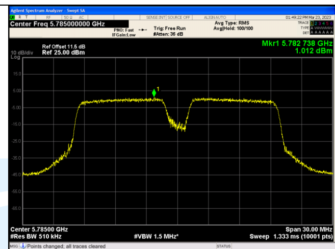
IEEE 802.11ax_Channel 157_20MHz_Antenna 3_RU&Index 106RU53
