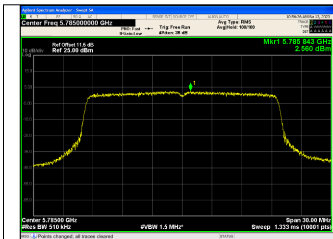
IEEE 802.11ax_Channel 157_20MHz_Antenna 2_RU&Index SU
