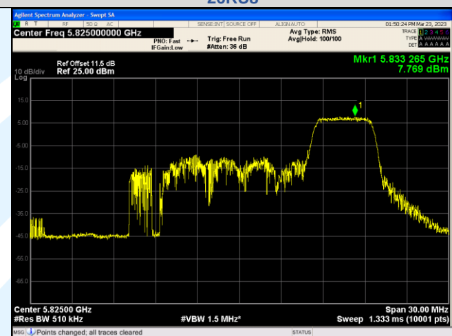
IEEE 802.11ax_Channel 165_20MHz_Antenna 3_RU&amp;Index 26RU8
