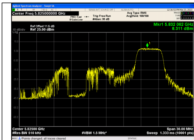
IEEE 802.11ax_Channel 165_20MHz_Antenna 0_RU&amp;Index 26RU8
