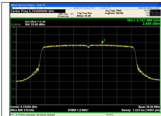
IEEE 802.11ax_Channel 149_20MHz_Antenna 0_RU&Index SU
