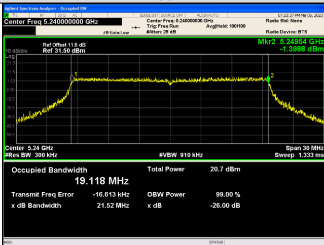
IEEE 802.11ax_Channel 48_20MHz_Antenna 0_RU&amp;Index SU
