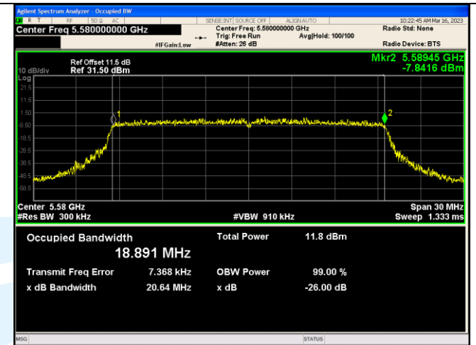
IEEE 802.11ax_Channel 116_20MHz_Antenna 3_RU&amp;Index SU
