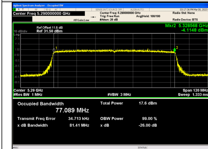
IEEE 802.11ax_Channel 58_80MHz_Antenna 2_RU&amp;Index SU
