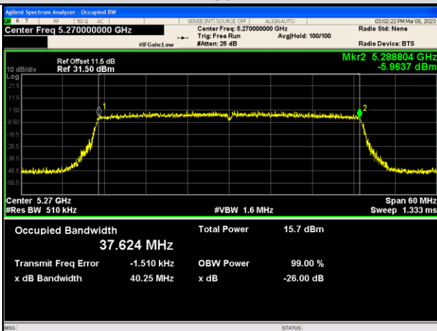
IEEE 802.11ax_Channel 54_40MHz_Antenna 2_RU&amp;Index SU
