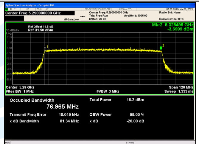
IEEE 802.11ax_Channel 58_80MHz_Antenna 3_RU&amp;Index SU
