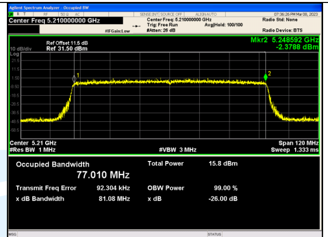
IEEE 802.11ax_Channel 42_80MHz_Antenna 3_RU&amp;Index SU
