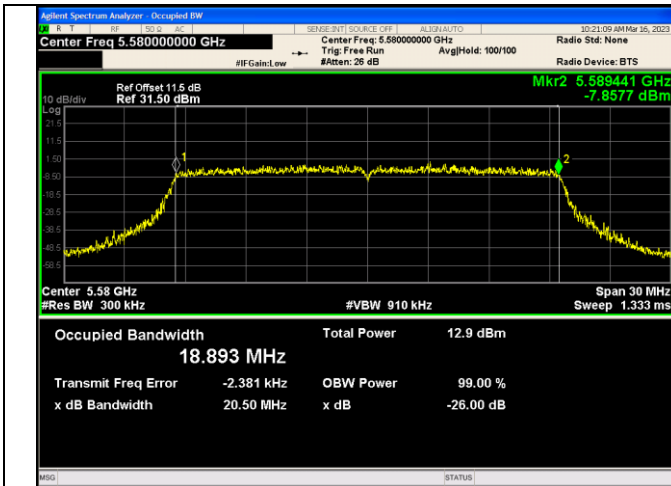
IEEE 802.11ax_Channel 116_20MHz_Antenna 2_RU&amp;Index SU
