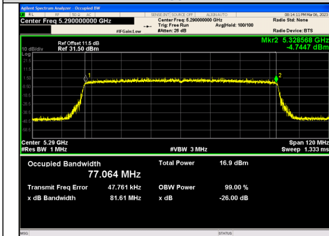
IEEE 802.11ax_Channel 58_80MHz_Antenna 0_RU&amp;Index SU
