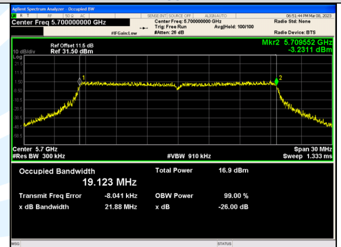
IEEE 802.11ax_Channel 140_20MHz_Antenna 3_RU&amp;Index SU
