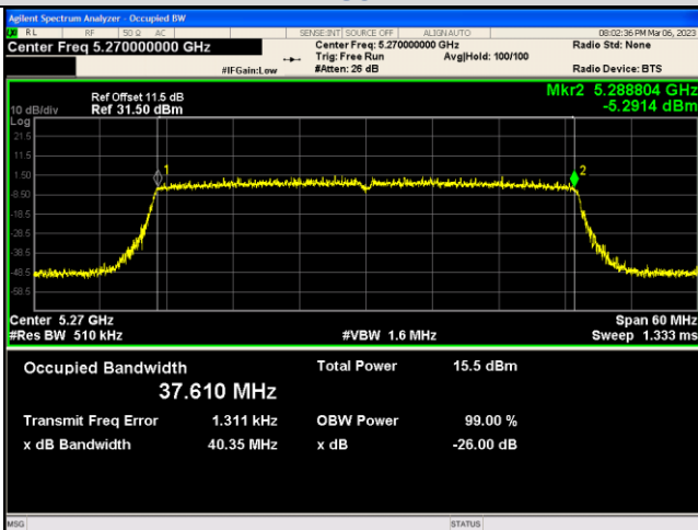
IEEE 802.11ax_Channel 54_40MHz_Antenna 0_RU&amp;Index SU
