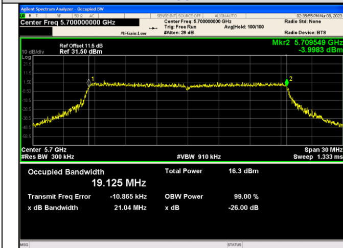
IEEE 802.11ax_Channel 140_20MHz_Antenna 2_RU&amp;Index SU
