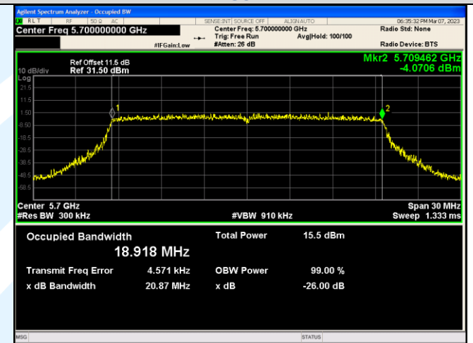
IEEE 802.11ax_Channel 140_20MHz_Antenna 1_RU&amp;Index SU
