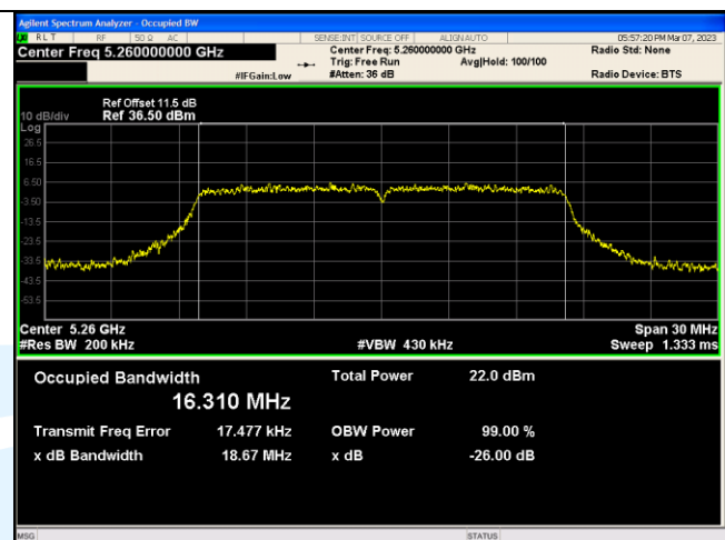
IEEE 802.11a_Channel 52_20MHz_Antenna 1
