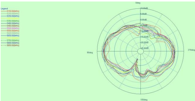
theta=90deg
