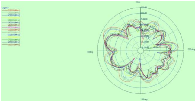
phi=0deg
