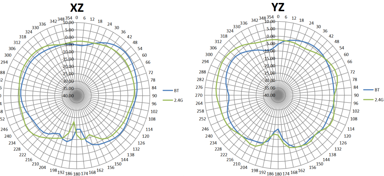
BT/2.4G 辐射方向图 Radiation Patterns(unit:dB)
