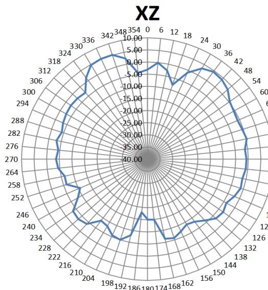
5G 辐射方向图 Radiation Patterns(unit:dB)
