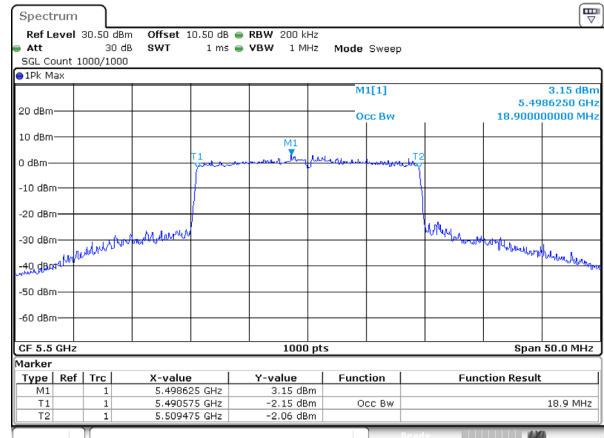
802.11be20_5500MHz_RU_FULL_Ant 1
