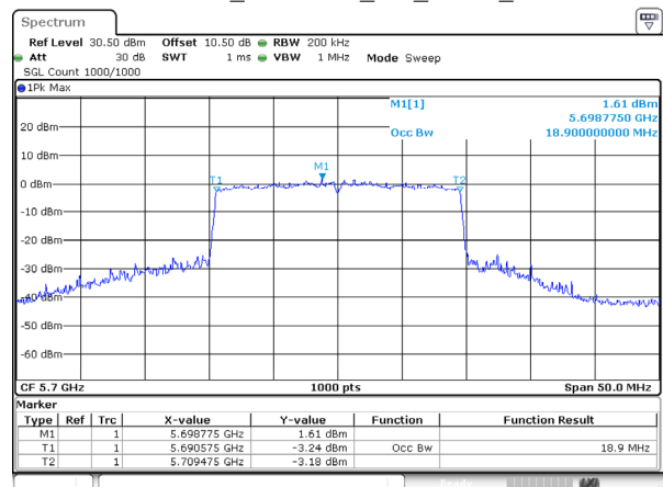
802.11be20_5700MHz_RU_FULL_Ant 0
