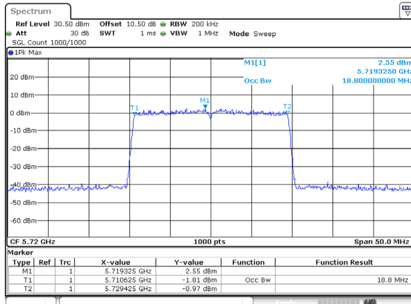
802.11ax20_5720MHz_RU_FULL_Ant 0
