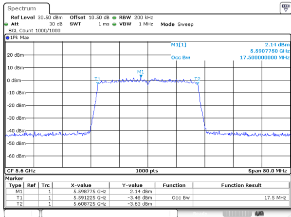
802.11ac20_5600MHz_Ant 1
