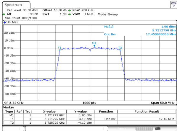
802.11ac20_5720MHz_Ant 0
