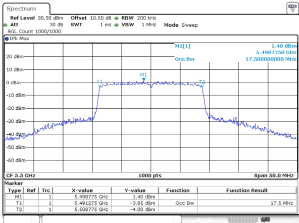
802.11ac20_5500MHz_Ant 2
