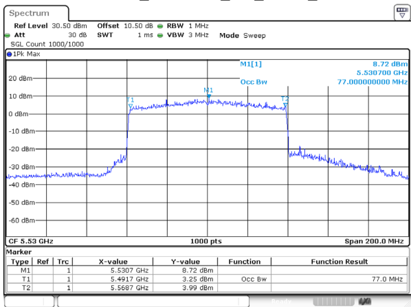
802.11ax80_5530MHz_RU_FULL_Ant 1
