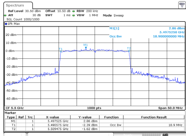
802.11be20_5500MHz_RU_FULL_Ant 0
