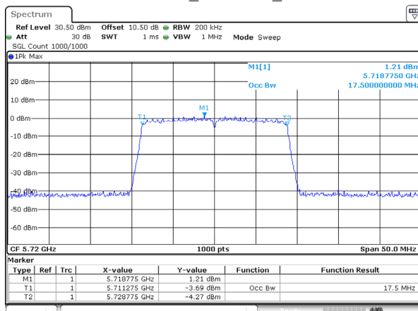
802.11ac20_5720MHz_Ant 2
