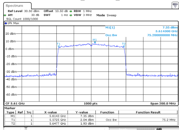
802.11ac80_5610MHz_Ant 1
