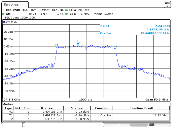
802.11ac20_5500MHz_Ant 1
