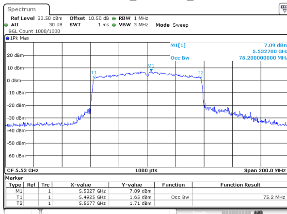
802.11ac80_5530MHz_Ant 1
