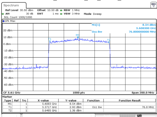
802.11ax80_5610MHz_RU_FULL_Ant 2
