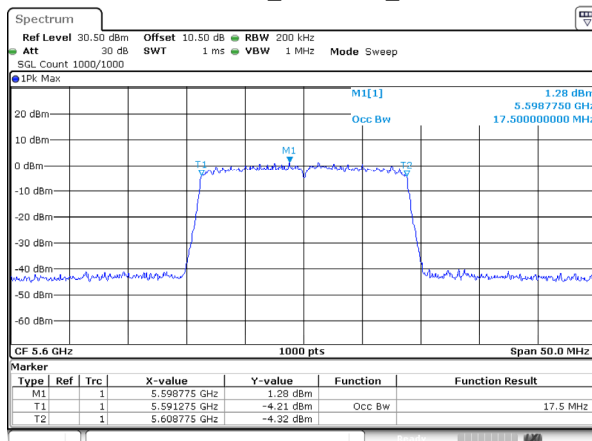
802.11ac20_5600MHz_Ant 2
