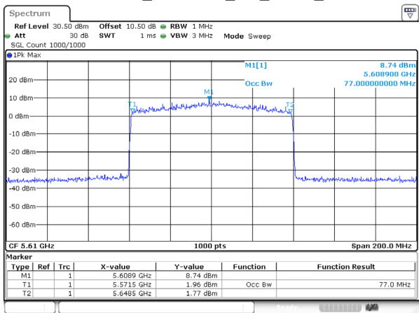
802.11ax80_5610MHz_RU_FULL_Ant 1
