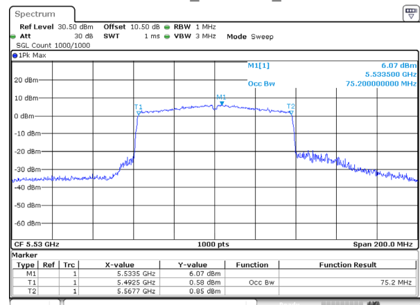
802.11ac80_5530MHz_Ant 0
