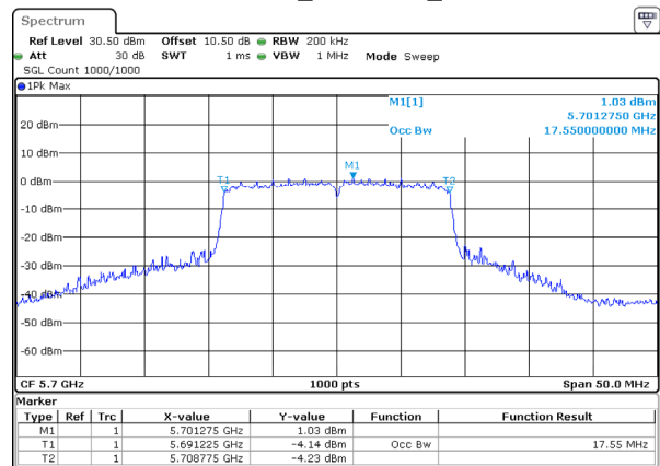
802.11ac20_5700MHz_Ant 2
