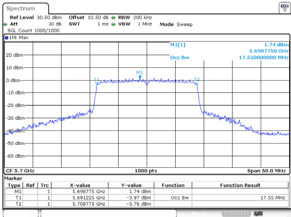
802.11ac20_5700MHz_Ant 1
