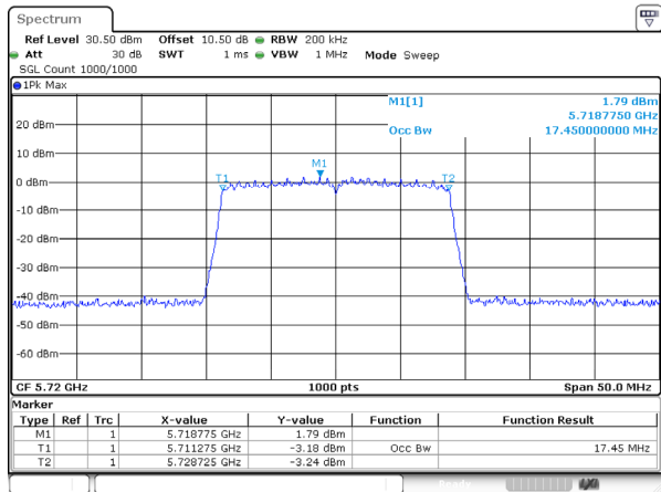
802.11ac20_5720MHz_Ant 1
