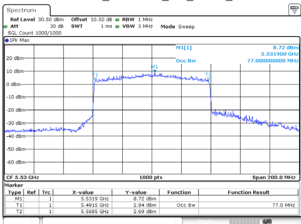
802.11ax80_5530MHz_RU_FULL_Ant 2
