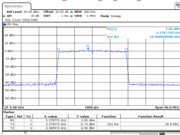
802.11be20_5580MHz_RU_FULL_Ant 0
