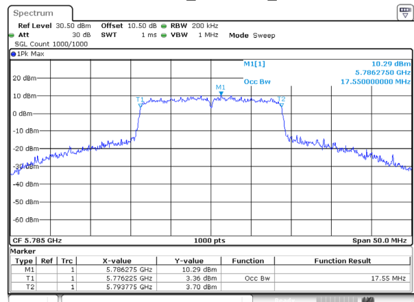
802.11ac20_5785MHz_Ant 0
