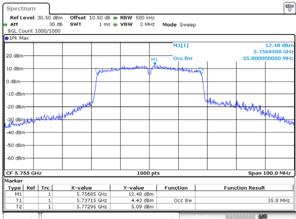
802.11ac40_5755MHz_Ant 1
