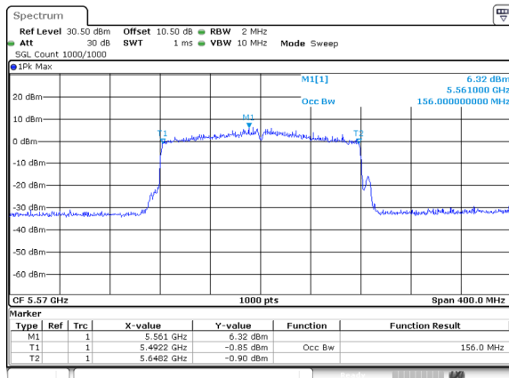
802.11be160_5570MHz_RU_FULL_Ant 2
