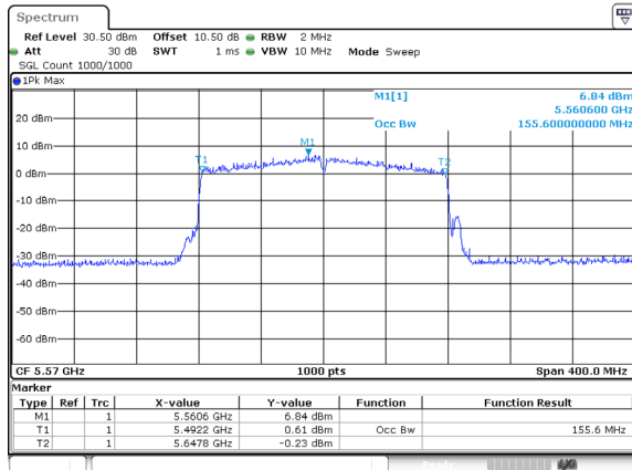
802.11be160_5570MHz_RU_FULL_Ant 0
