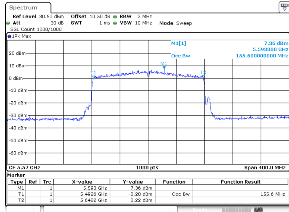
802.11be160_5570MHz_RU_FULL_Ant 1
