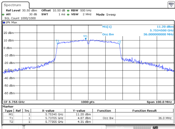
802.11ac40_5755MHz_Ant 0
