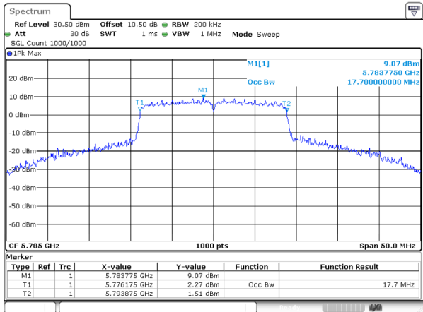
802.11ac20_5785MHz_Ant 2
