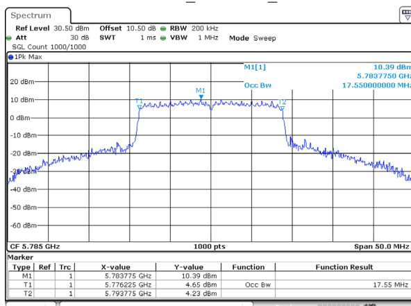
802.11ac20_5785MHz_Ant 1
