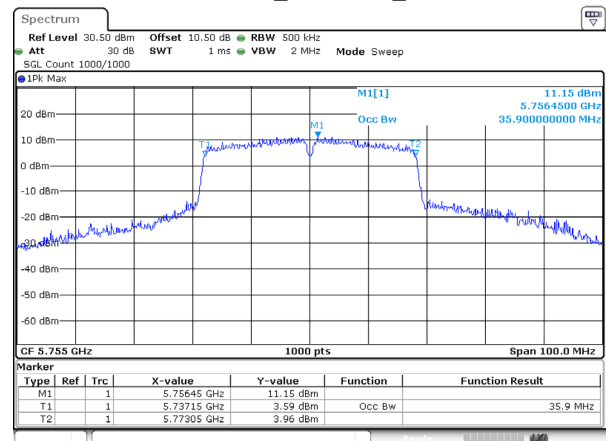
802.11ac40_5755MHz_Ant 2
